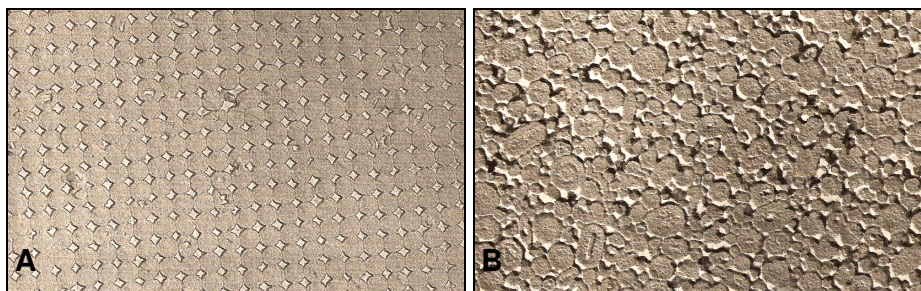
Figura 12. Micrografia eletrônica. (A) opala preciosa demonstrando o agrupamento regular das partículas de sílica e (B) opala comum com arranjo irregular das esferas.
