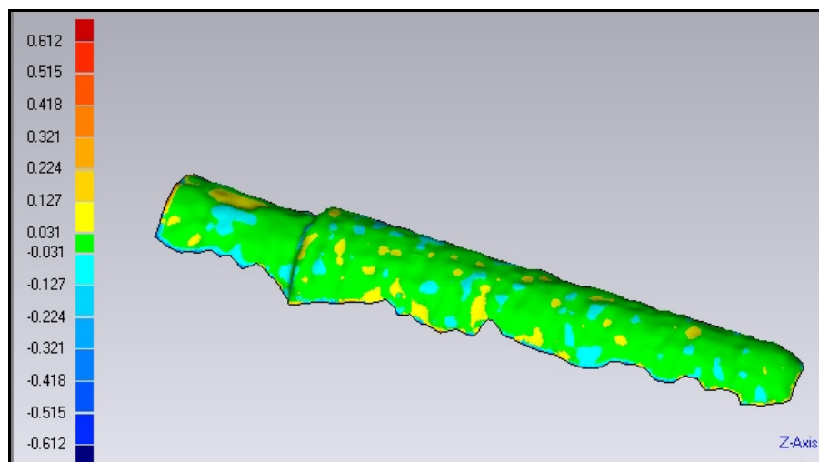
Figura 53. Fresa PMG_720 e a ausência dos tons avermelhados, que indicam a diferença de medidas.
