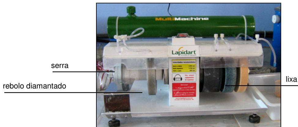
Figura 24. Equipamento de corte, formação e polimento de materiais gemológicos, pertencente ao LdSM – UFGRS
