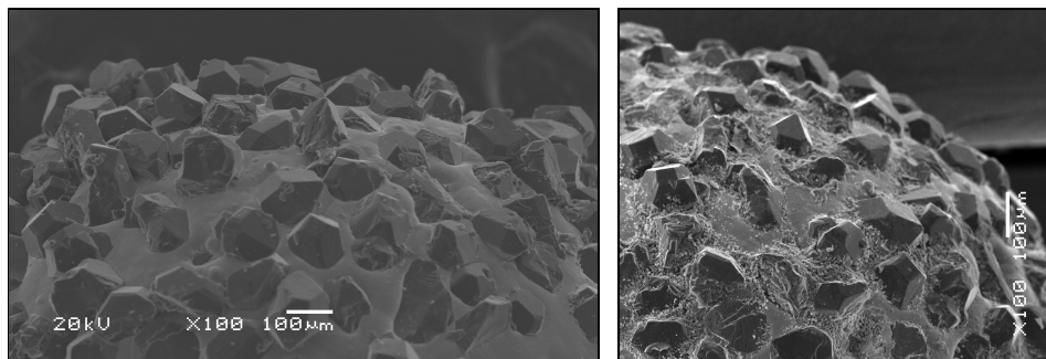
Figura 49. Em (A), fresa PMG_720 antes da usinagem e em (B) após a usinagem, não demonstrando desgaste visível.
