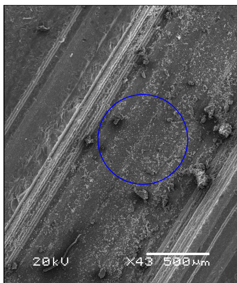
Figura 45. Marcas da fresa de ponta cônica, PMG_710_2, na superfície de opala branca.
