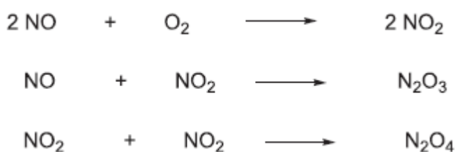
Esquema 3.8: Reações de NO na fase gasosa
