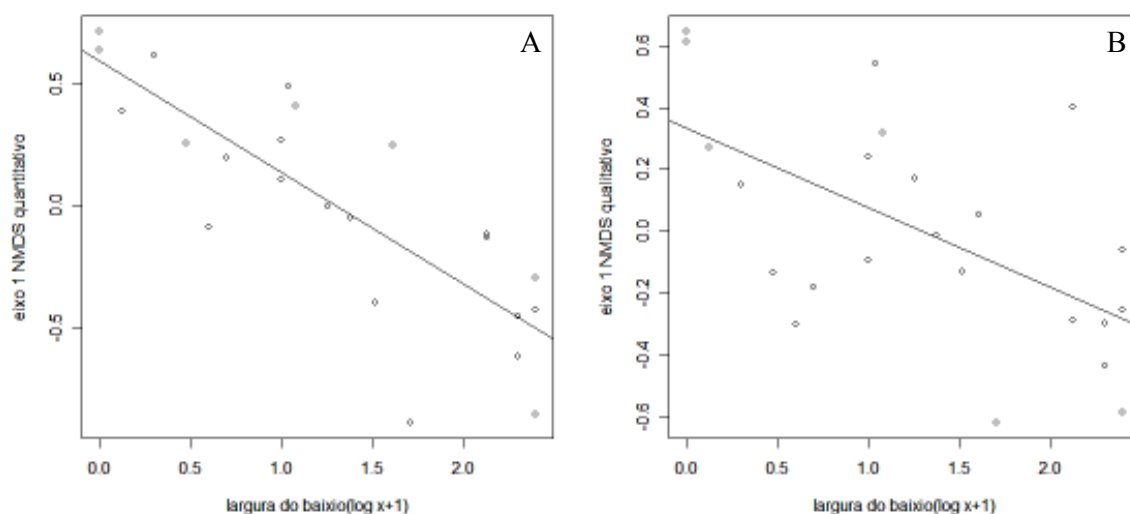
FIGURA 13. — Relação entre a largura do baixio (log x+1) e a composição das espécies nas comunidades ripárias sumarizada em uma dimensão de uma ordenação NMDS (eixo 1 NMDS). (A) composição baseada nos dados de abundância (quantitativos) e (B) composição baseada nos dados de presença/ausência (qualitativos).
