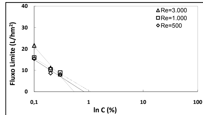
Figura 5.28: Fluxo limite em função do logaritmo da concentração da bentonita. Influência do regime de escoamento para densidade de empacotamento de 1.500 m 2 /m 3 . Módulo híbrido.
