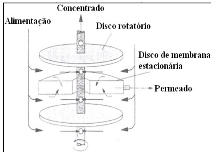
Figura 2.17: Módulo rotatório em placas planas. Adaptado de CHERYAN, 1998.
