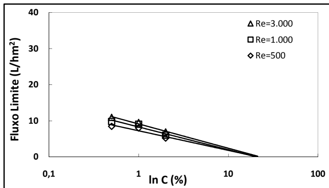
Figura 5.27: Fluxo limite em função do ln da concentração da levedura. Influência do regime de escoamento e da densidade de empacotamento de 1.500 m 2 /m 3 . Módulo híbrido.
