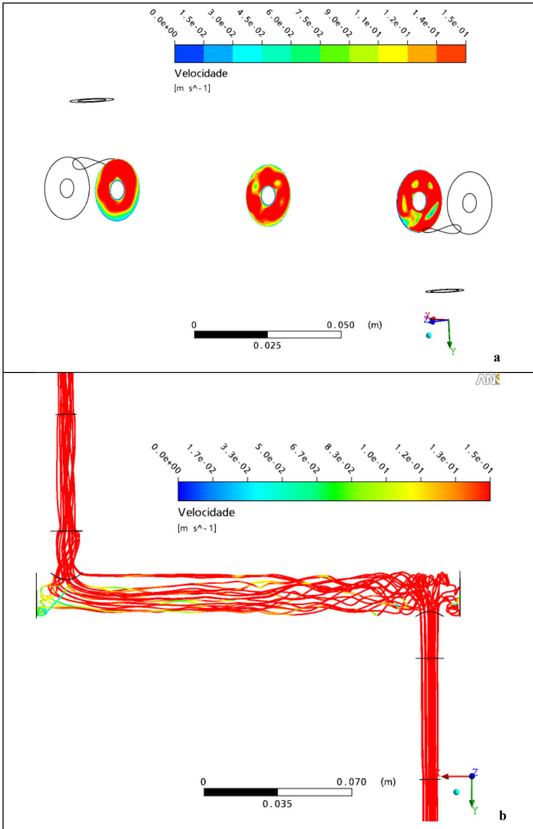
Figura 4.13: Perfil de velocidade para malha ML2. BSL e Reynolds igual a 3.000. (a) perfil de velocidade para três seções transversais ao escoamento e (b) perfil de velocidade representado por linhas de corrente.
