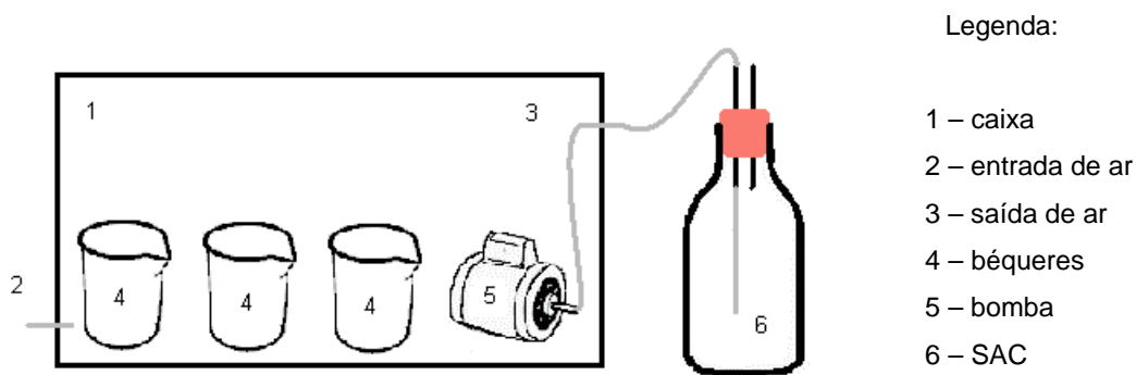
Figura 1. Esquema do sistema de secagem de urina usado no experimento.
