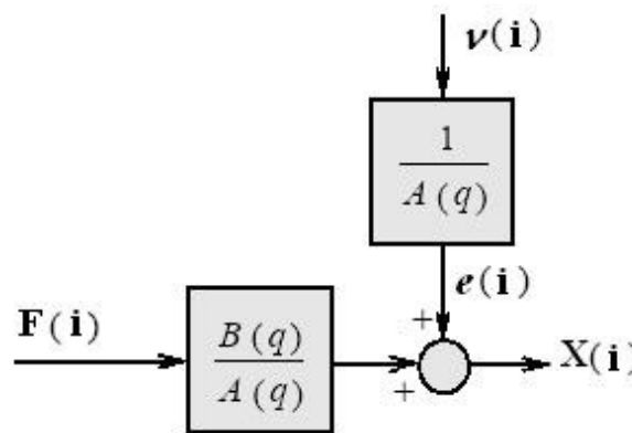
Figura 4.7: Representação esquemática do modelo ARX.
