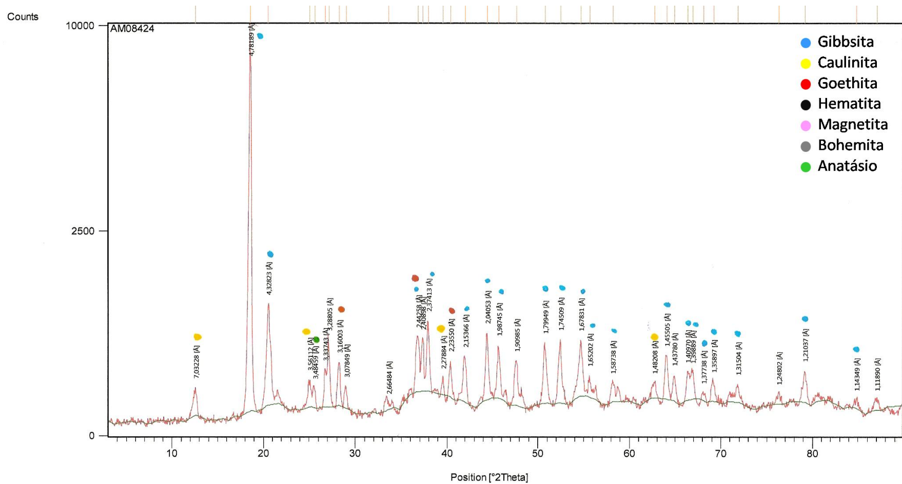
Difratograma amostra Bauxita Nodular (-0,840+0,212mm – Produto Não Magnético)
