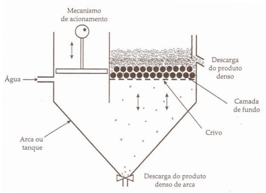
Figura 3.12: Esquema de separação em um jig (Sampaio e Tavares, 2005)
