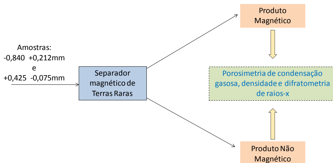
Figura 4.8: Esquema da separação magnética
