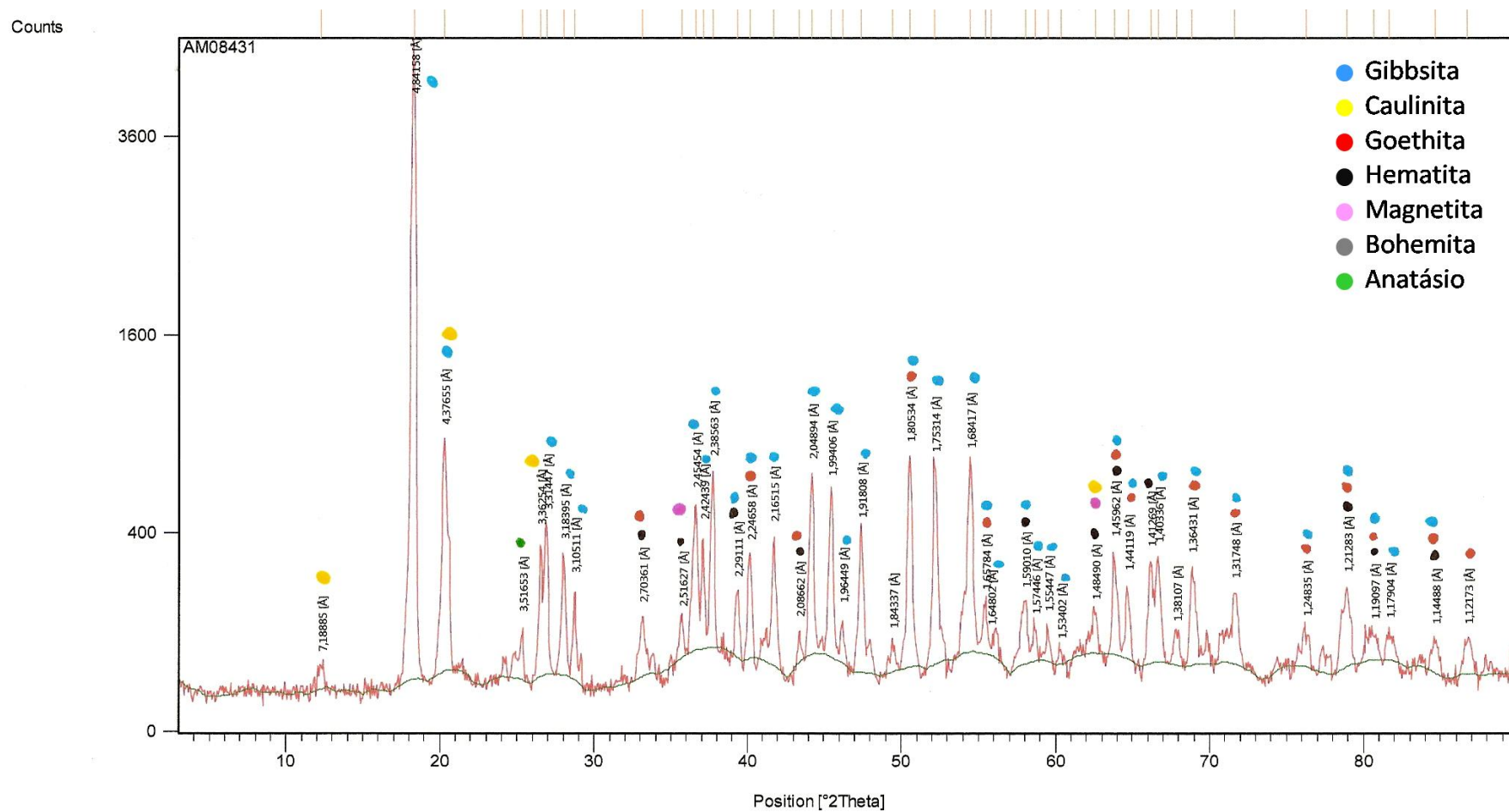
Difratograma amostra Bauxita Maciça in Natura (-0,840 + 0,212mm – Produto Não Magnético)
