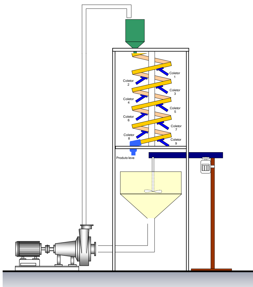
Figura 4.3: Esquema da montagem utilizada na realização dos testes de concentração.
