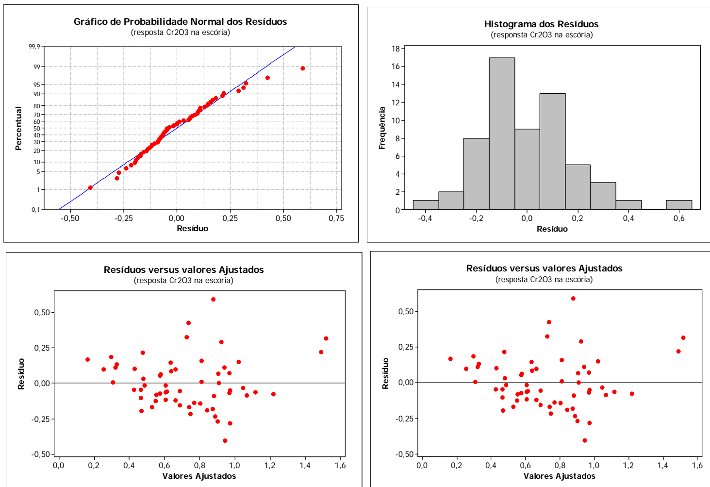
Figura 5.23 – Gráficos de resíduos para o \text{Cr}_2\text{O}_3 .
