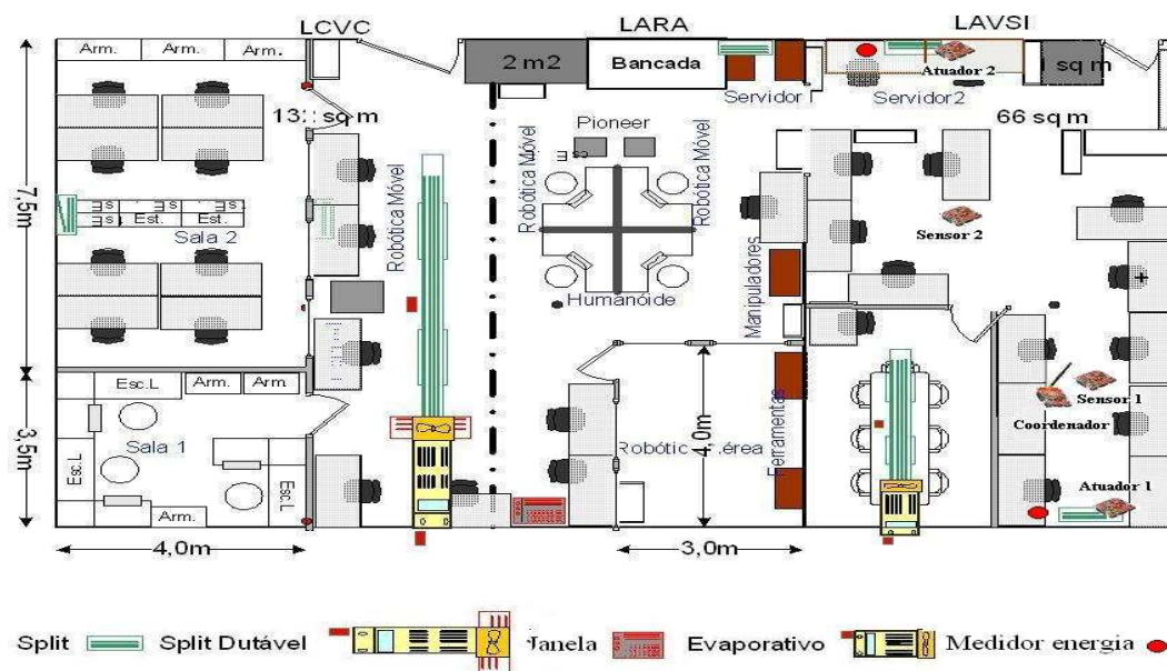
Figura 4.1 - Sistema térmico.
