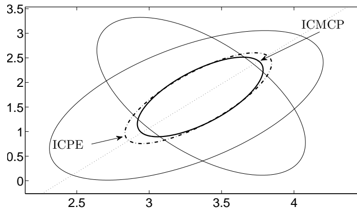
Figura 3.2: Fusão de dados em um sistema com restrição entre os estados e correlação desconhecida utilizando método da intersecção de covariâncias com minimização da covariância projetada (ICMCP) e método da intersecção de covariâncias com projeção da estimativa (ICPE)
