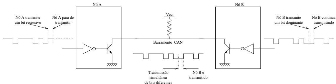
Figura 26: Característica da dominância em um barramento.
