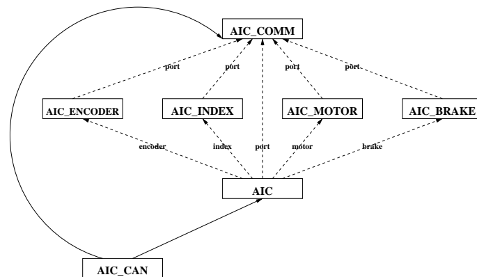
Figura 32: Hierarquia de classes da biblioteca AIC.
