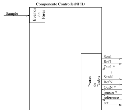
Figura 17: Modelo de componente ControllerNPID .
