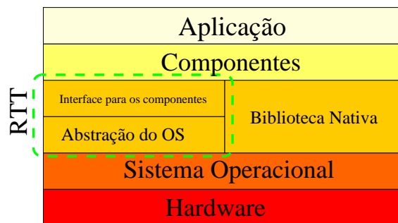
Figura 2: Camadas de uma aplicação utilizando o OROCOS.
