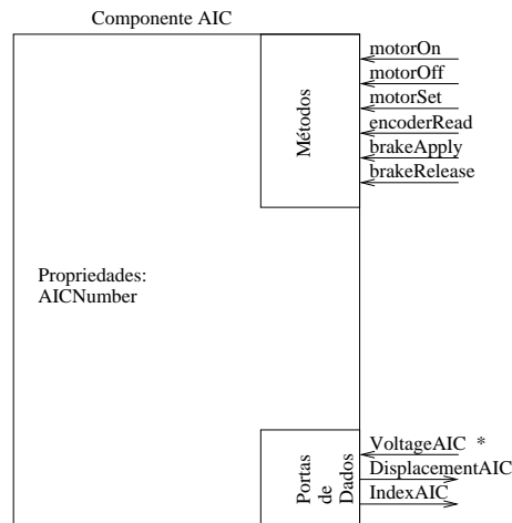
Figura 34: Modelo de componente AIC.
