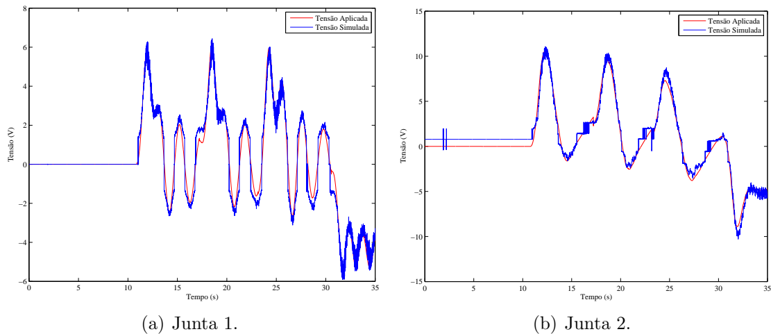
Figura 49: Tensão.
