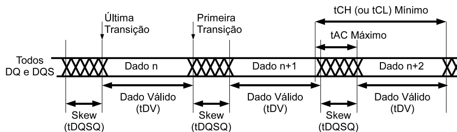
Figura 3.7: Janela de dado válido e variação entre os sinais DQ e DQS gerados pela memória DDR.
