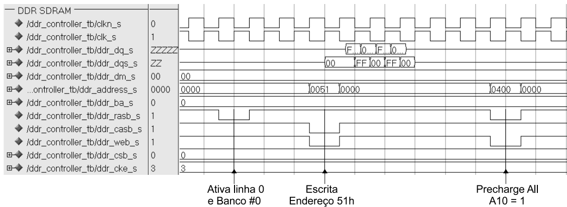
Figura 5.8: Forma de onda de simulação de uma escrita na memória.
