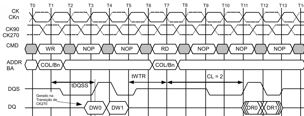
Figura 3.3: Diagrama de tempo de escrita e leitura na memória DDR.
