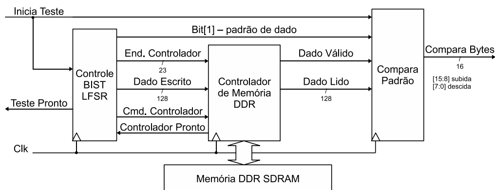
Figura 5.5: Diagrama de blocos do BIST.
