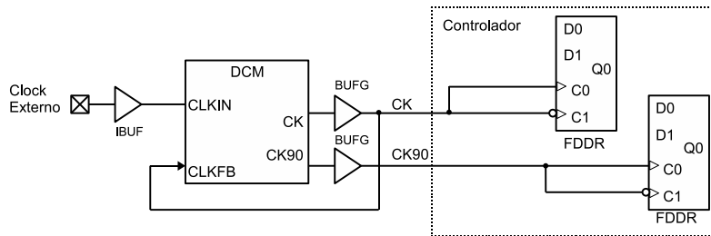
Figura 3.4: Diagrama de blocos da distribuição de relógios com inversão local.
