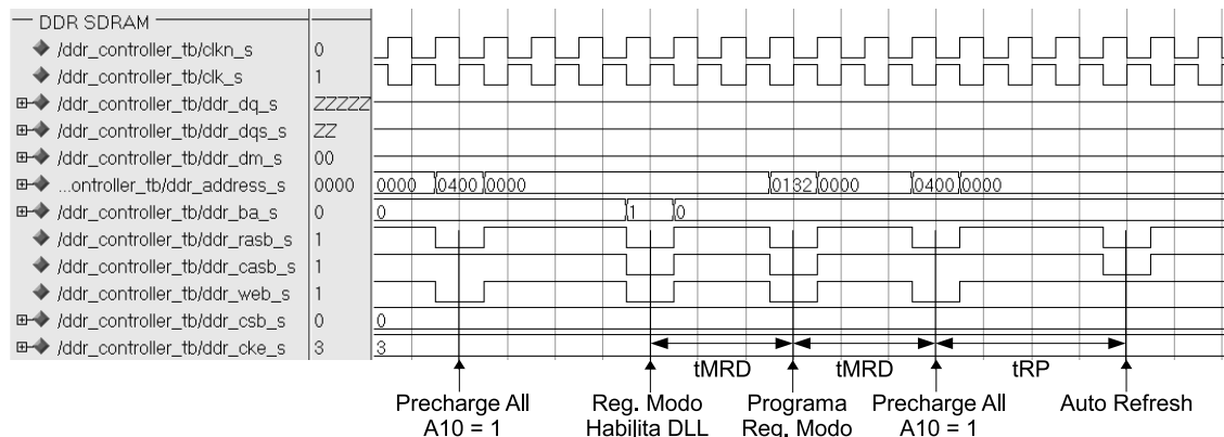
Figura 5.6: Forma de onda de simulação da etapa de inicialização da memória.
