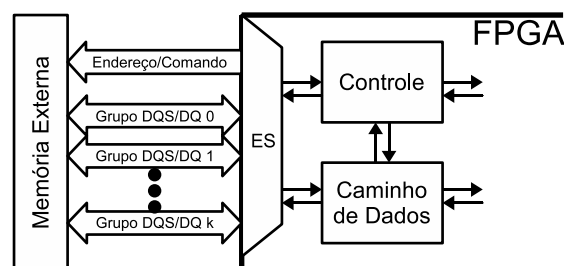
Figura 3.15: Interface de ES do controlador mapeada para a fronteira do FPGA mais próxima com a memória externa.
