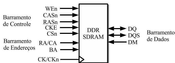
Figura 2.5: Diagrama de sinais da interface de memória DDR SDRAM.
