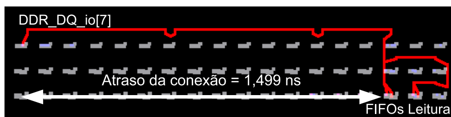
Figura 4.8: Captura do FPGA Editor , atraso entre pino de ES e registradores.
