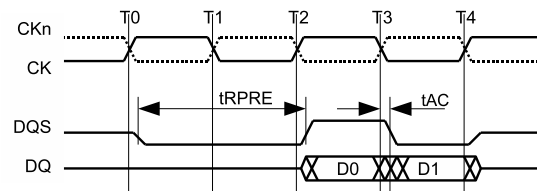
Figura 3.2: Diagrama de tempo de leitura, dado DQ e amostrador DQS são entregues ao controlador alinhados.
