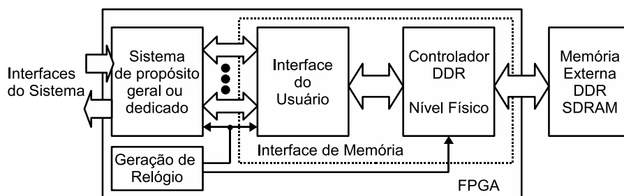
Figura 3.16: Diagrama de blocos simplificado da interface de memória.
