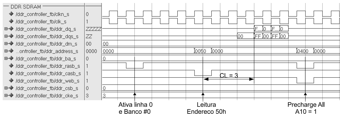
Figura 5.7: Forma de onda de simulação de uma leitura da memória.
