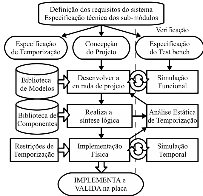
Figura 4.1: Fluxo de projeto de um núcleo firm para FPGA.
