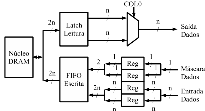
Figura 2.7: Arquitetura 2n -prefetch: circuito de sincronização de dados da memória.
