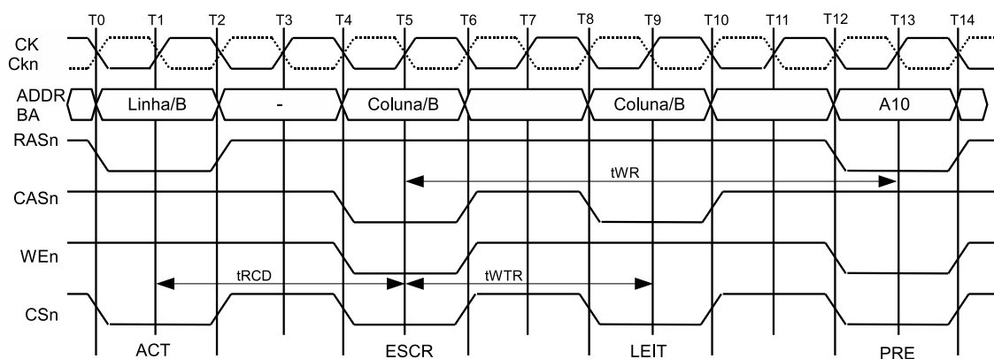
Figura 4.3: Diagrama de tempo dos sinais de controle e endereço.
