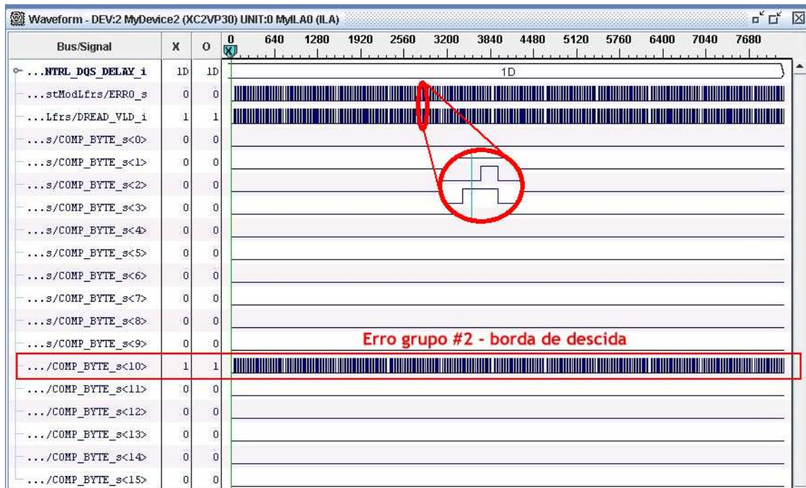
Figura 5.12: Verificação do controlador com defeito de implementação.
