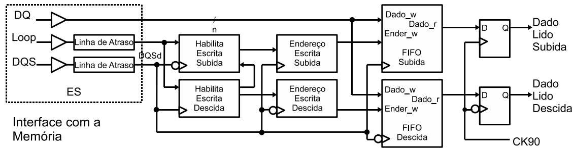
Figura 4.5: Caminho de leitura de dados na memória.
