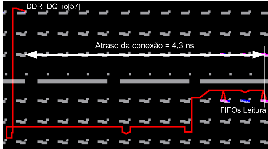
Figura 4.7: Captura do FPGA Editor , atraso entre pino de ES e registradores.
