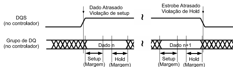
Figura 5.10: Violações de setup e hold na interface de dados.
