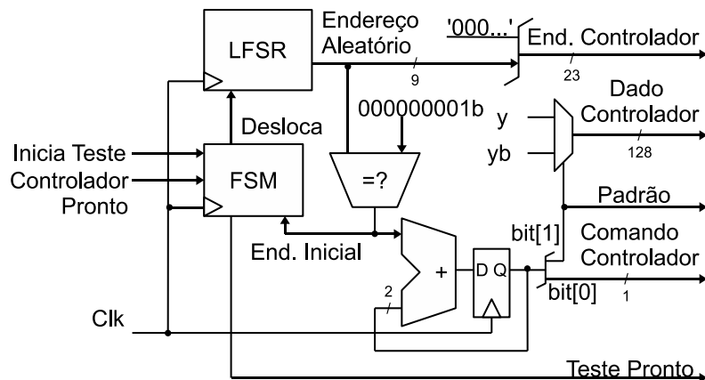
Figura 5.4: Diagrama de blocos da parte de controle do BIST.
