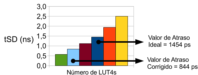
Figura 5.13: Gráfico comparativo entre o número de LUT4s e o atraso.
