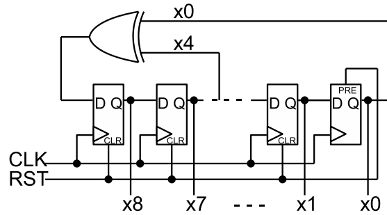
Figura 5.2: Gerador de padrão LFSR.
