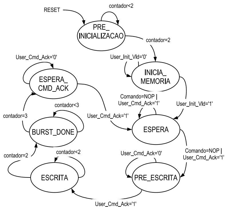
Figura 3.24: Diagrama de estados da máquina de escrita.
