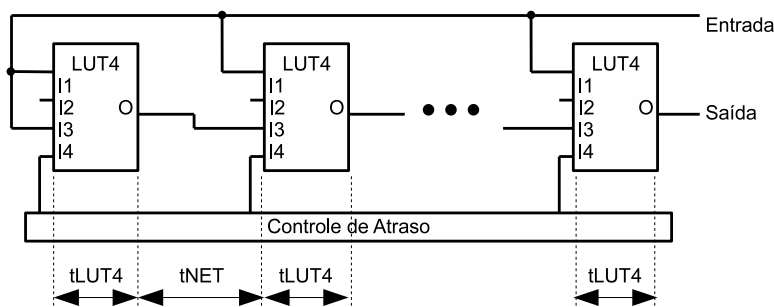
Figura 3.13: Circuito de geração de atraso programável para implementação em FPGA.
