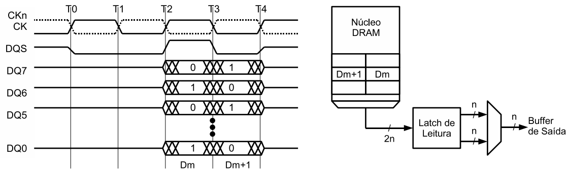
Figura 5.1: Padrão de dados usado no teste do controlador e diagrama de blocos da arquitetura interna da memória DDR SDRAM.
