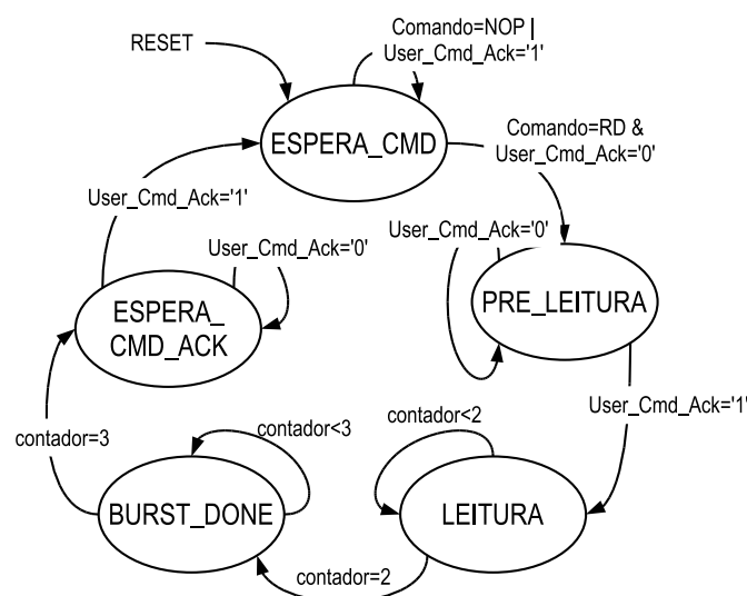
Figura 3.22: Diagrama de estados da máquina de leitura.
