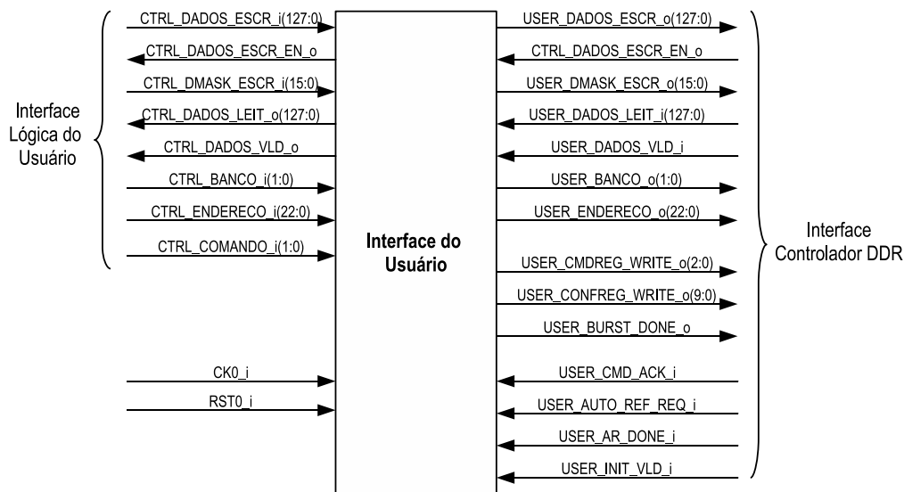
Figura 3.21: Sinais da interface com o usuário.
