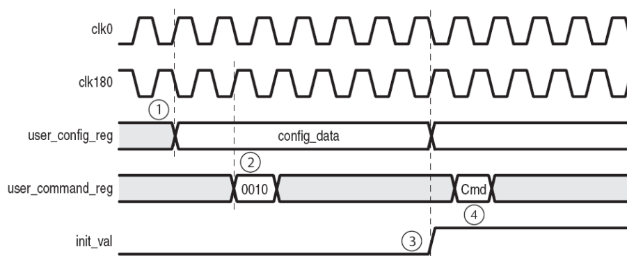
Figura 3.17: Diagrama temporal de inicialização da memória na entrada do controlador DDR. Fonte: (XILINX, 2005).
