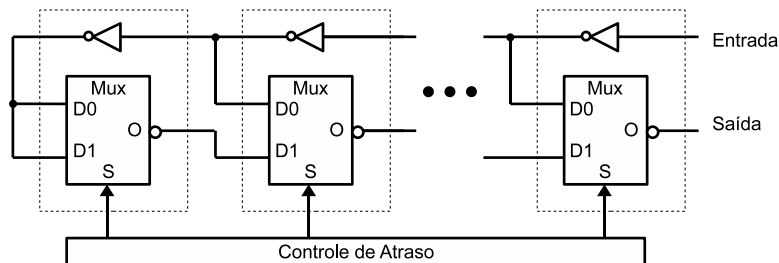
Figura 3.12: Circuito de geração de atraso com elementos programáveis.
