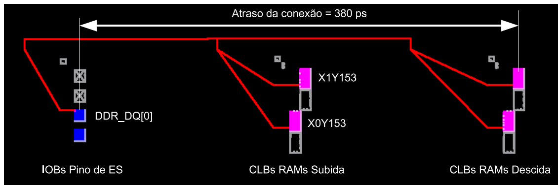
Figura 3.26: Registradores de captura com mapeamento forçado próximos ao pino de ES.
