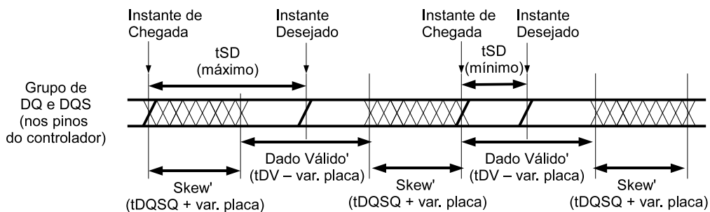
Figura 3.9: Intervalos mínimo e máximo de t_{SD} para atraso do amostrador DQS.
