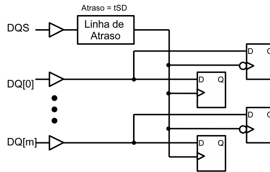
Figura 3.11: Circuito de captura de dados do controlador com amostrador atrasado.
