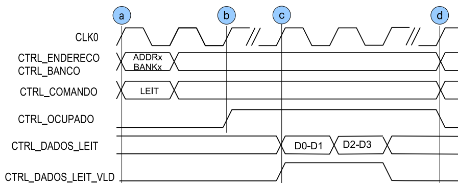
Figura 3.23: Diagrama de tempo da leitura de dados da interface do usuário.
