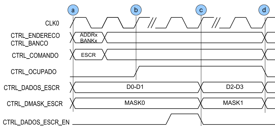
Figura 3.25: Diagrama de tempo da escrita de dados da interface do usuário.
