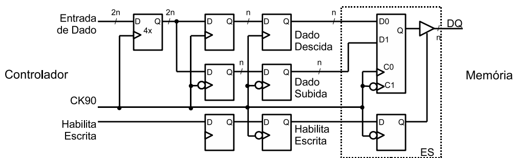
Figura 4.4: Caminho de escrita de dados na memória.
