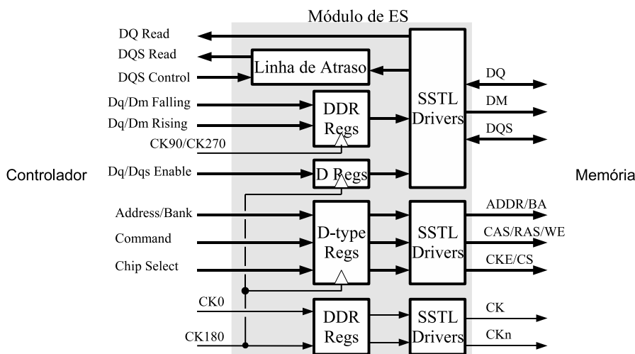
Figura 4.6: Diagrama de blocos do módulo de ES.
