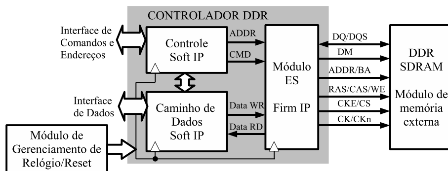
Figura 4.2: Diagrama de blocos da arquitetura do IP do controlador de memória DDR.
