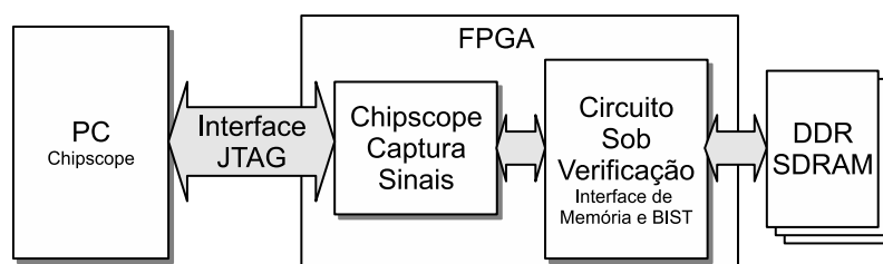
Figura 5.11: Diagrama de blocos do circuito de captura de sinais utilizando ChipScope.
