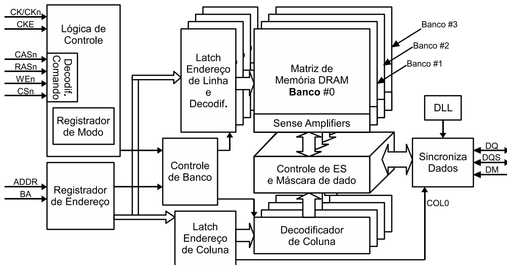
Figura 2.6: Diagrama de blocos simplificado da arquitetura interna da memória DDR SDRAM.
