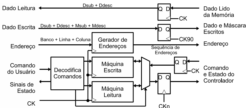
Figura 3.20: Diagrama de blocos simplificado da interface do usuário com o controlador DDR.
