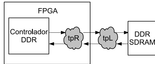
Figura 3.6: Tempos de propagação nas conexões entre memória e controlador.
