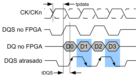
Figura 3.5: Diagrama de tempo da leitura dos dados com DQS atrasado.
