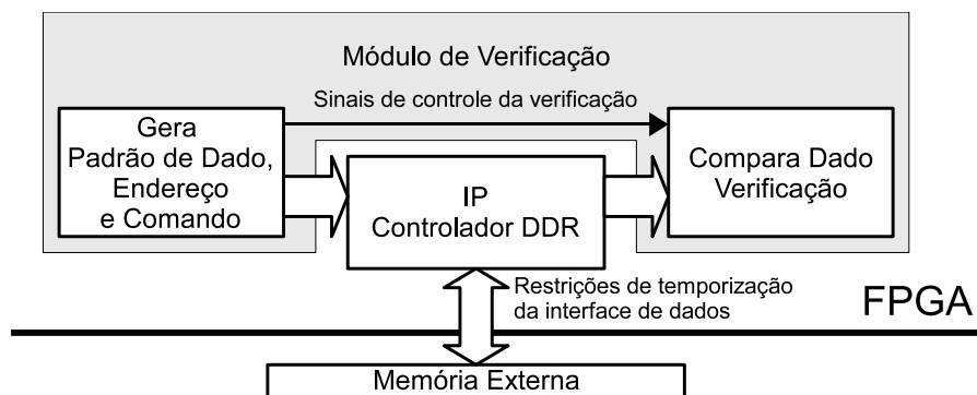
Figura 5.3: Diagrama de blocos do módulo de verificação do controlador.
