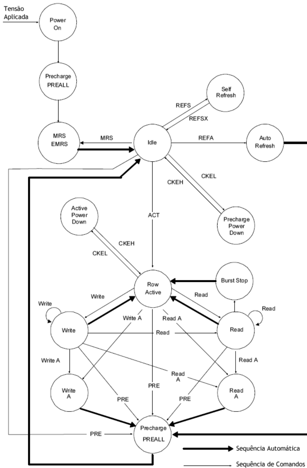
Figura 2.9: Diagrama de estados da máquina de controle de uma memória DDR SDRAM. Fonte: (JEDEC, 2003).
