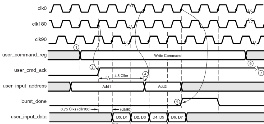
Figura 3.18: Diagrama temporal da interface com o controlador durante o processo de escrita. Fonte: (XILINX, 2005).
