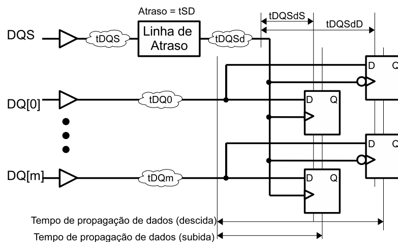
Figura 3.14: Diagrama de blocos simplificado do circuito de captura de dados e a representação dos tempos de propagação dos sinais pela matriz do FPGA.
