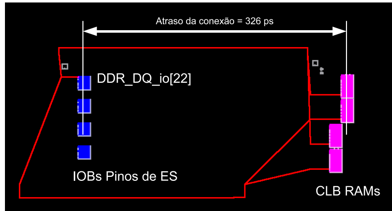
Figura 4.9: Captura FPGA Editor , exemplo de menor atraso entre dado e registrador.
