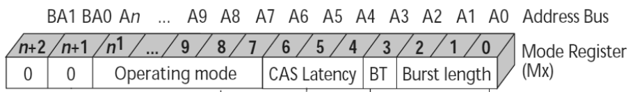
Figura 2.8: Registrador de Modo da DDR SDRAM. Fonte (JEDEC, 2003).
