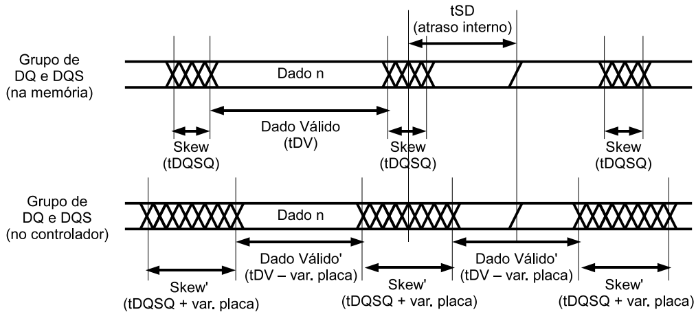
Figura 3.8: Redução da janela de dado válido pelas variações da placa.
