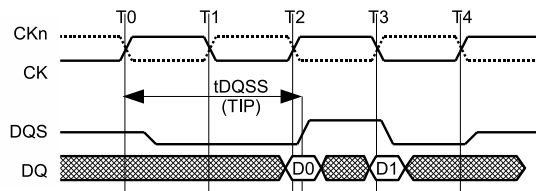
Figura 3.1: Diagrama de tempo de escrita, dado DQ e amostrador DQS são entregues à memória defasados de 90°.
