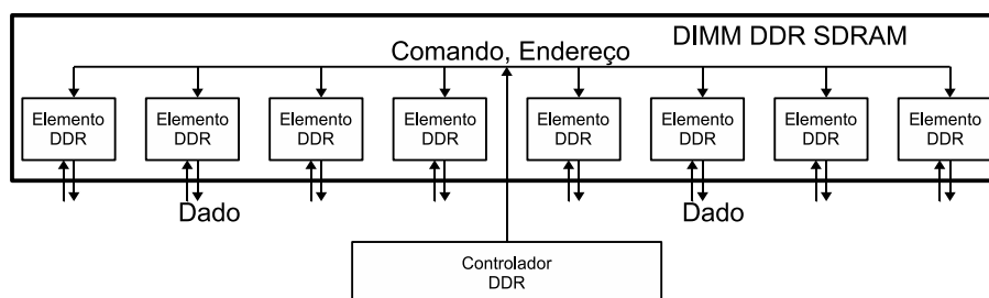
Figura 2.3: Diagrama de blocos simplificado de um módulo DIMM DDR SDRAM.
