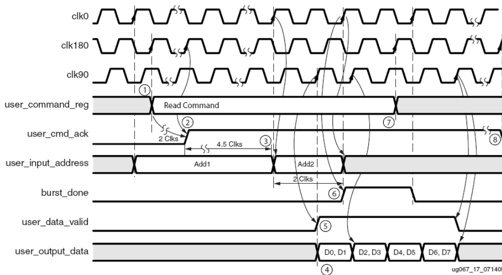
Figura 3.19: Diagrama temporal da interface com o controlador durante o processo de leitura. Fonte: (XILINX, 2005).
