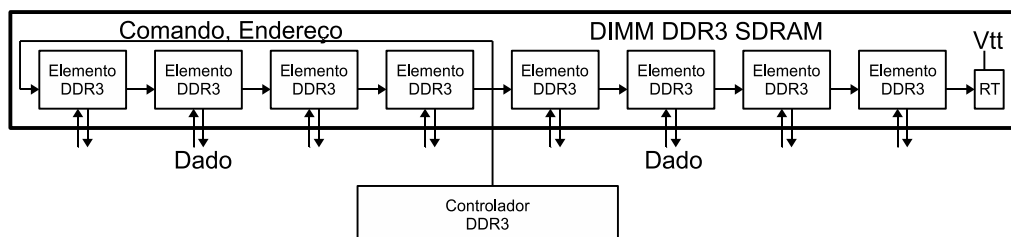
Figura 2.2: Diagrama de blocos simplificado de um pente DIMM DDR3 SDRAM.
