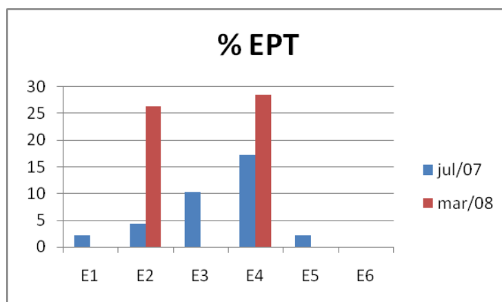
Figura 21: Porcentagem de Ephemeroptera, Plecoptera e Trichoptera (%EPT) ao longo das estações amostrais nas épocas de estiagem (jul/07) e chuva (março/2008).
