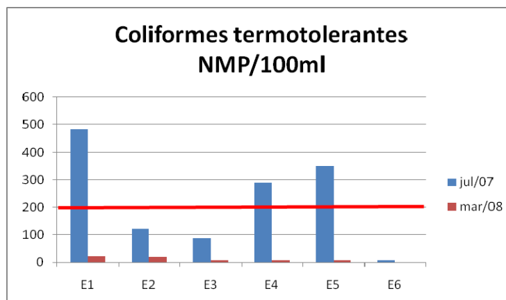
Figura 15: Concentração de coliformes fecais (NMP/100ml) na água ao longo das estações amostrais nas épocas de estiagem (julho/2007) e chuva (março/2008).
