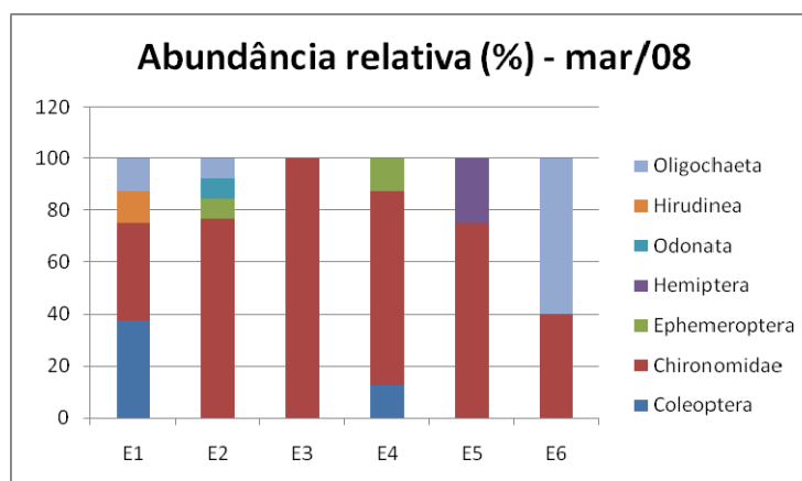
Figura 19: Abundância relativa (%) dos principais grupos taxonômicos coletados ao longo das estações amostrais na época de chuva (março/2008).
