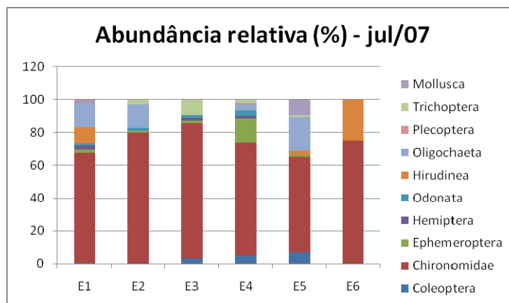
Figura 18: Abundância relativa (%) dos principais grupos taxonômicos coletados ao longo das estações amostrais na época de estiagem (julho/2007).
