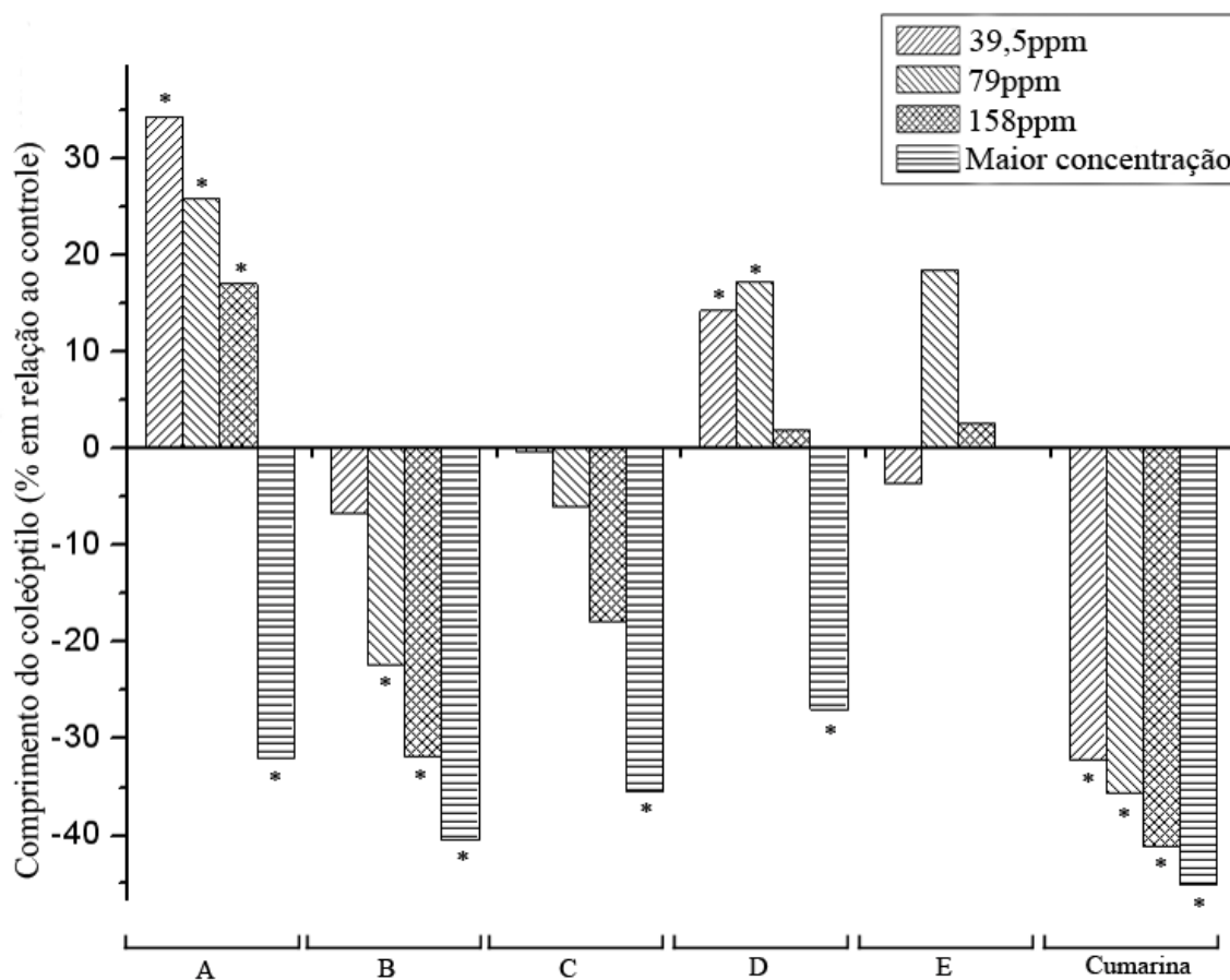
Figura 1. Valores percentuais médios do comprimento dos coleóptilos de trigo em relação ao controle (* - diferença significativa em relação ao controle).
