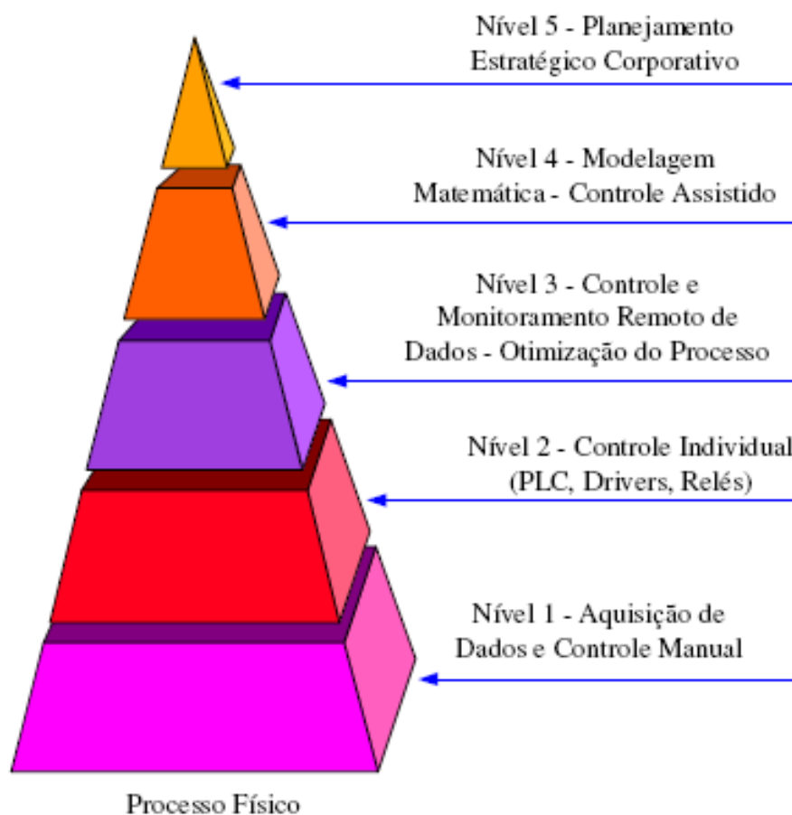
Figura 10 – Níveis de Controle Industrial – Pirâmide de Automação. Fonte: Webb, 1992 apud Pereira e Souza, 2008
