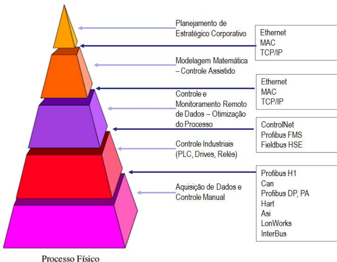
Figura 11 – Correspondência Pirâmide de Automação e Protocolos de Rede. Fonte: Moraes e Castrucci, 2007
