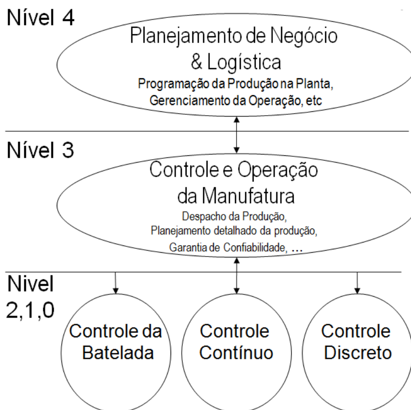
Figura 5 – Hierarquia Funcional. Fonte: Adaptado de ISA, 2000, p. 19
