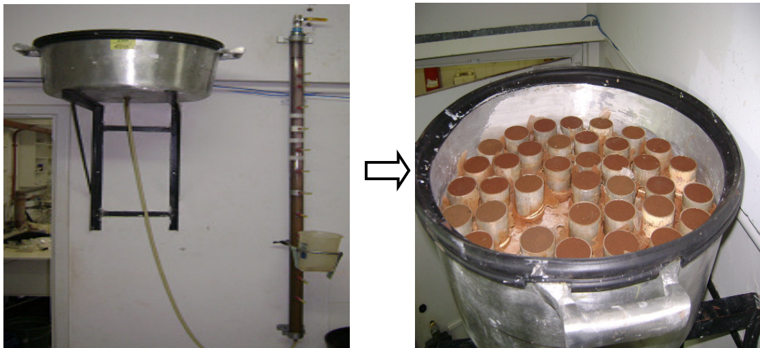
FIGURA 7. Panela de tensão a 60 cm da coluna d'água, utilizada para determinação de macroporosidade do solo. (Adaptado para o Laboratório de Manejo e Conservação do solo - UFU, 2008). Foto: Gomides, 2008
