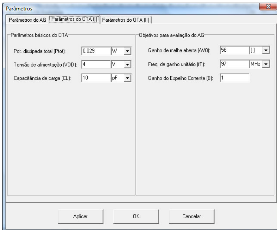
Figura 45 – Janela onde são determinados pelo projetista, V_{DD} , C_L e P_{tot} , além dos valores dos objetivos A_{V0\_obj} , f_{T\_obj} e B_{obj} .
