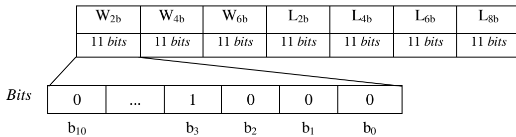
Figura 17 – Estrutura do cromossoma para o AG proposto no estudo do OTA.
