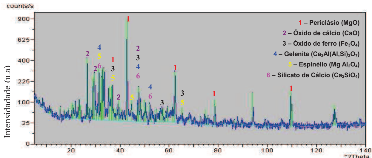
Figura 4.6 - Difratoograma da Escória D45.
