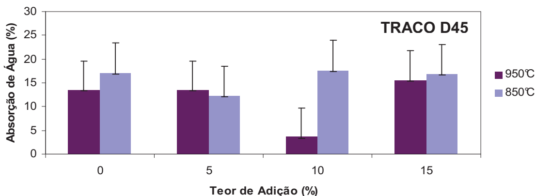
Figura 4.29 - Absorção de água dos corpos de prova D45.
