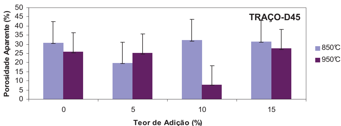
Figura 4.31 - Porosidade aparente do Traço-D45.
