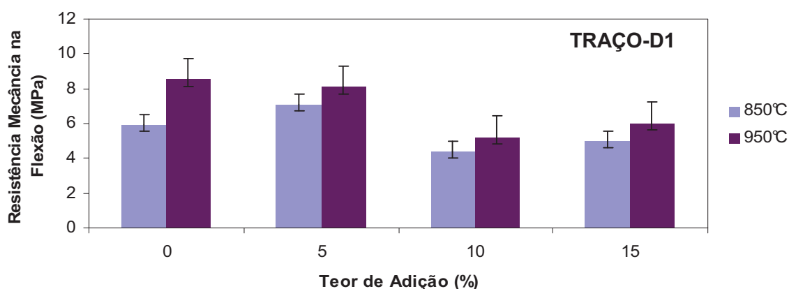
Figura 4.26 - Resistência mecânica na flexão dos corpos de prova D1.
