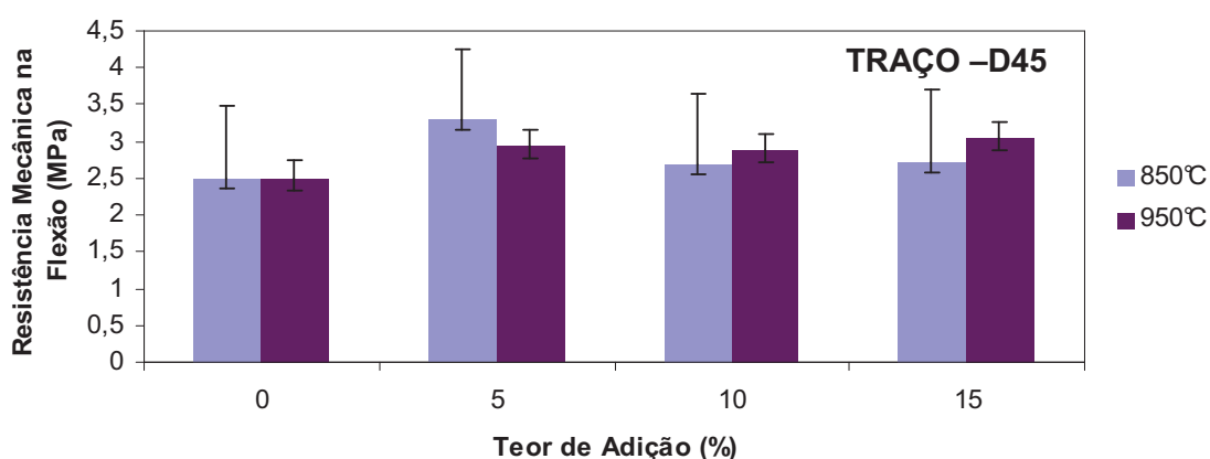
Figura 4.16 - Resistência mecânica dos corpos de prova D45.
