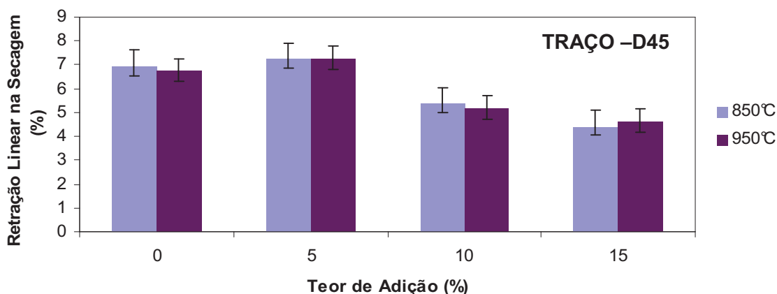
Figura 4.14- Retração linear dos corpos de prova D45.
