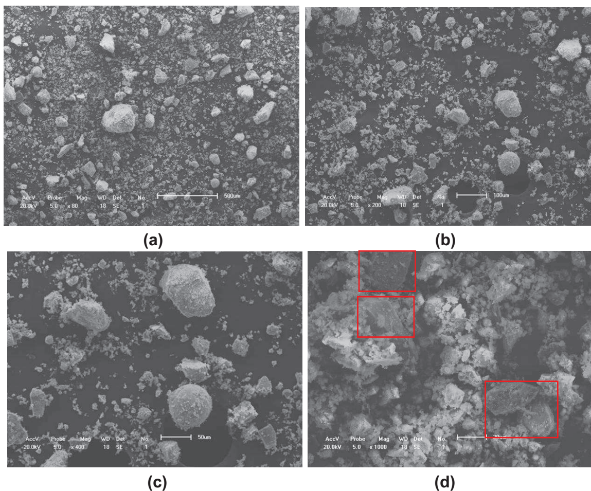
Figura 4.7 - Micrografia da Escória D1 - (a) 500 µm (b) 100 µm (c) 50 µm e (d) 20 µm. (b) Grão esférico (vermelho); (d) Grãos angulosos (vermelho).
