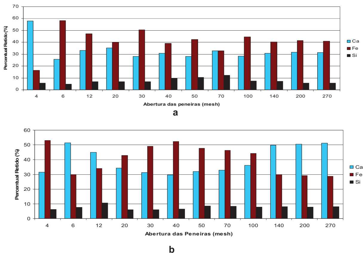
Figura 4.1 - Análise por fluorescência de raios-x dos elementos principais da escória: (a) Escória D1 e (b) Escória D45.
