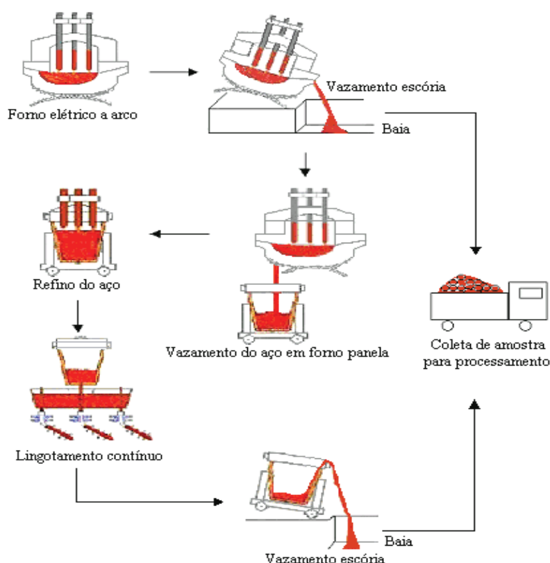
Figura 2.6 - Esquema do processo de formação e descarte da escória de aciaria elétrica na fabricação do aço (segundo Graffitti, 2002).
