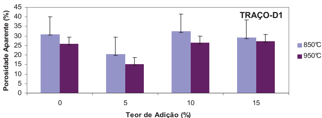
Figura 4.30 - Porosidade aparente do Traço-D1.
