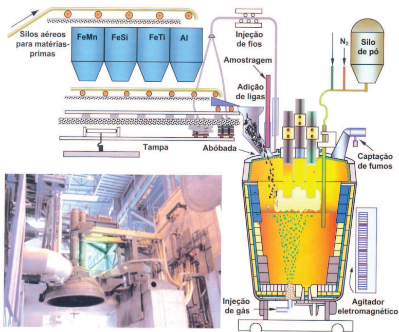
Figura 2.5 – Etapas do refino secundário forno-panela nas usinas siderúrgicas no Brasil (segundo Rizzo, 2006).
