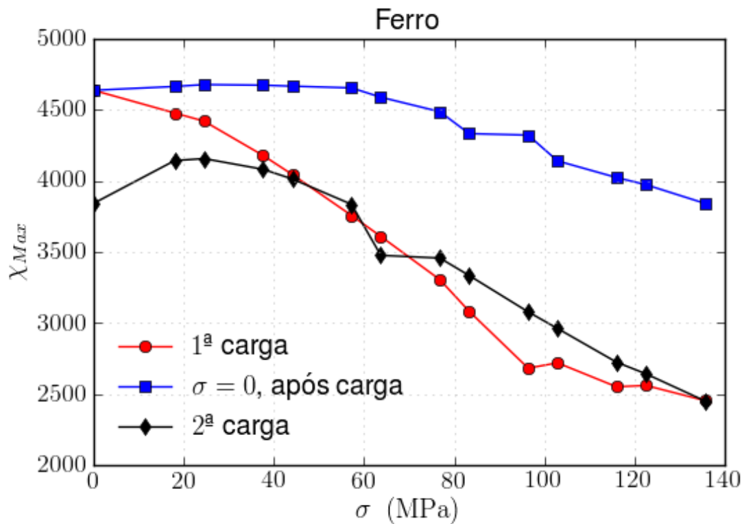
Figura 5.16: Susceptibilidade máxima diferencial em função da tensão aplicada sobre uma amostra de ferro.
