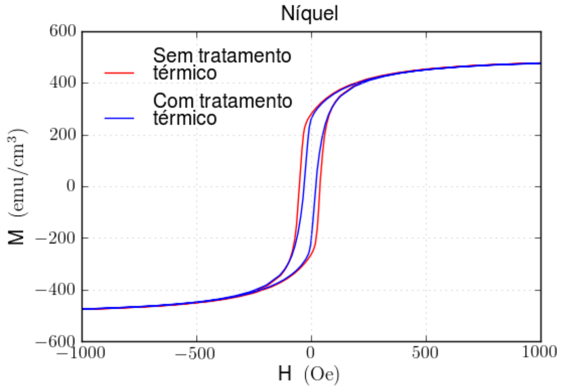
Figura 5.4: Curvas de magnetização M \times H para amostras de níquel com e sem tratamento térmico
