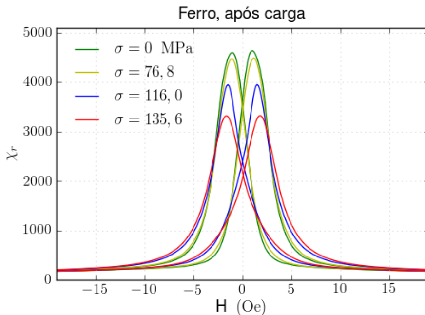
Figura 5.14: Curvas da susceptibilidade diferencial para amostras de ferro medidas após retirar a tensão \sigma aplicada. A curva para \sigma = 76,8 MPa apresenta uma pequena variação em relação à curva sem tensão, além dessa tensão a diminuição da susceptibilidade máxima é muito mais significativa.
