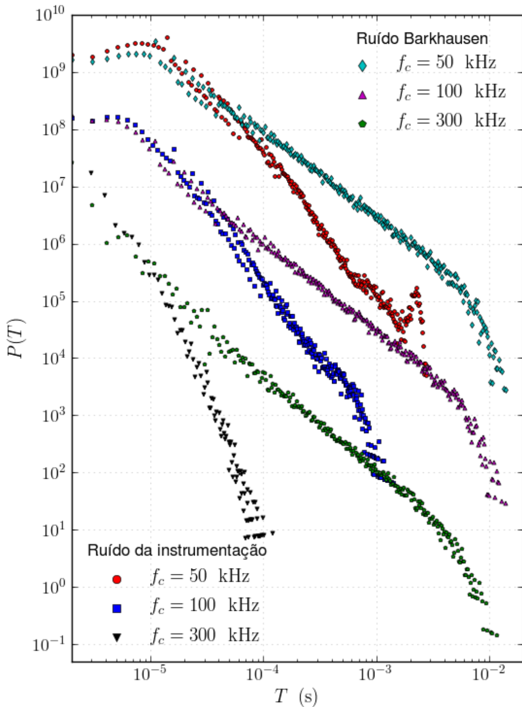
Figura 5.32: Distribuições de duração para uma amostra de ferro e para o ruído da instrumentação, calculadas das séries temporais medidas e filtradas com um filtro digital passa-baixa de frequência de corte f_c
