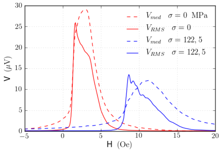
Figura 5.26: Curvas do RMS V_{RMS} e do valor medio V_{med} , obtidas para uma amostra de níquel após ter aplicado e retirado as tensões \sigma .
