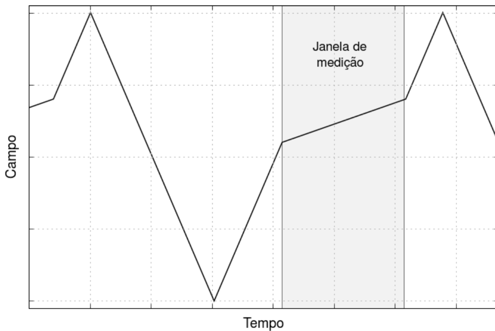
Figura 4.3: Sinal fornecido pelo gerador de funções, apresentando a janela com taxa de variação regulável onde é medido o ruído Barkhausen.
