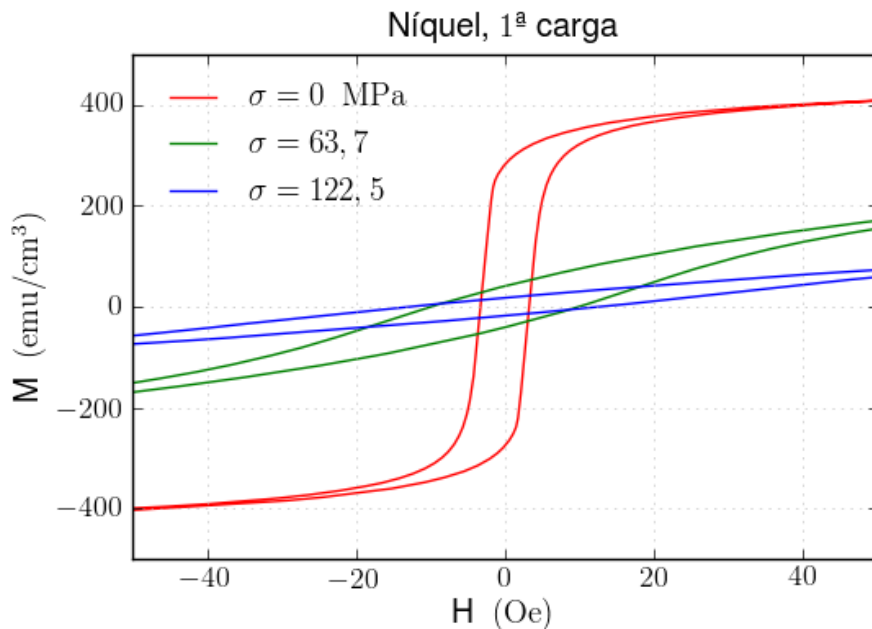
Figura 5.9: Curvas de magnetização para a amostra de níquel submetidas a diferentes tensões \sigma após do tratamento térmico. Pode-se observar a forte diminuição da magnetização com a tensão e o aumento do campo coercivo.
