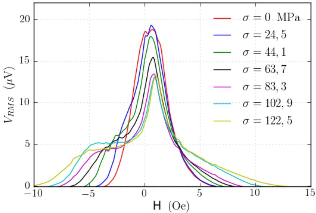
Figura 5.24: Curvas RMS obtidas para uma amostra de ferro sobre diferentes tensões \sigma , aplicadas após do tratamento térmico.
