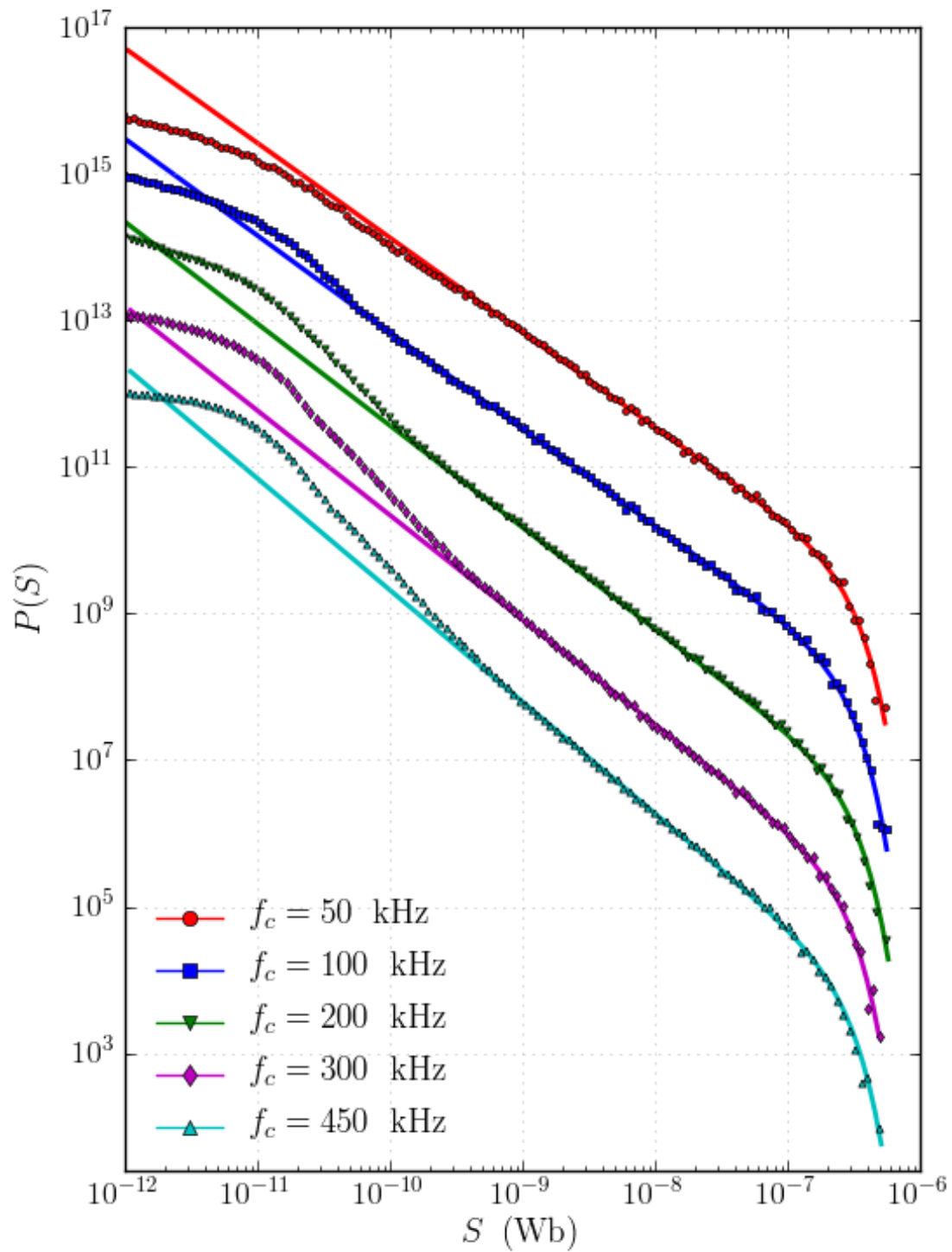
Figura 5.35: Distribuições de tamanho e ajustes respectivos para uma amostra de ferro, calculadas com diferentes filtros passa-baixa de frequência de corte f_c aplicados nas séries temporais.
