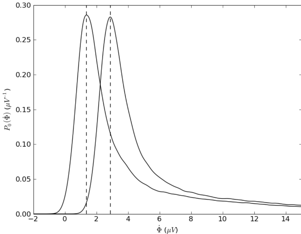
Figura 4.5: Histogramas suavizados de duas séries temporais após filtradas, e as modas calculadas para cada um deles (linhas verticais)
