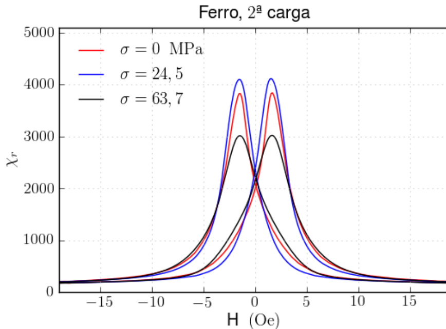
Figura 5.15: Curvas da susceptibilidade diferencial para amostras de ferro com diferentes tensões \sigma aplicadas, após ter sido aplicada uma tensão de 135 MPa. A curva para a tensão \sigma = 24,5 MPa apresenta uma maior susceptibilidade que a curva sem tensão (magnetostricção efetiva positiva), mas para a tensão \sigma = 63,7 MPa a susceptibilidade diminui novamente (magnetostricção efetiva negativa).
