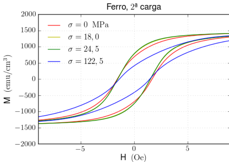
Figura 5.7: Curvas de magnetização para amostras de ferro com diferentes tensões \sigma aplicadas, após de ter aplicado uma tensão de 135,6 MPa. As curvas com tensões \sigma = 18 MPa e \sigma = 24,5 MPa apresentam maior magnetização que a curva sem tensão, mas ao aumentar a tensão até \sigma = 122,5 MPa a magnetização diminui significativamente.
