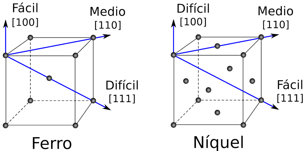
Figura 2.1: Direções preferenciais de magnetização para cristais de ferro e níquel
