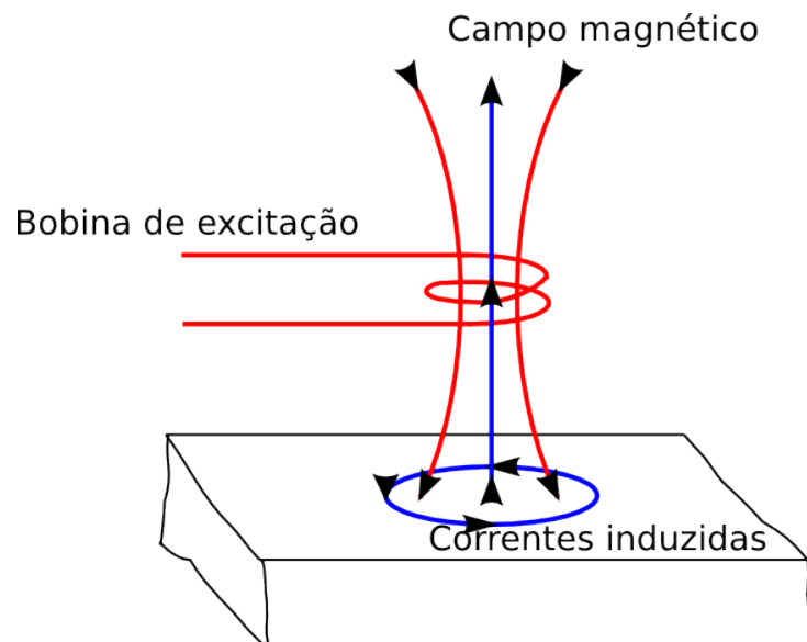
Figura 3.1: Esquema do ensaio de correntes parasitas.
