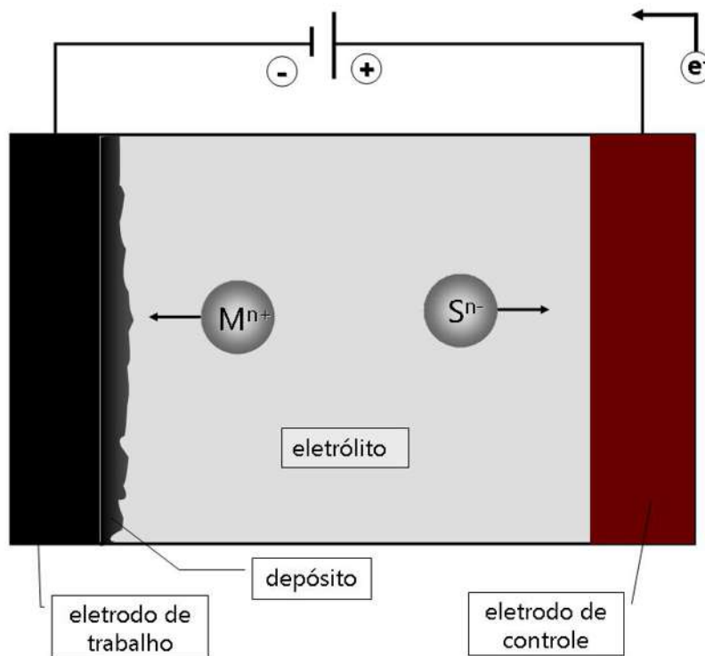
Figura 1.4: Esquema de uma célula usada para eletrodeposição. O sal que compõe o eletrólito é, usualmente, formado pelo metal representado pela letra M e um sulfato ou sulfeto representado pela letra S, diluído. Ao conectarmos os eletrodos à bateria, uma corrente é produzida no fluido, que faz com que este metal se solidifique no eletrodo de trabalho, formando o depósito.
