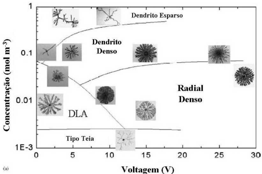
Figura 1.6: Diagrama de fase da eletrodeposição de Zn com relação à voltagem aplicada sobre os eletrodos e a concentração da solução. (Retirada de [22].)
