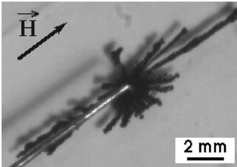
Figura 2.14: Depósito de Cobalto com B_{\parallel} = 0,2 \text{ T} , C = 0,1 M , V = 5 \text{ V} . Cedida pelo autor, retirada de [27].
