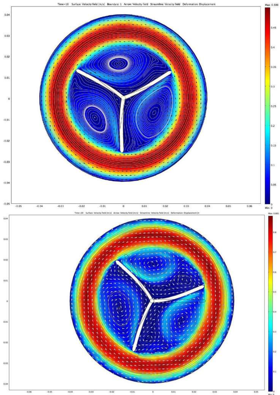
Figura 4.39: Perfil das velocidades do fluido (segundo a escala à direita) no interior da célula, usando os parâmetros: v = 1 \text{ V} , \sigma = 1 \text{ S/m} , \sigma_b = 10^7 \text{ S/m} , \nu = 10^{-2} \text{ Pa s} , e campo magnético externo: (a) B = 5 \text{ T} , Re = 2,0 , (b) B = 10 \text{ T} , Re = 3,5 .
