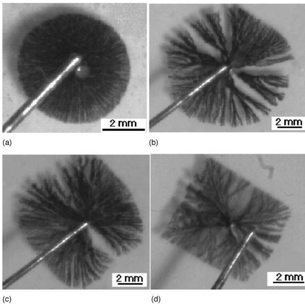
Figura 2.11: Deposição de Ferro com (a) B = 0 (b) B_{\parallel} = 0,04 T (c) B_{\parallel} = 0,14 T (d) B_{\parallel} = 0,23 T, mantendo todos os outros parâmetros da experiência idênticos. C = 0,06 M, V = 5 V. Cedida pelo autor, retirada de [27].
