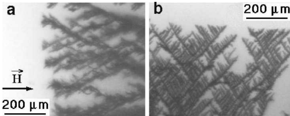
Figura 2.12: Detalhe dos braços do depósito de Ferro da figura 2.11(d) observado pelo microscópio, perpendicular (a) e paralelamente (b) à direção do campo. B_{\parallel} = 0,23 \text{ T} , C = 0,06 \text{ M} , V = 5 \text{ V} . Cedidas pelo autor, retiradas de [27]
