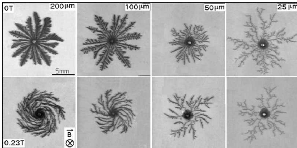
Figura 2.9: Depósitos de Zn (sal de \text{ZnSO}_4 , C = 0,06 \text{ M} , V = 10 \text{ V} ) crescidos livre e sob ação de campo magnético de magnitude B_{\perp} = 0,23 \text{ T} , em função da espessura da célula usada. Cedida pelos autores [25].
