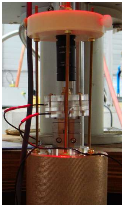
Figura 2.4: Fotografia do aparato experimental. A célula e a câmera prestes a entrar na bobina supercondutora que produzirá o campo magnético.
