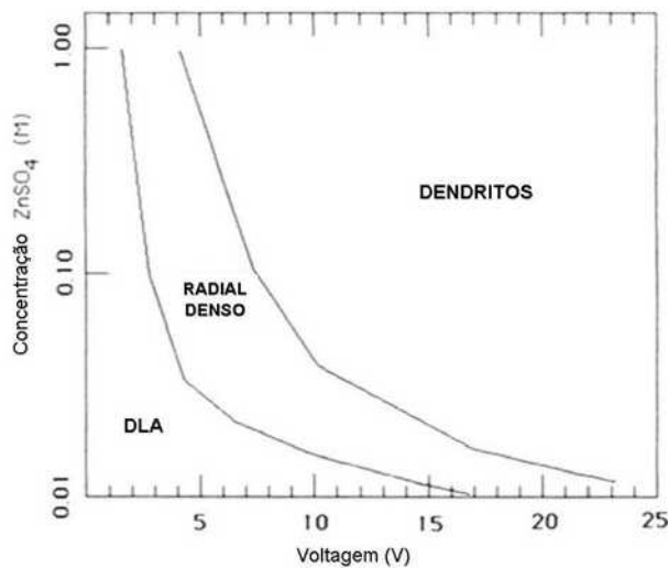
Figura 1.5: Diagrama de fase da eletrodeposição de Zn com relação à voltagem aplicada sobre os eletrodos e a concentração da solução. (Retirada de [21].)
