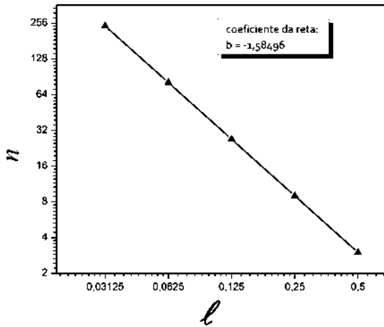
Figura 3.7: Cálculo da dimensão fractal usando os valores encontrados na Figura 3.6(b).
