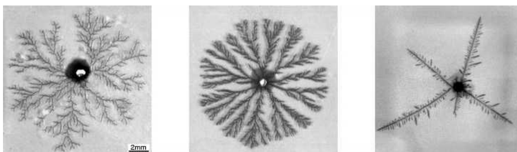
Figura 2.5: Depósitos de Zinco. (a) Tipo DLA C = 0,01 \text{ M} , V = 2,6 \text{ V} , espessura da célula t = 50 \mu\text{m} , (b) Morfologia densa radial (DBM): C = 0,01 \text{ M} , V = 4 \text{ V} , espessura da célula t = 200 \mu\text{m} , (c) Morfologia esparsa: C = 0,3 \text{ M} , V = 10 \text{ V} , espessura da célula t = 100 \mu\text{m} . Cedida pelos autores [25].
