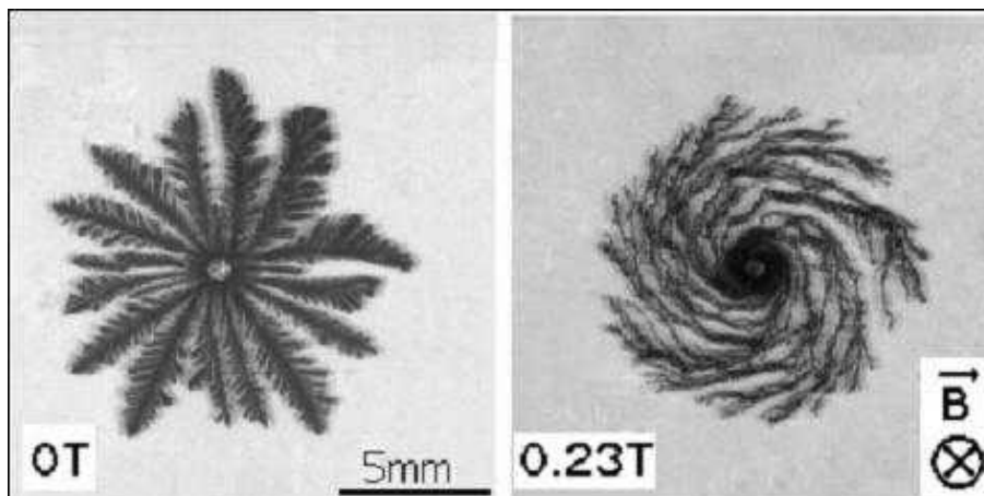
Figura 2.6: Comparação entre depósitos de zinco (sal de ZnSO_4 ), crescidos sob mesmas condições ( C = 0,06 M , V = 10 V ) sem campo magnético (figura à esquerda) e com campo magnético B_{\perp} = 0,23 T (à direita). Cedida pelos autores [25].
