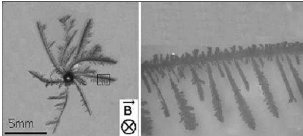
Figura 2.8: A figura à direita mostra o detalhe de um dos braços da estrutura de zinco à esquerda, crescido sob ação de campo magnético perpendicular B_{\perp} = 0,2 T ( C = 0,1 M, V = 10 V). Obtidas no Institute Néel, Grenoble, França (2007) [34].
