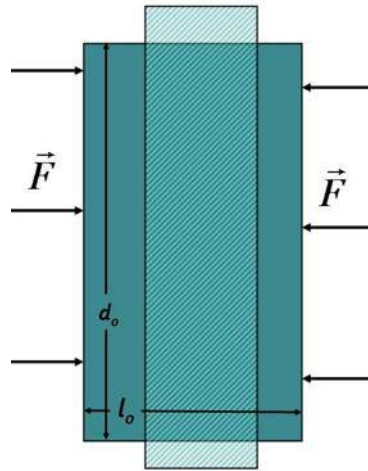
Figura 3.10: Esquema de deformação de um bloco sólido produzido por uma força de magnitude F .
