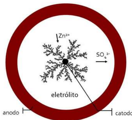
Figura 2.3: Vista superior da célula experimental, usando como exemplo a deposição de Zinco.
