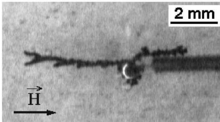
Figura 2.12: Detalhe dos braços do depósito de Ferro da figura 2.11(d) observado pelo microscópio, perpendicular (a) e paralelamente (b) à direção do campo. B_{\parallel} = 0,23 \text{ T} , C = 0,06 \text{ M} , V = 5 \text{ V} . Cedidas pelo autor, retiradas de [27]
