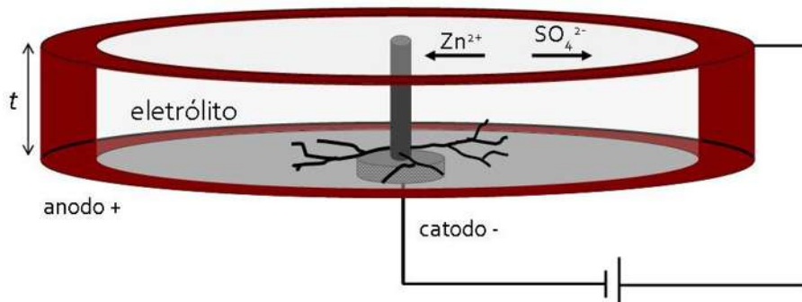
Figura 2.2: Esquema ilustrativo de uma célula circular usada em eletrodeposição. Como exemplo, foi usado um sal de sulfato de Zinco, ZnSO_4 .
