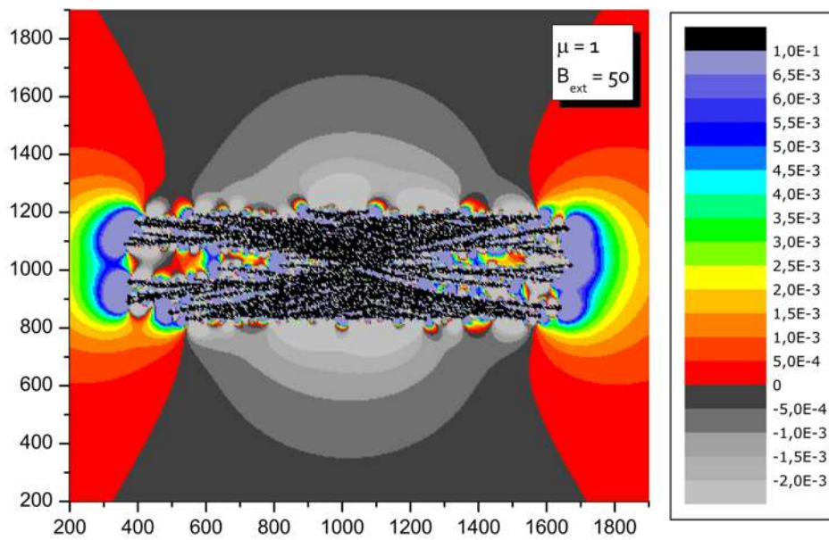
Figura 4.19: Resultados da simulação para baixos valores de momento magnético das partículas do agregado, K_{dd} = 5 . (c) Mapa do potencial magnético sentido por uma partícula de momento igual em módulo àquelas pertencentes ao agregado da fig. 4.17(b) ( B_x = 50 ). As cores dos gráficos representam faixas de valores dos potenciais, conforme escala à direita das figuras.
