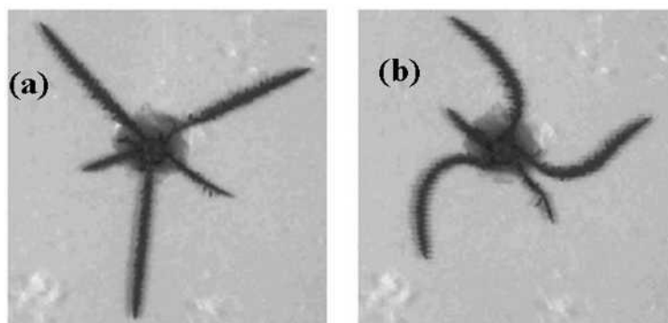
Figura 2.10: Resultado da deposição de Zn ( C = 0,3 \text{ M} , V = 10 \text{ V} ): (a) Inicialmente a estrutura cresce sem a ação de campo magnético, até um dado momento em que ele é ligado. (b) Após 0,24 segundos da aplicação do campo B = 0,23 \text{ T} , a forma original se torna uma espiral. Cedida pelos autores [25].
