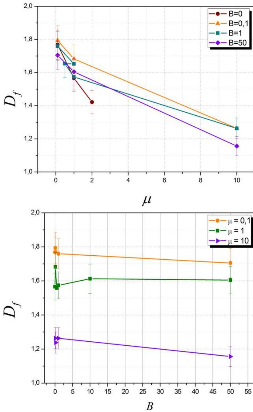
Figura 4.22: Comportamento da dimensão fractal dos agregados obtidos pela simulação: (a) Em função do momento magnético das partículas, para os seguintes valores de campo magnético B = 0 , B = 0,1 , B = 1 e B = 50 . (b) Em função do campo magnético aplicado, usando \mu = 0,1 , \mu = 1 e \mu = 10
