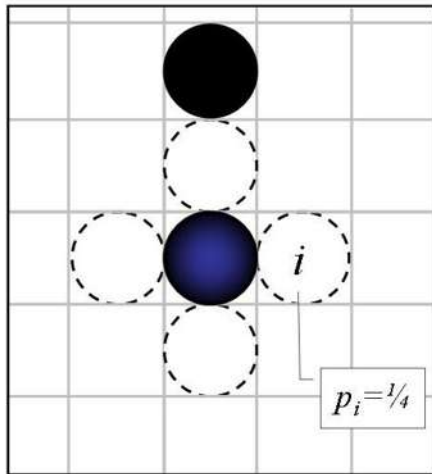
Figura 3.2: Esquema de caminhada para o algoritmo de DLA, numa rede quadrada, a partícula livre (círculo azul) pode se mover para qualquer uma das quatro novas posições com a mesma probabilidade.
