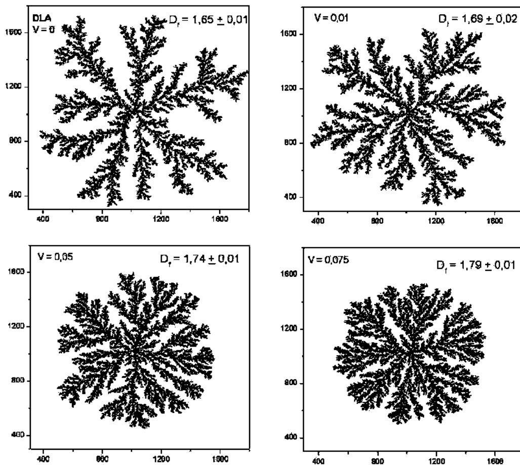
Figura 4.2: Variação da dimensão fractal em função do Potencial Elétrico. Todas as figuras são formadas por 100.000 partículas, 1/kT = 1 . (a) v = 0 (b) v = 0,01 (c) v = 0,05 (d) v = 0,075
