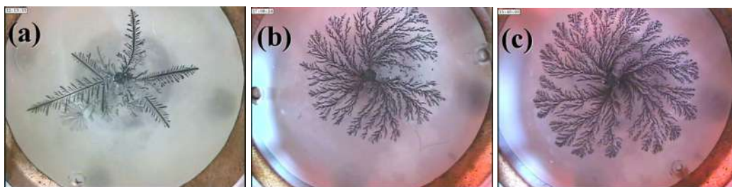
Figura 2.7: Depósitos de zinco (usando sal de \text{ZnSO}_4 e C = 0,1 \text{ M} , V = 10 \text{ V} , espessura da célula, t = 15 \mu\text{m} ) (a) Crescido sem aplicação de campo magnético (b) Sob ação de um campo magnético de B_{\perp} = 2 \text{ T} (c) e campo magnético de B_{\perp} = 4 \text{ T} . Obtidas no Institute Néel, Grenoble, França (2007).
