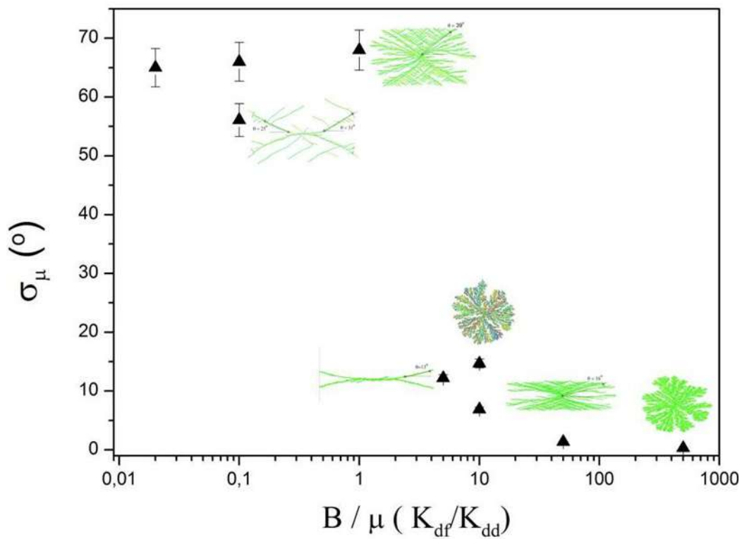
Figura 4.27: Relação entre \sigma e a razão K_{dd}/K_{df} , com o exemplo da forma das estruturas encontradas para alguns deles. \sigma indica o quão alinhados estão os momentos dipolares das partículas no agregado. Eles estão mais alinhados quanto menor for o valor de \sigma .
