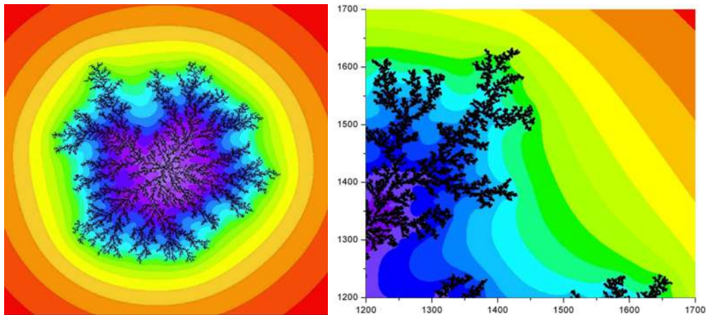
Figura 4.1: Mapa do campo elétrico próximo ao agregado, calculado usando v = 0,01 . Abaixo: detalhe do quadrante superior direito de (a).
