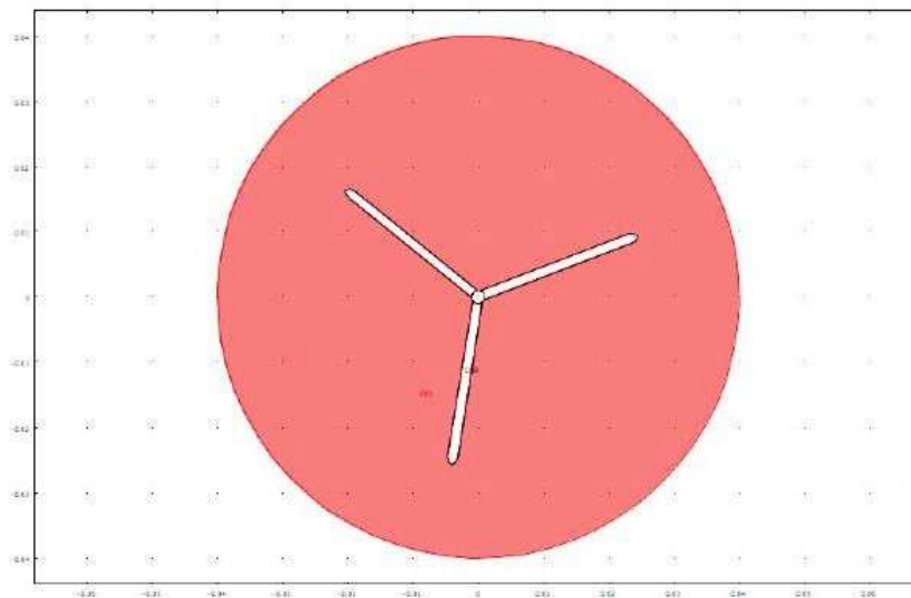
Figura 3.9: Geometria usada para produzir os resultados usando o Método de Elementos finitos. A região rosa representa o fluido, e a região branca é o domínio sólido que representa o agregado já crescido, preso ao catodo central. O círculo externo, de raio 4 cm representa o anodo, enquanto o catodo é representado pelo círculo interno de raio 2 mm.
