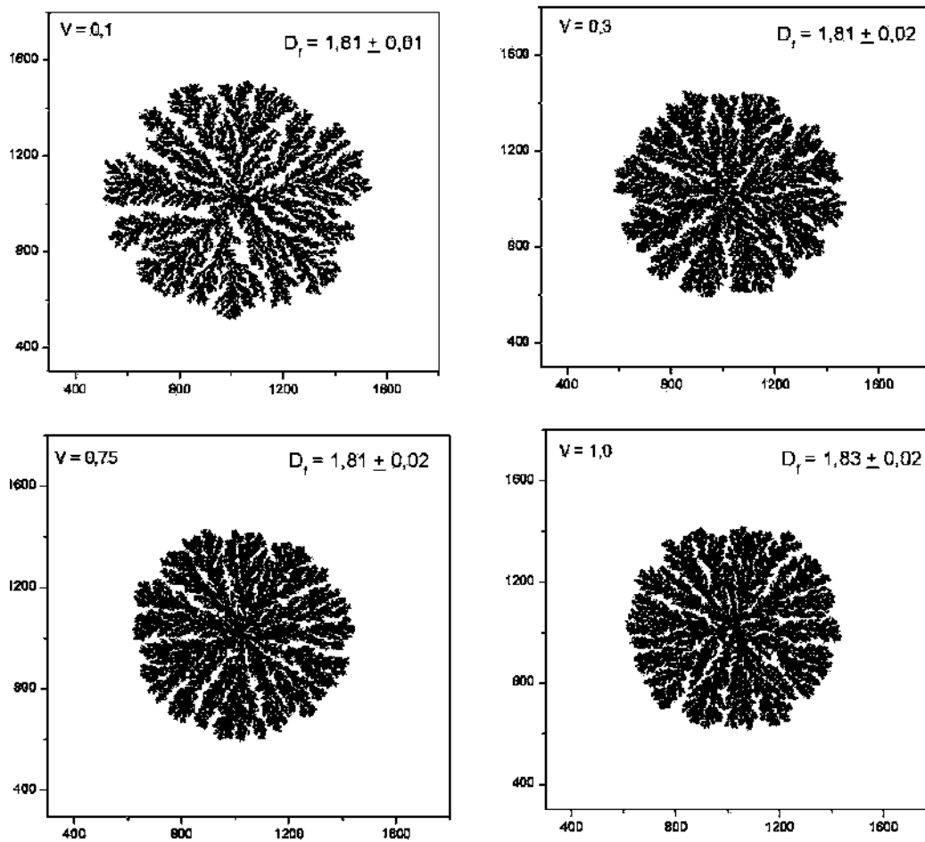
Figura 4.3: Variação da dimensão fractal em função do Potencial Elétrico. Todas as figuras são formadas por 100.000 partículas, 1/kT = 1 . (e) v = 0,1 (f) v = 0,3 (g) v = 0,75 (h) v = 1,0
