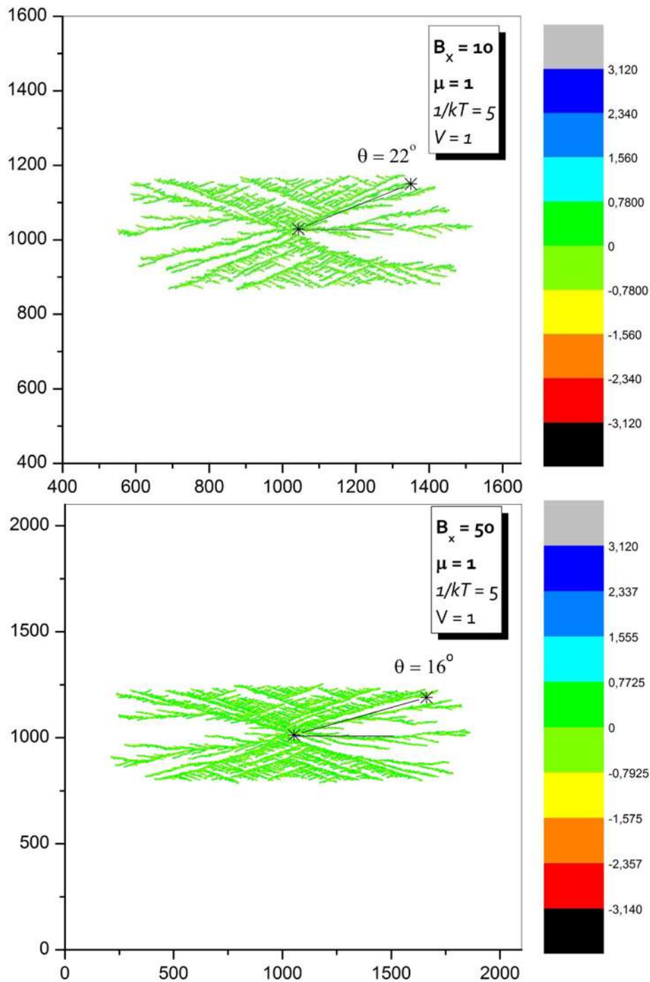
Figura 4.17: Agregados obtidos pela simulação com v = 1 , \mu = 1 e campo magnético aplicado: (e) B_x = 10 e (f) B_x = 50 . As cores representam faixas de valores dos ângulos de orientação do momento magnético das partículas do agregado em relação ao campo externo aplicado, conforme escala de cores à direita de cada gráfico.
