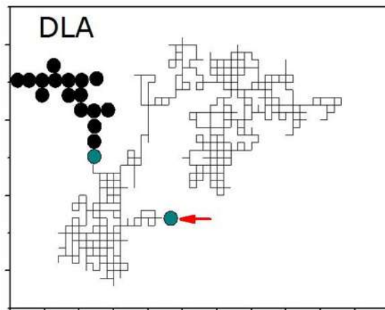
Figura 3.1: Exemplo da caminhada de uma partícula no algoritmo de DLA bidimensional. A partícula representada por um círculo verde executa um movimento tipo caminhada aleatória até atingir a região vizinha ao agregado, representado na figura pelo conjunto de círculos pretos.
