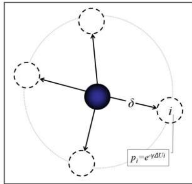
Figura 3.5: Esquema de caminhada para o algoritmo de DLA modificado sem rede.
