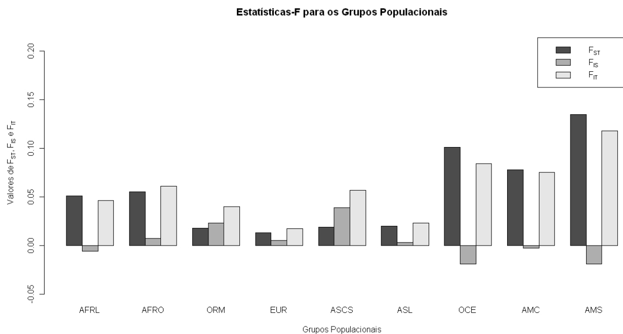
Gráfico 3: Valores das estatísticas-F ( F_{ST} , F_{IS} e F_{IT} ) dentro dos grupos populacionais.
