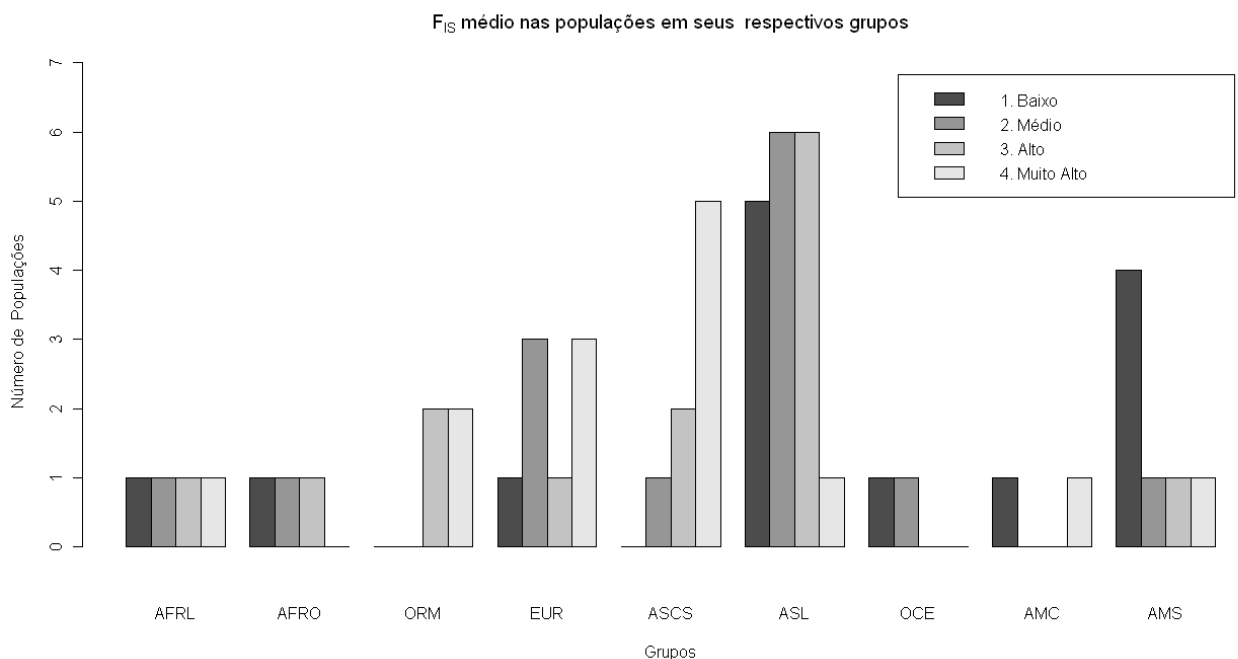
Gráfico 2: Classes* do coeficiente de endocruzamento, F_{IS} , dentro das populações, distribuídas ao longo de seus grupos.
