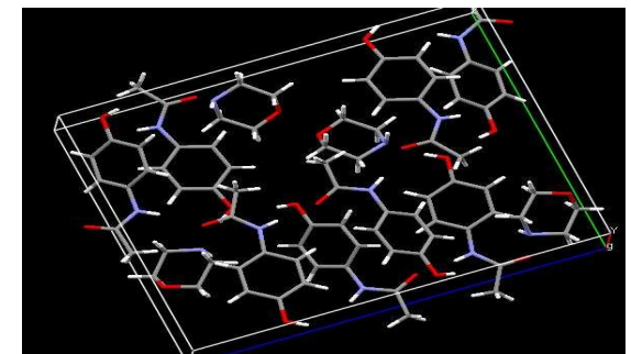
Figura 47 - Forma 30: empacotamento cristalino do Paracetamol: código CCDC MUPQET
