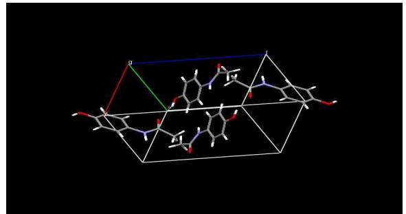
Figura 25 - Forma 08: empacotamento cristalino do Paracetamol: código CCDC HXACAN09
