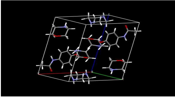
Figura 18 - Forma 01: empacotamento cristalino do Paracetamol: código CCDC AHEPUY
