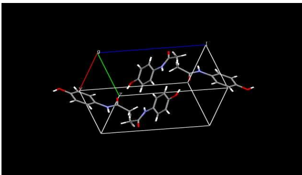
Figura 26 - Forma 09: empacotamento cristalino do Paracetamol: código CCDC HXACAN10
