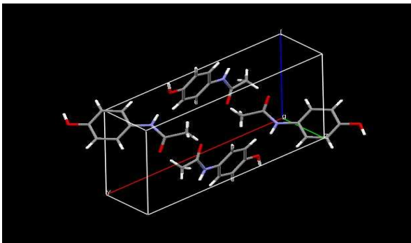
Figura 20 - Forma 03: empacotamento cristalino do Paracetamol: código CCDC HXACAN01
