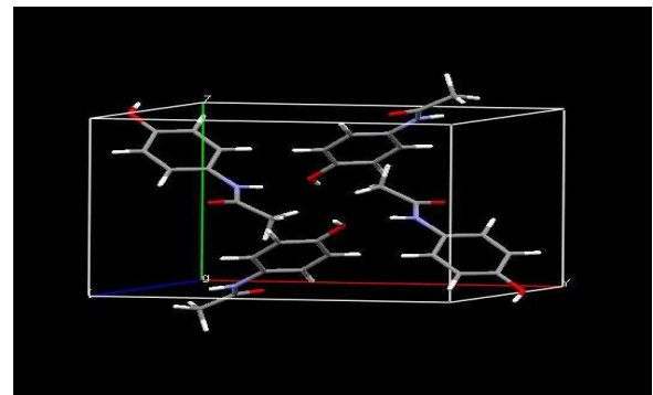
Figura 29 - Forma 12: empacotamento cristalino do Paracetamol: código CCDC HXACAN13
