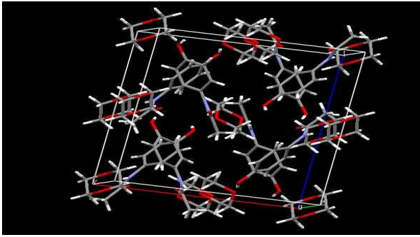
Figura 42 - Forma 25: empacotamento cristalino do Paracetamol: código CCDC MUPPES02
