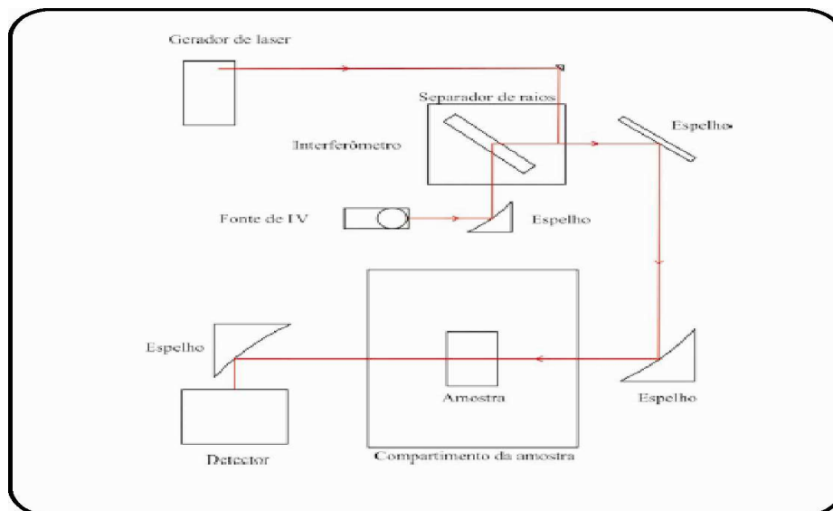
Figura 3 - Representação de um Espectrômetro de Infravermelho Simples
