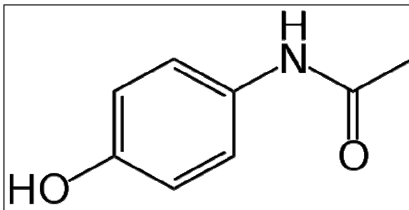
Figura 6 - Fórmula Estrutural do Paracetamol N -(4-hidroxifenil)etanamida PM151,163g/mol Formula molecular C_8H_9NO_2
