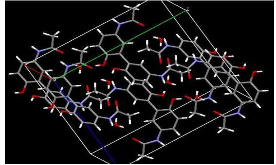
Figura 49 - Forma 32: empacotamento cristalino do Paracetamol: código CCDC SAZNEN
