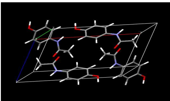
Figura 22 - Forma 05: empacotamento cristalino do Paracetamol: código CCDC HXACAN06
