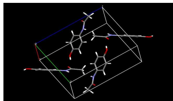
Figura 23 - Forma 06: empacotamento cristalino do Paracetamol: código CCDC HXACAN07
