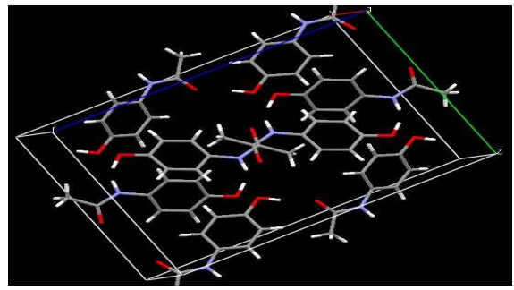
Figura 39 - Forma 22: empacotamento cristalino do Paracetamol: código CCDC HXACAN24
