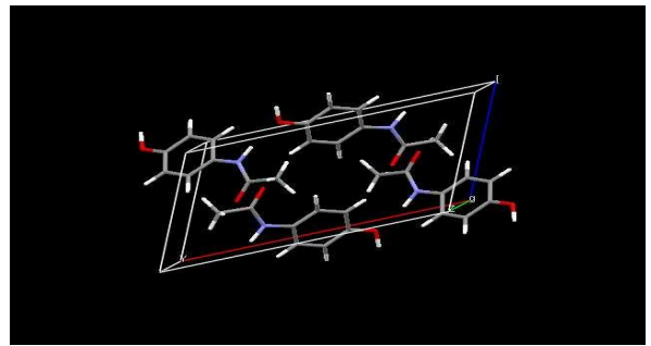
Figura 31 - Forma 14: empacotamento cristalino do Paracetamol: código CCDC HXACAN15
