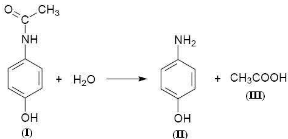
Equação 1 - Hidrólise do paracetamol
