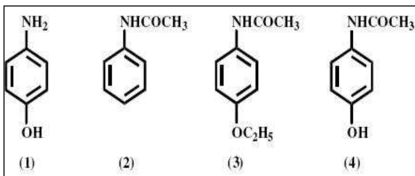
Figura 1 - Série de compostos derivados do para-Aminofenol. Legenda: (1) para-Aminofenol, (2) Acetanilida, (3) Fenacetina e (4) Paracetamol. (SILVA, 2002).
