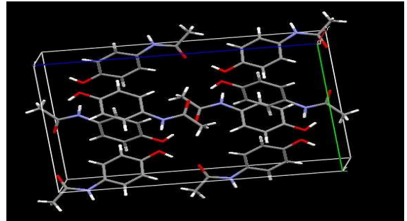
Figura 37 - Forma 20: empacotamento cristalino do Paracetamol: código CCDC HXACAN22
