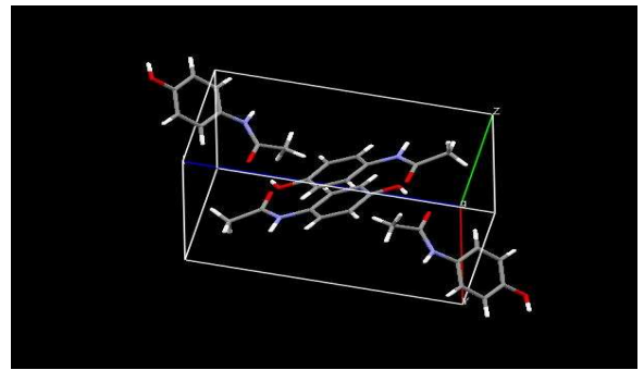
Figura 27 - Forma 10: empacotamento cristalino do Paracetamol: código CCDC HXACAN11
