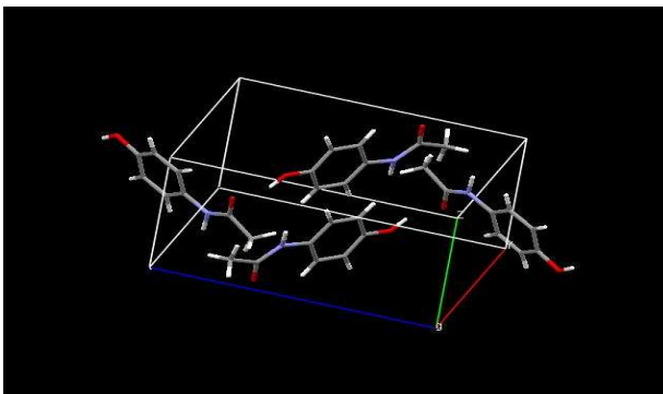
Figura 28 - Forma 11: empacotamento cristalino do Paracetamol: código CCDC HXACAN12
