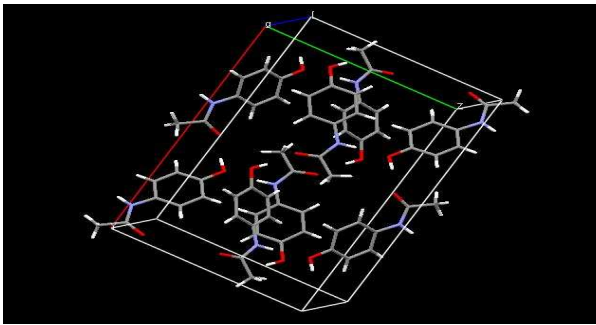
Figura 24 - Forma 07: empacotamento cristalino do Paracetamol: código CCDC HXACAN08
