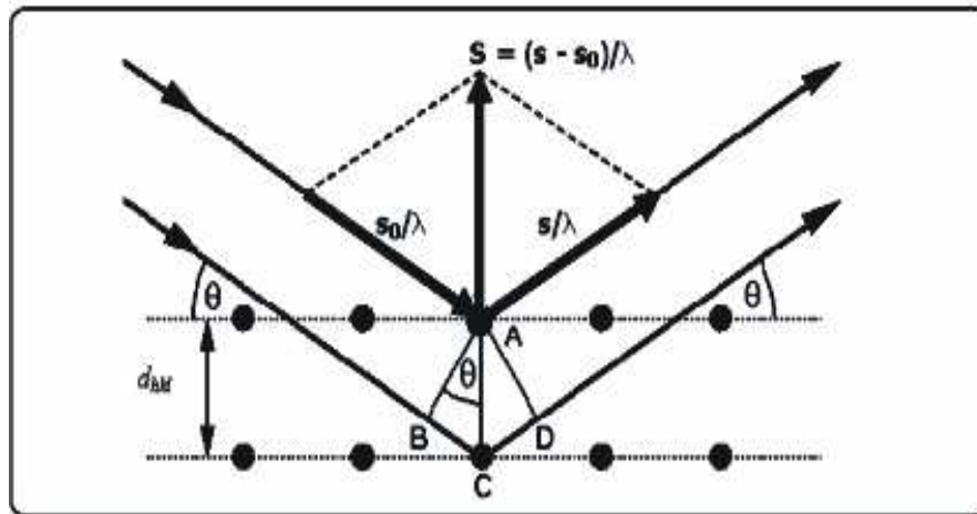
Figura 17 - Representação esquemática (fora de escala) da equação de Bragg.
