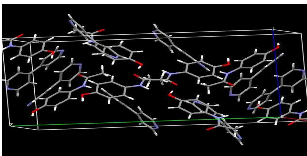
Figura 46 - Forma 29: empacotamento cristalino do Paracetamol: código CCDC MUPQAP
