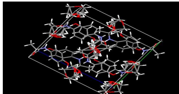
Figura 41 - Forma 24: empacotamento cristalino do Paracetamol: código CCDC MUPPES01
