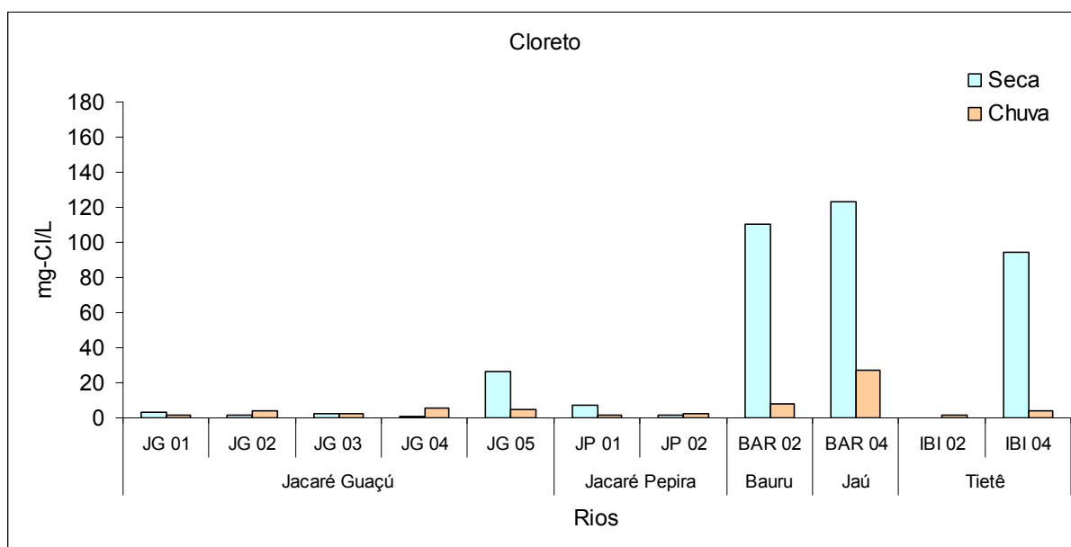
Figura 13 - Valores das concentrações de cloreto durante os períodos de seca e chuva, nos diferentes pontos de coleta.
