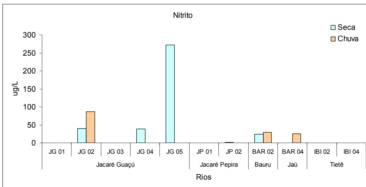
Figura 19 - Valores das concentrações de nitrito durante os períodos de seca e chuva, nos diferentes pontos de coleta.
