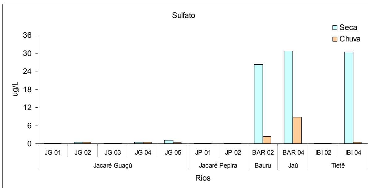
Figura 15 - Valores das concentrações de sulfato durante os períodos de seca e chuva, nos diferentes pontos de coleta.
