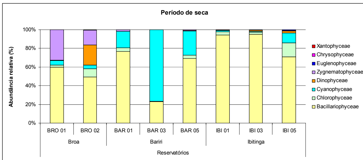
Figura 72 - Valores da abundância relativa das classes fitoplanctônicas, durante o período de seca, nos diferentes pontos de coleta dos reservatórios.
