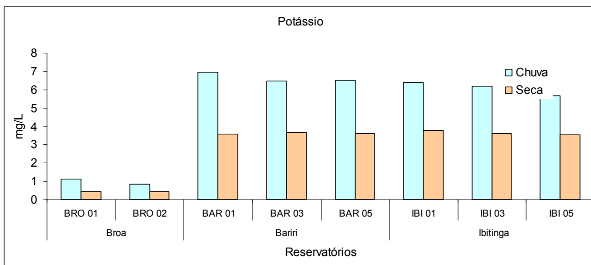
Figura 51 - Valores das concentrações de potássio durante os períodos de seca e chuva, nos diferentes pontos de coleta dos reservatórios do Broa, Bariri e Ibatinga.
