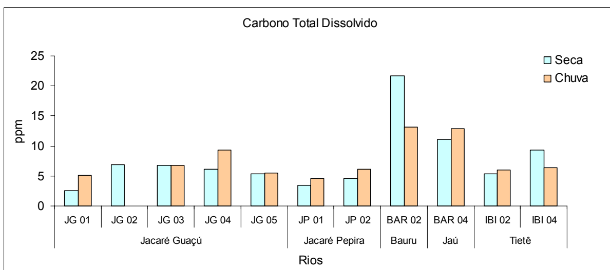
Figura 27 - Valores das concentrações de Carbono total dissolvido durante os períodos de seca e chuva, nos diferentes pontos de coleta.
