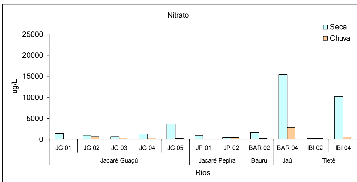
Figura 20 - Valores das concentrações de nitrato durante os períodos de seca e chuva, nos diferentes pontos de coleta.
