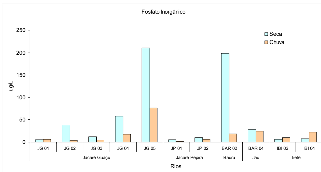
Figura 22- Valores das concentrações de fosfato inorgânico durante os períodos de seca e chuva, nos diferentes pontos de coleta.
