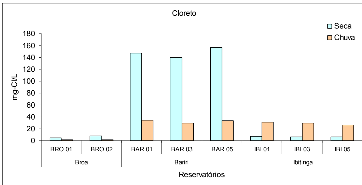
Figura 48 - Valores das concentrações de cloreto durante os períodos de seca e chuva, nos diferentes pontos de coleta dos reservatórios do Broa, Bariri e Ibitinga.
