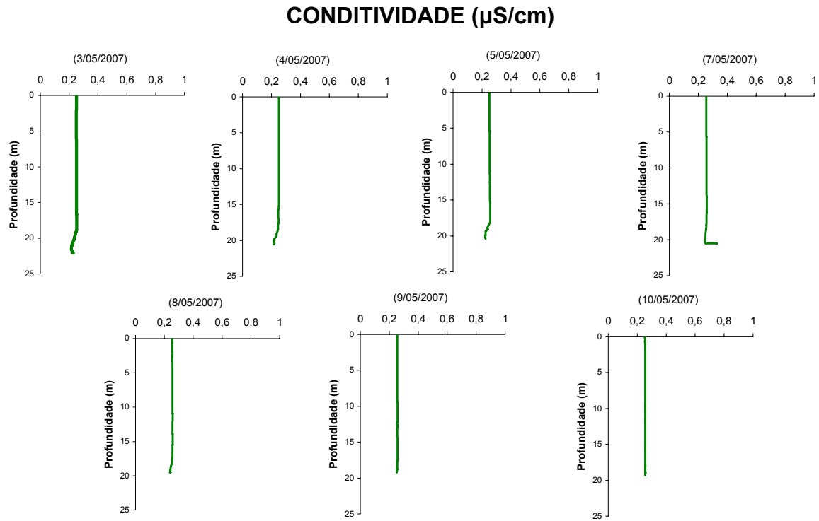
Figura 86 - Perfis verticais de condutividade na represa de Bariri durante o período de coleta de 3 a 10 de maio de 2007.
