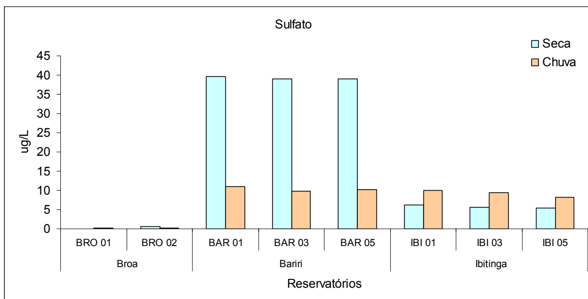
Figura 50 - Valores das concentrações de sulfato durante os períodos de seca e chuva, nos diferentes pontos de coleta dos reservatórios do Broa, Bariri e Ibatinga.
