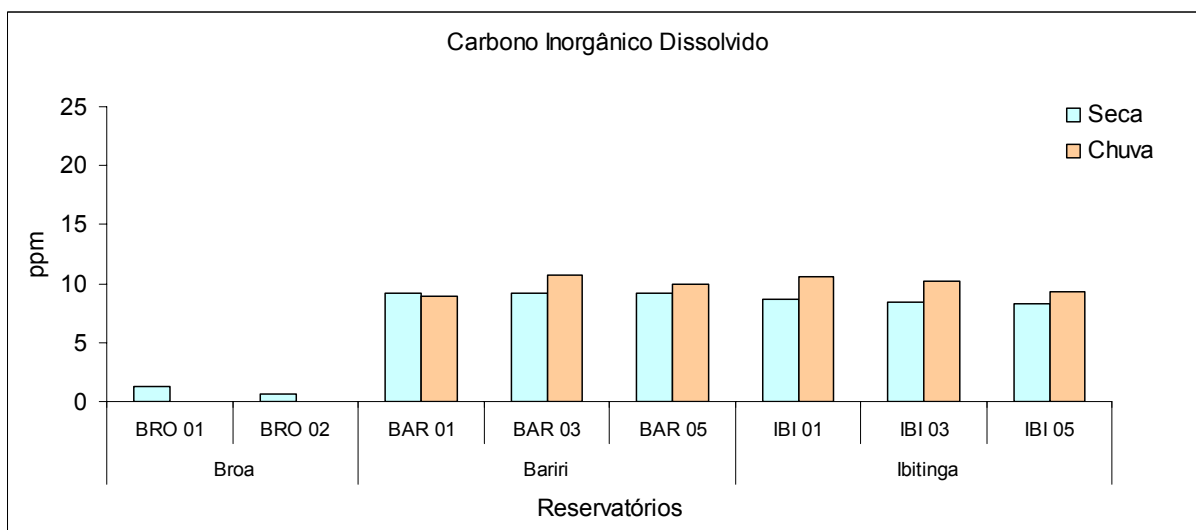
Figura 63 - Valores das concentrações de carbono inorgânico dissolvido durante os períodos de seca e chuva, nos diferentes pontos de coleta.
