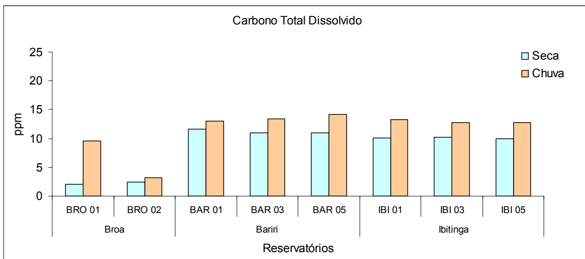
Figura 62 - Valores das concentrações de carbono total dissolvido durante os períodos de seca e chuva, nos diferentes pontos de coleta.
