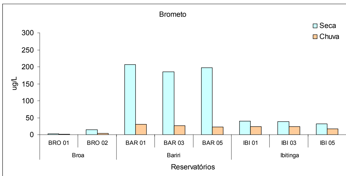
Figura 49 - Valores das concentrações de brometo durante os períodos de seca e chuva, nos diferentes pontos de coleta dos reservatórios do Broa, Bariri e Ibitinga.
