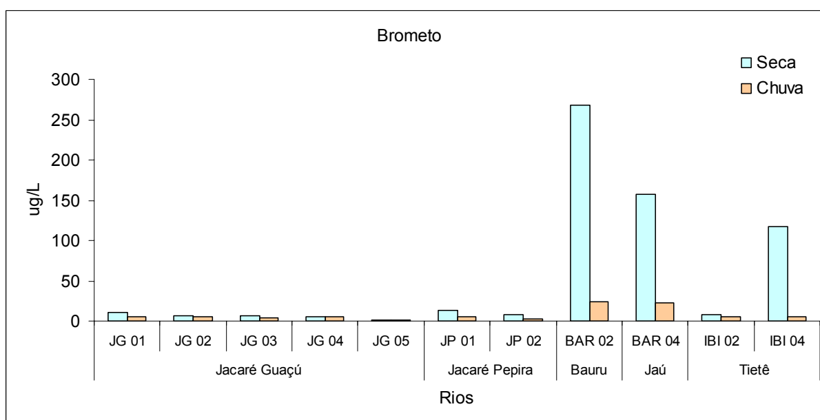
Figura 14 - Valores das concentrações de brometo durante os períodos de seca e chuva, nos diferentes pontos de coleta.
