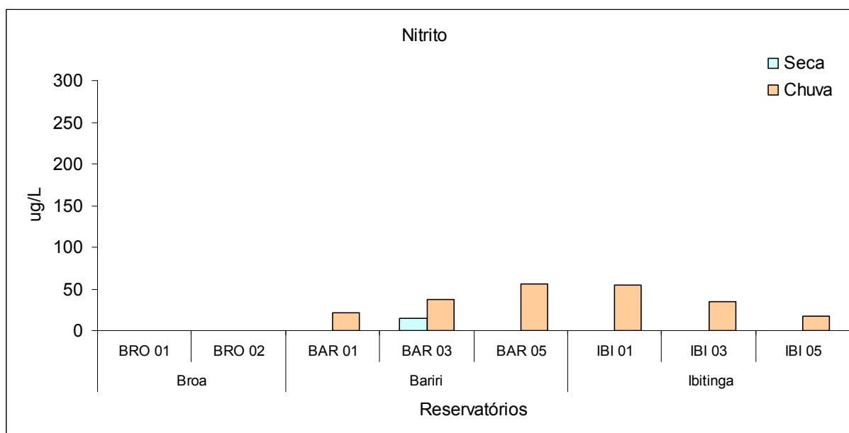
Figura 54 - Valores das concentrações de Nitrito durante os períodos de seca e chuva, nos diferentes pontos de coleta dos reservatórios do Broa, Bariri e Ibatinga.
