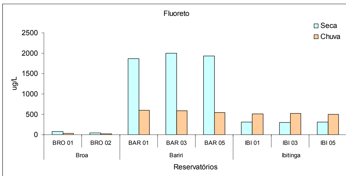
Figura 47 - Valores das concentrações de fluoreto durante os períodos de seca e chuva, nos diferentes pontos de coleta dos reservatórios do Broa, Bariri e Ibitinga.
