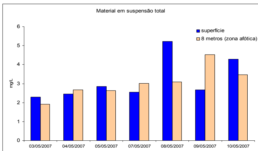
Figura 96 - Valores de material em suspensão total encontrados na superfície e a 8 metros de profundidade (zona afótica) nos diferentes dias de coleta na represa de Bariri.
