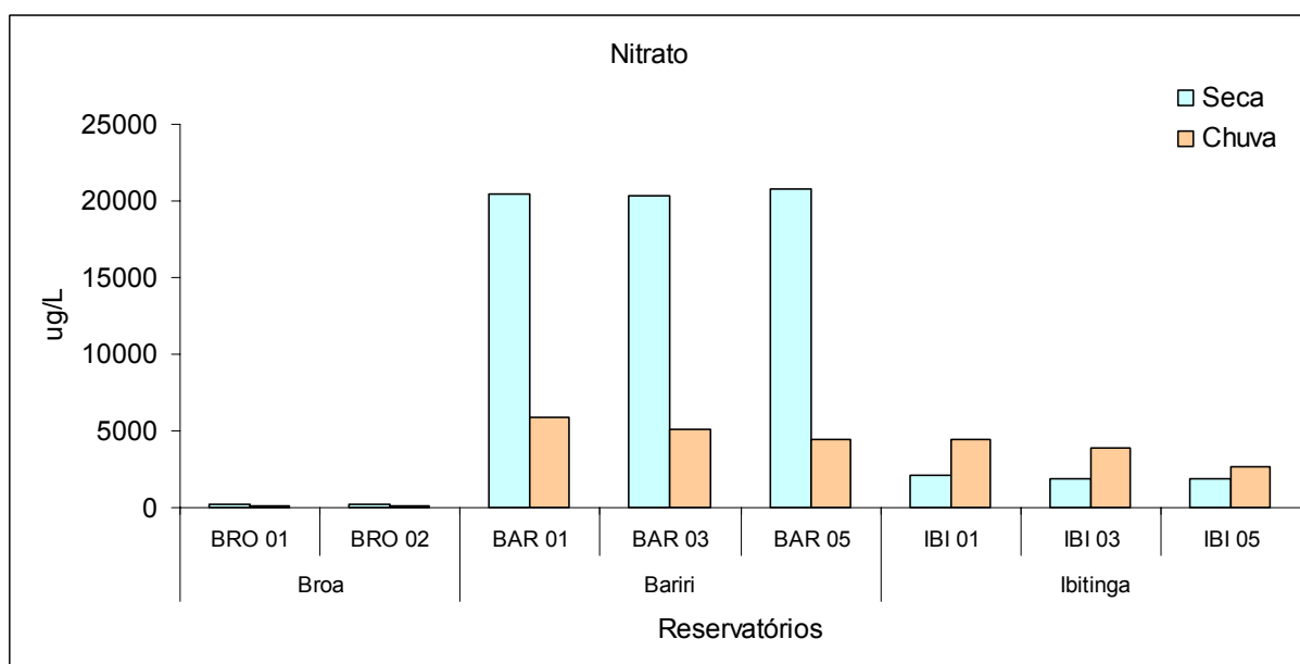
Figura 55 - Valores das concentrações de Nitrato durante os períodos de seca e chuva, nos diferentes pontos de coleta dos reservatórios do Broa, Bariri e Ibatinga.
