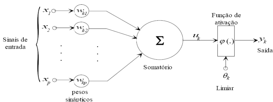
Figura 2.2. Neurônio matemático. Fonte: GALVÃO e VALENÇA (1999).
