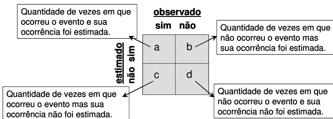
Figura 3.12. Esquema da tabela de contingência com análise comparativa dos acertos e erros nas estimativas da ocorrência (“sim”) e não ocorrência (“não”) de um determinado evento.
