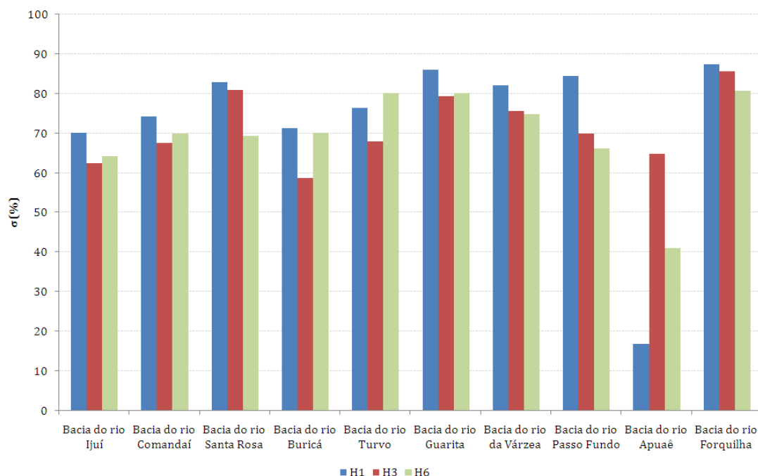
Figura 3.9. Percentual de ganho com a previsão de precipitação através do modelo climático, para os horizontes de 1, 3 e 6 meses.
