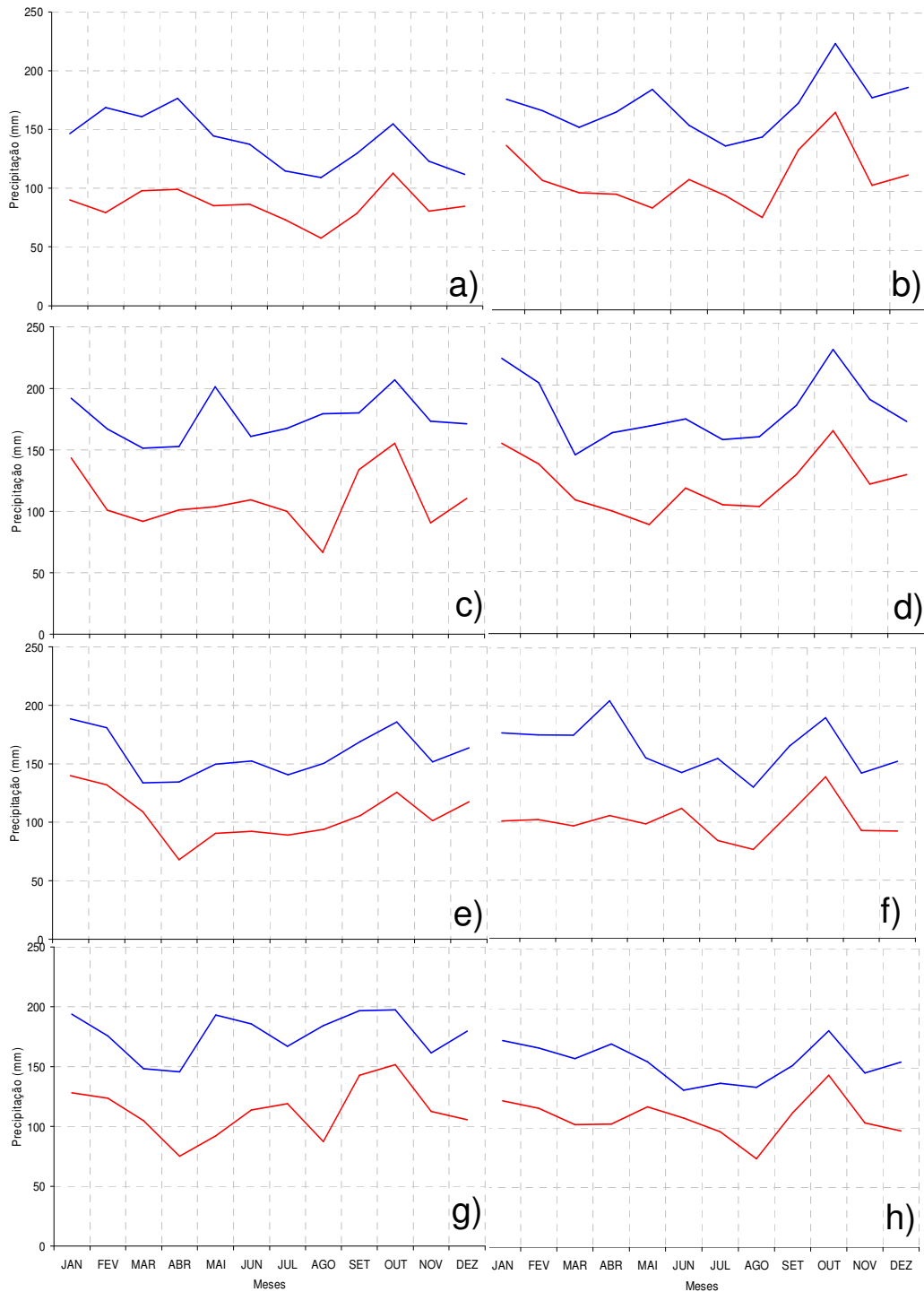
Figura A.4. Limites das 3 categorias de precipitação mensal: acima da normal (acima da linha azul), abaixo da normal (abaixo da linha vermelha) e normal (entre a linha azul e vermelha) para as 7 regiões homogêneas: Região 1 (a), Região 2 (b), Região 3 (c), Região 4 (d), Região 5 (e), Região 6 (f), Região 7 (g), Média da Bacia (h).
