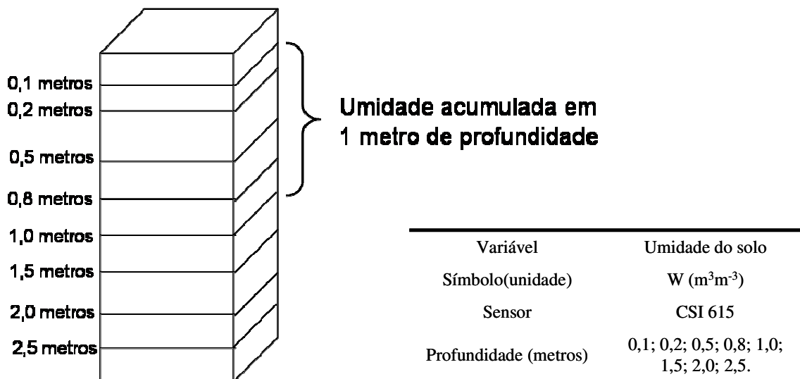
Figura 2.9. Descrição da coleta de umidade do solo no sitio experimental de cerrado ss.
