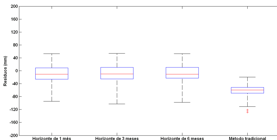
Figura 3.25. Resíduos do modelo de previsão de umidade do solo (diagrama de caixa)- Bacia do rio Comandai. A linha horizontal no interior das caixas representa o percentil 50 (mediana); o final das caixas, os percentis 25 e 75; as barras, os percentis 10 e 90; o símbolo de cruz representa os valores extremos.
