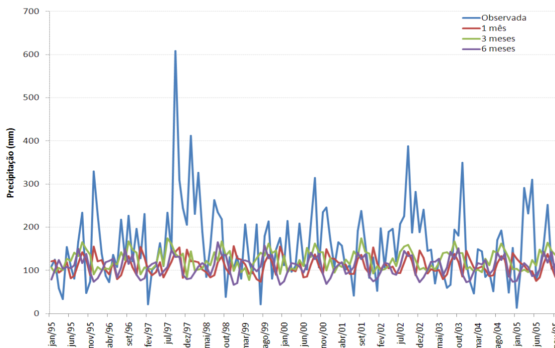
Figura 3.10. Comparação entre a precipitação observada e a precipitação prevista através do modelo global CFS para os horizontes de 1, 3 e 6 meses. (Precipitação média da área de estudo).
