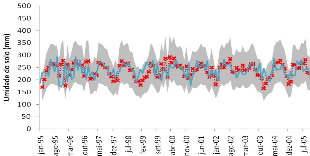
Figura 3.18. Previsão de umidade do solo com intervalo de confiança para o horizonte de 6 meses – Bacia do Rio Turvo.
