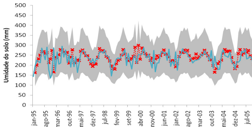
Figura 3.19. Previsão de umidade do solo com intervalo de confiança para o horizonte de 6 meses – Bacia do Rio Guarita.
