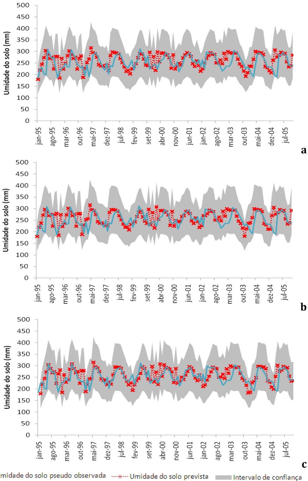
Figura 3.17. Previsão de umidade do solo com intervalo de confiança para o horizonte de 6 meses – Bacia do Rio Buricá.
