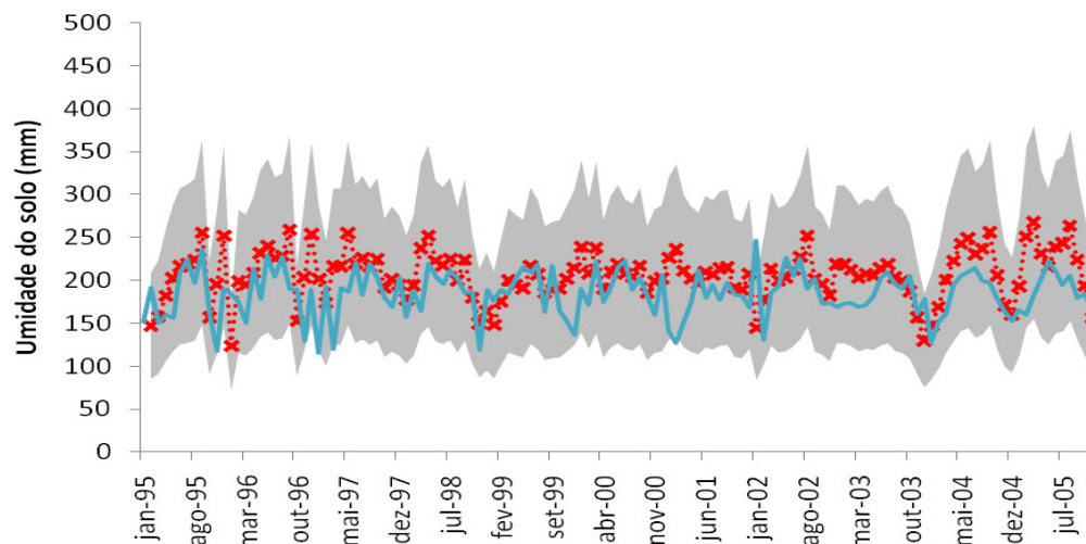
Figura 3.21. Previsão de umidade do solo com intervalo de confiança para o horizonte de 6 meses – Bacia do Rio Passo fundo.
