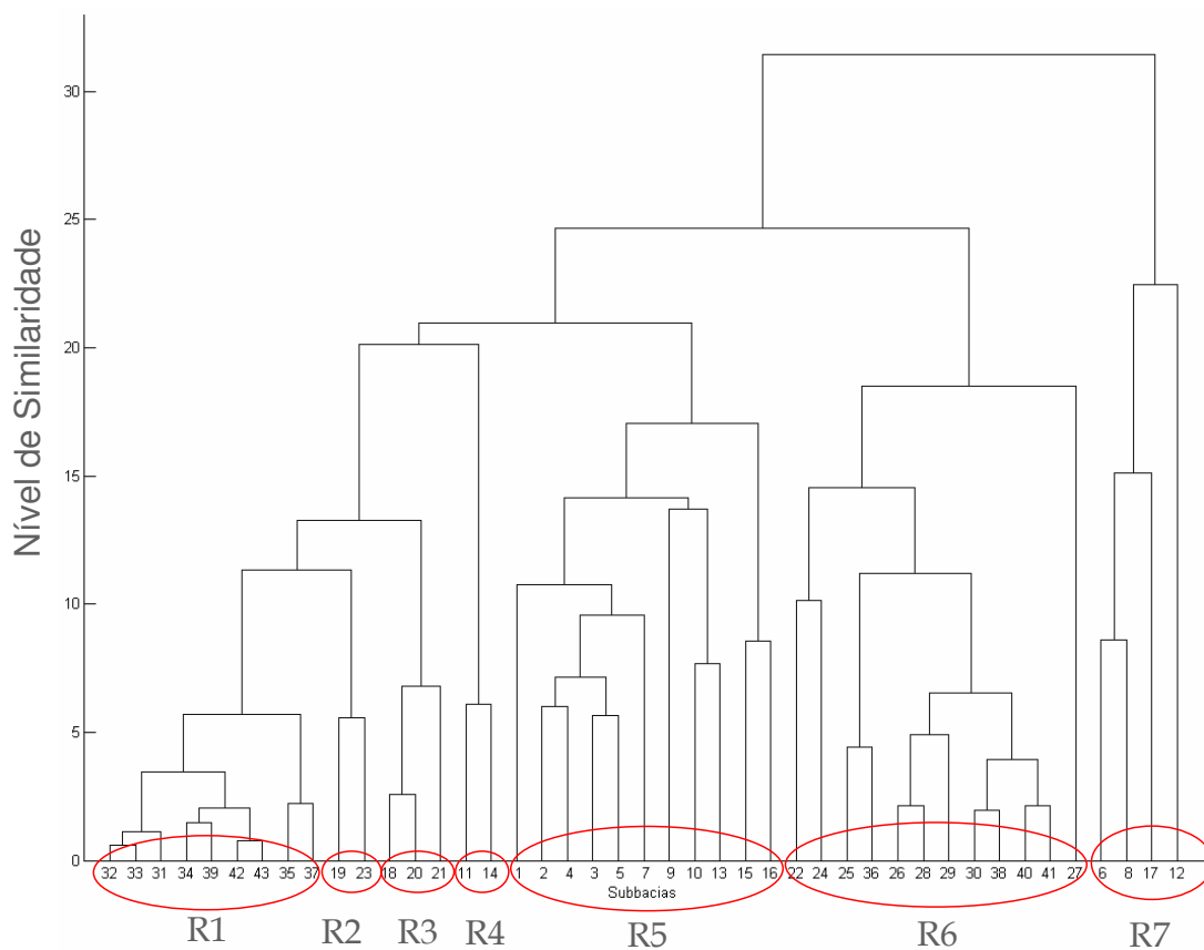
Figura A.2. Dendrograma do agrupamento feito pelo método da ligação completa com dados padronizados de precipitação das 43 subbacias do rio Uruguai, período de 1950 a 2005.
