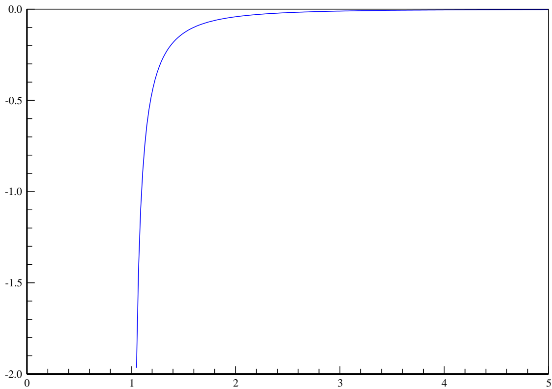
Figura A.9: Gráfico do tempo de reflexão contra a variável \gamma_0 para um degrau de potencial puramente quaterniônico [ V(x) = jV_3(x) - kV_2(x) ]. O gráfico mostra o instante t = 2\hbar\theta'(\gamma_0)/\sqrt{V_2^2 + V_3^2} em que o máximo da onda refletida atinge o ponto x = 0 . A variável \gamma_0 representa a razão entre a energia E da partícula e a perturbação quaterniônica \sqrt{V_2^2 + V_3^2} , calculada em E_0 . Observamos que \gamma_0 > 1 . É interessante notar que na mecânica quântica complexa, para o degrau de potencial, o tempo de reflexão é nulo no caso E_0 > V_1 ( V_1 é um potencial real).
