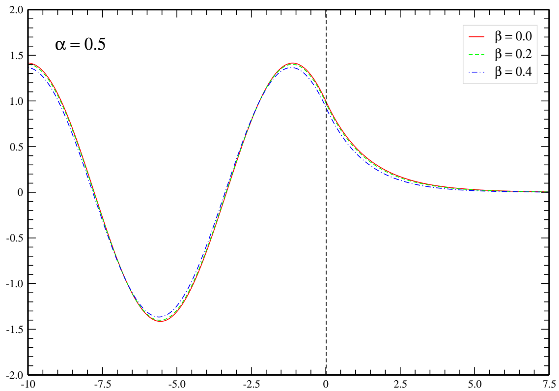
Figura A.2: Gráficos da parte real da função de onda estacionária quaterniônica contra a variável espacial adimensional \sqrt{2mV_1} x/\hbar . O espaço está dividido pela região I ( x < 0 ), onde não existe potencial, e região II ( x > 0 ), cujo potencial é constante ( V_1 + jV_3 - kV_2 ). A constante \alpha é a razão entre a energia da partícula e o potencial real V_1 da mecânica quântica complexa. A constante \beta representa a razão entre a perturbação quaterniônica \sqrt{V_2^2 + V_3^2} e o potencial V_1 .
