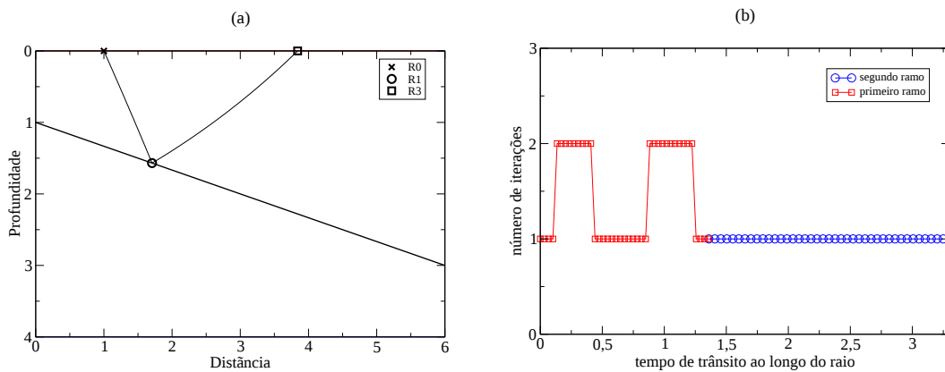
Figura 4.10: (a) Raio em um meio com velocidade afim, partindo do ponto (1,0) com direção inicial 25^\circ . (b) Número de iterações do método de Newton para avaliar quantidades ao longo de cada segmento do raio.
