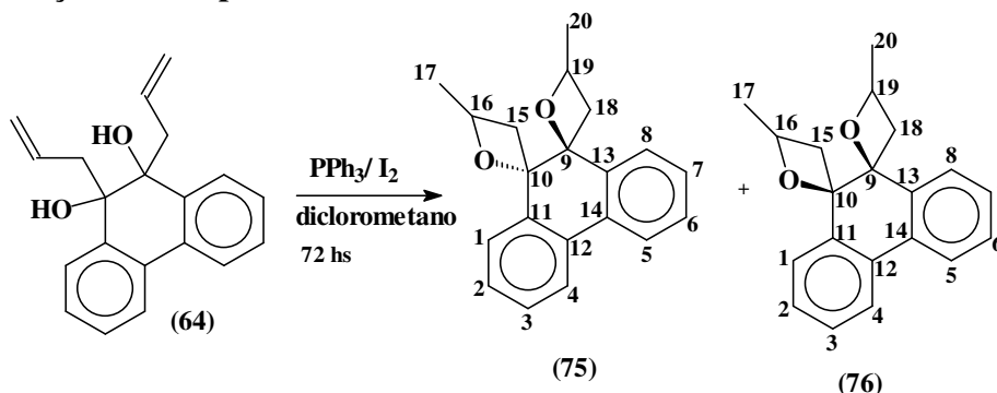
Figura 72: Reação do composto 64 com trifetilfosfina e iodo. (Também nesta figura foi usada nos produtos numeração que facilita comparações dos espectros).
