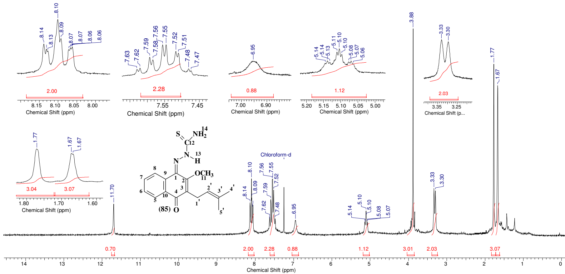
Espectro 118: RMN de ^1\text{H} do composto 85 .
