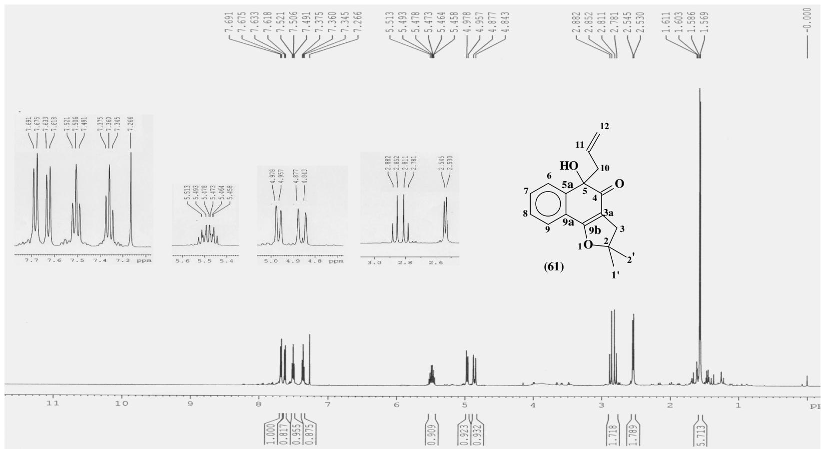
Espectro 37: RMN de 1 H do composto 61 .
