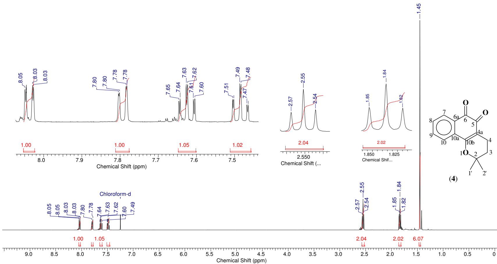
Espectro 7: RMN de 1 H da β-lapachona (4).
