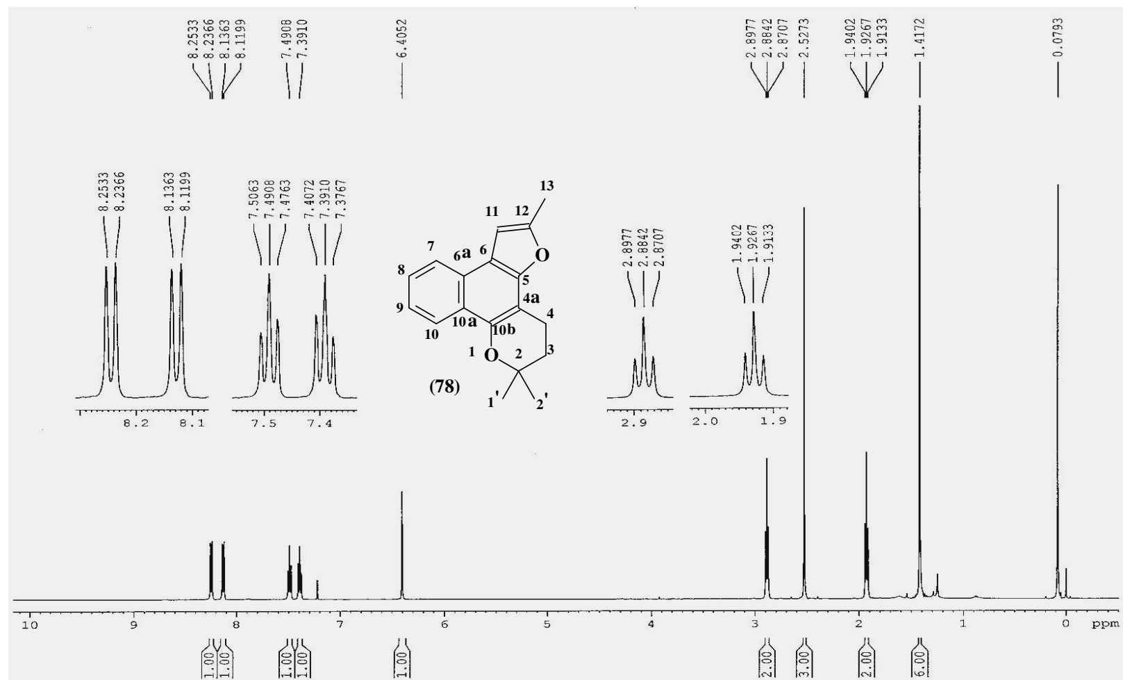
Espectro 86: RMN de ^1\text{H} do composto 78 .
