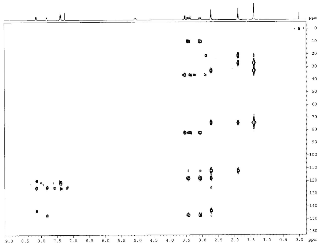
Espectro 61: RMN HET-COSY ( J^2 e J^3 ) do composto 71 .
