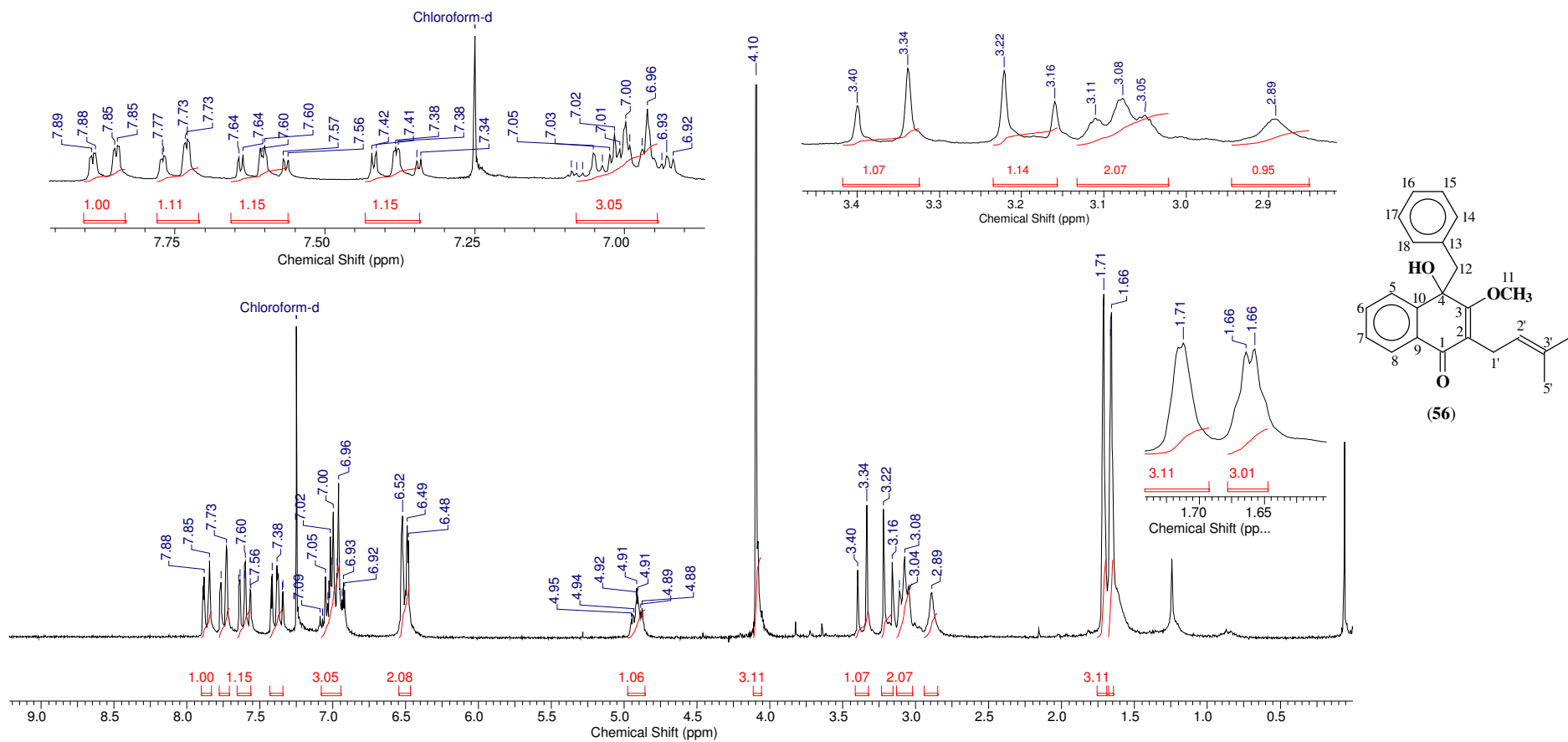
Espectro 19: RMN de 1 H do composto 56 .
