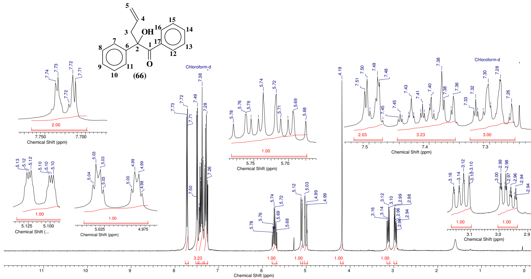
Espectro 49: RMN 1 H do composto 66.
