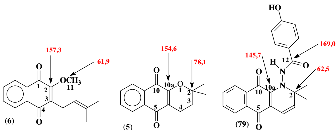
Figura 115: Deslocamentos químicos dos carbonos do 2-metóxi-lapachol (6), da \alpha -lapachona (5) e do composto 87.
