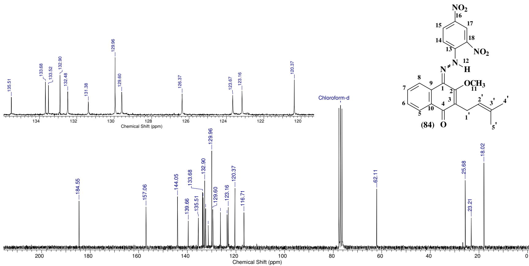
Espectro 115: RMN de ^{13}\text{C} do composto 84 .
