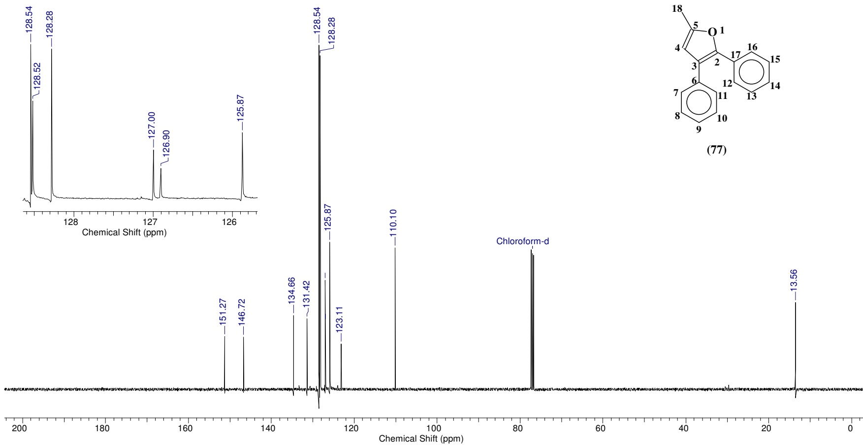
Espectro 83: RMN 13 C do composto 77.
