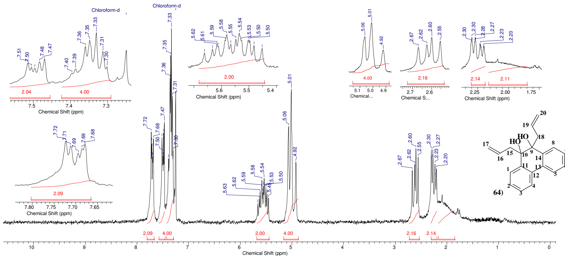
Espectro 45: RMN 1 H do composto 64 .
