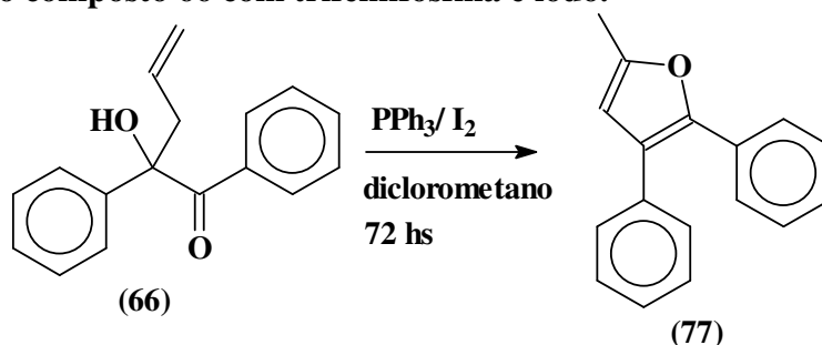
Figura 73: Reação do composto 66 com trifetilfosfina e iodo.
