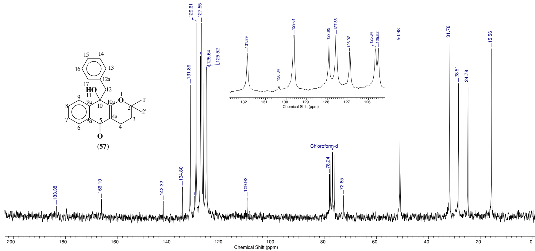
Espectro 24: RMN de 13 C do composto 57 .
