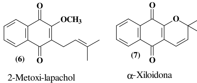
Figura 13: Outras naftoquinonas encontradas no ipê-roxo.
