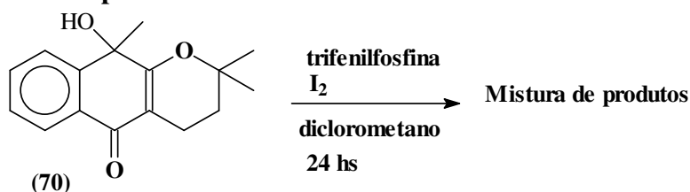
Figura 67: Reação do composto 70 com trifetilfosfina e iodo.
