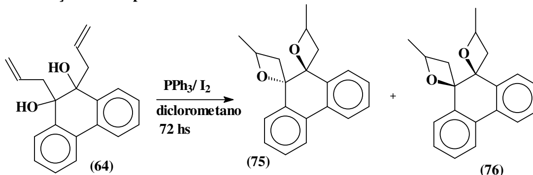
Figura 72: Reação do composto 64 com trifetilfosfina e iodo.
