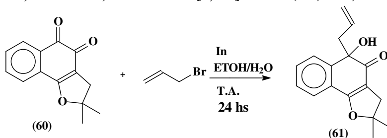
Figura 57: Reação da nor - \beta -lapachona (60) com brometo de alila e índio.
