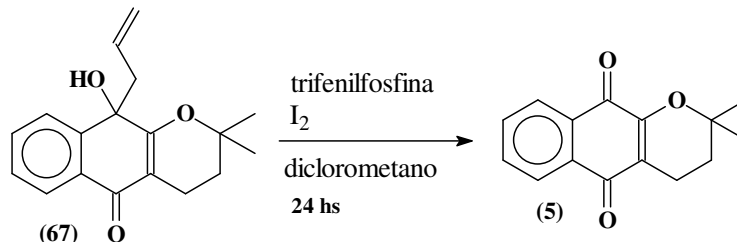
Figura 65: Reação do composto 67 com trifenilfosfina e iodo. OBS: Esta Figura tem numeração inferior a 98, porque ela já está presente na parte experimental.
