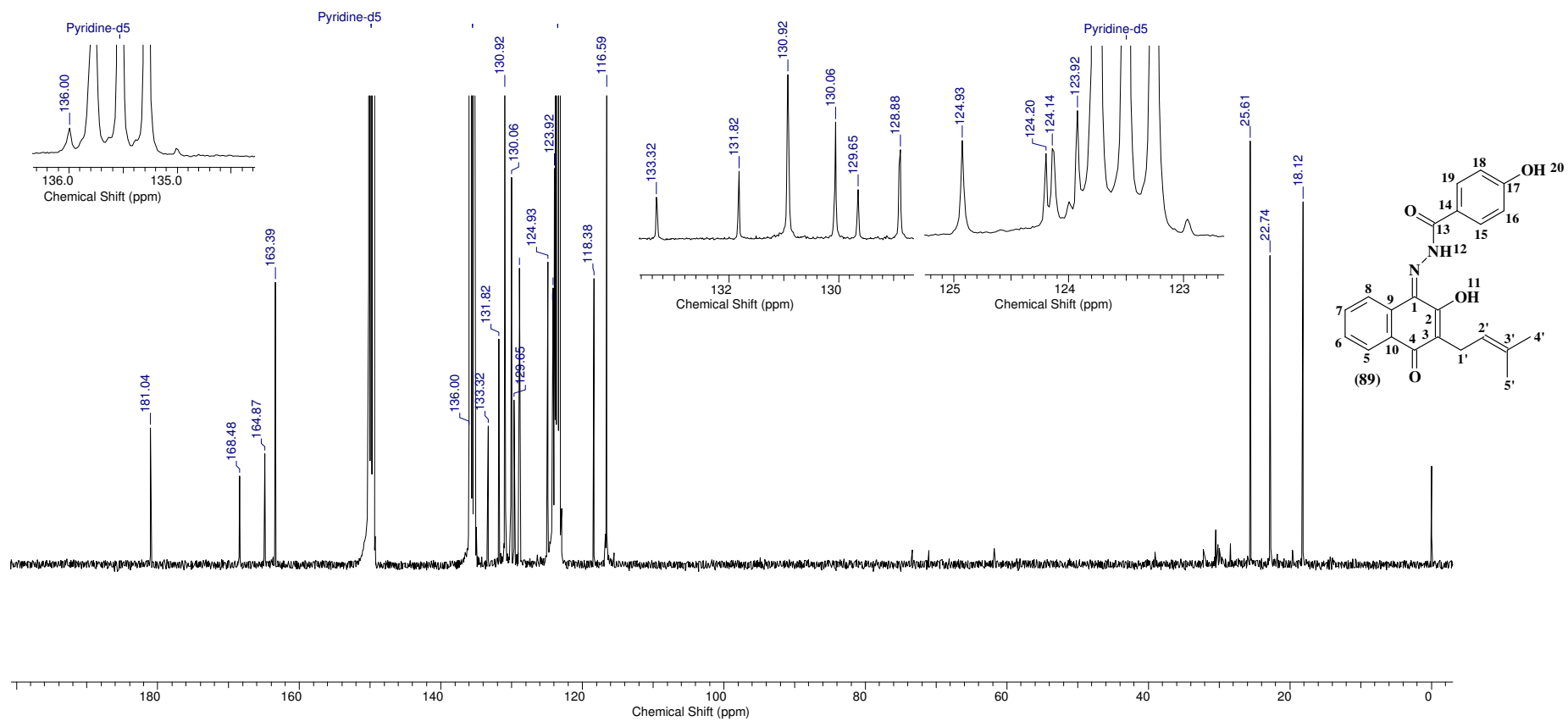
Espectro 144: RMN ^{13}\text{C} do composto 89 em piridina deuturada.
