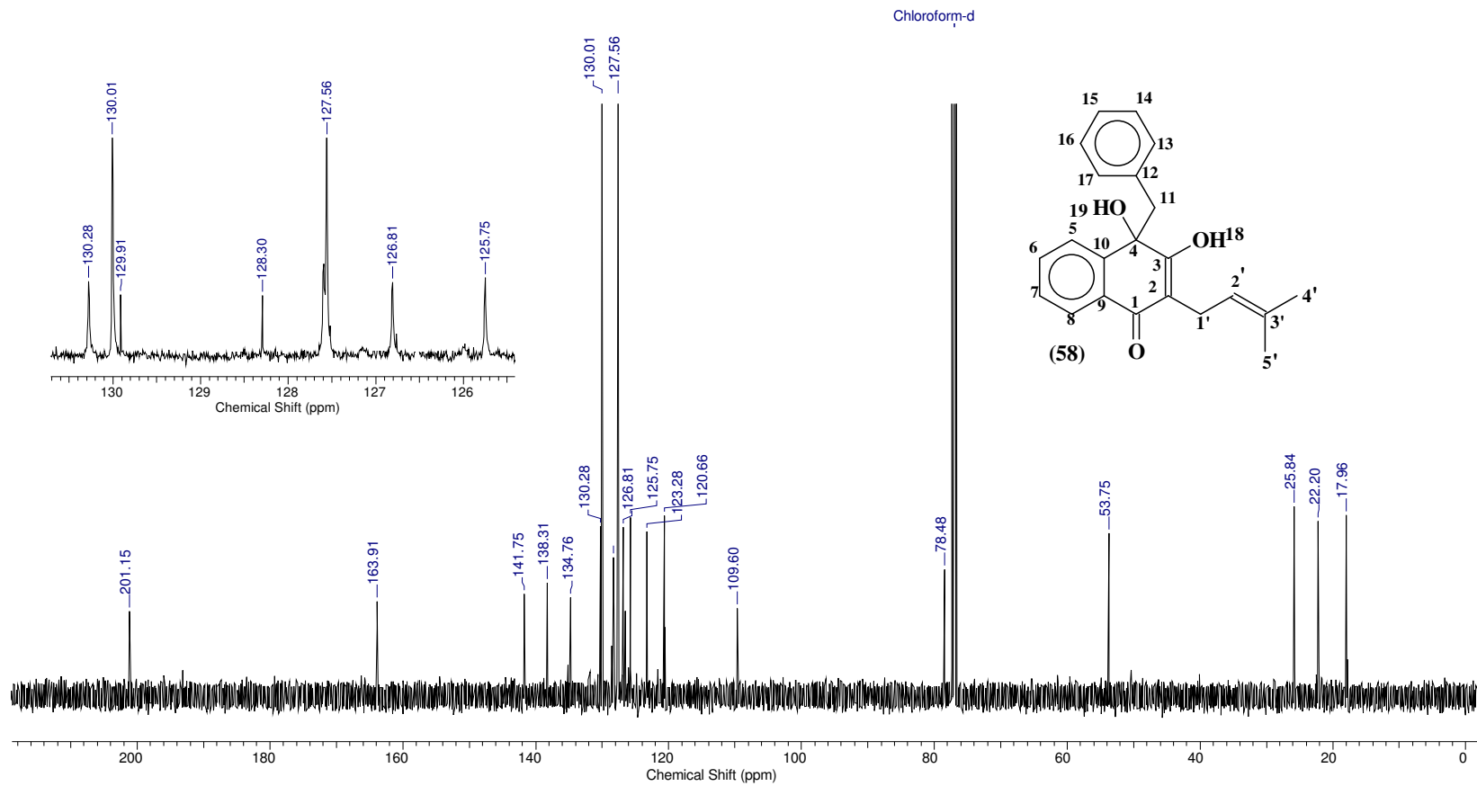
Espectro 28: RMN de ^{13}\text{C} do composto 58 .
