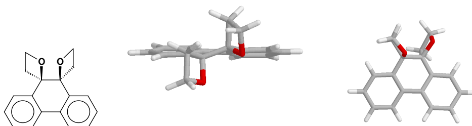
Figura 103: Estruturas em 3D do composto 76 .
