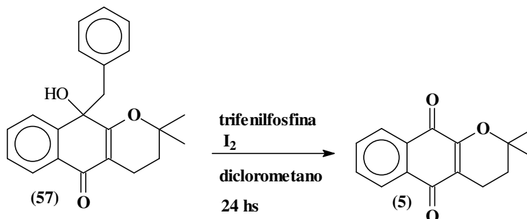
Figura 66: Reação do composto 57 com trifetilfosfina e iodo.
