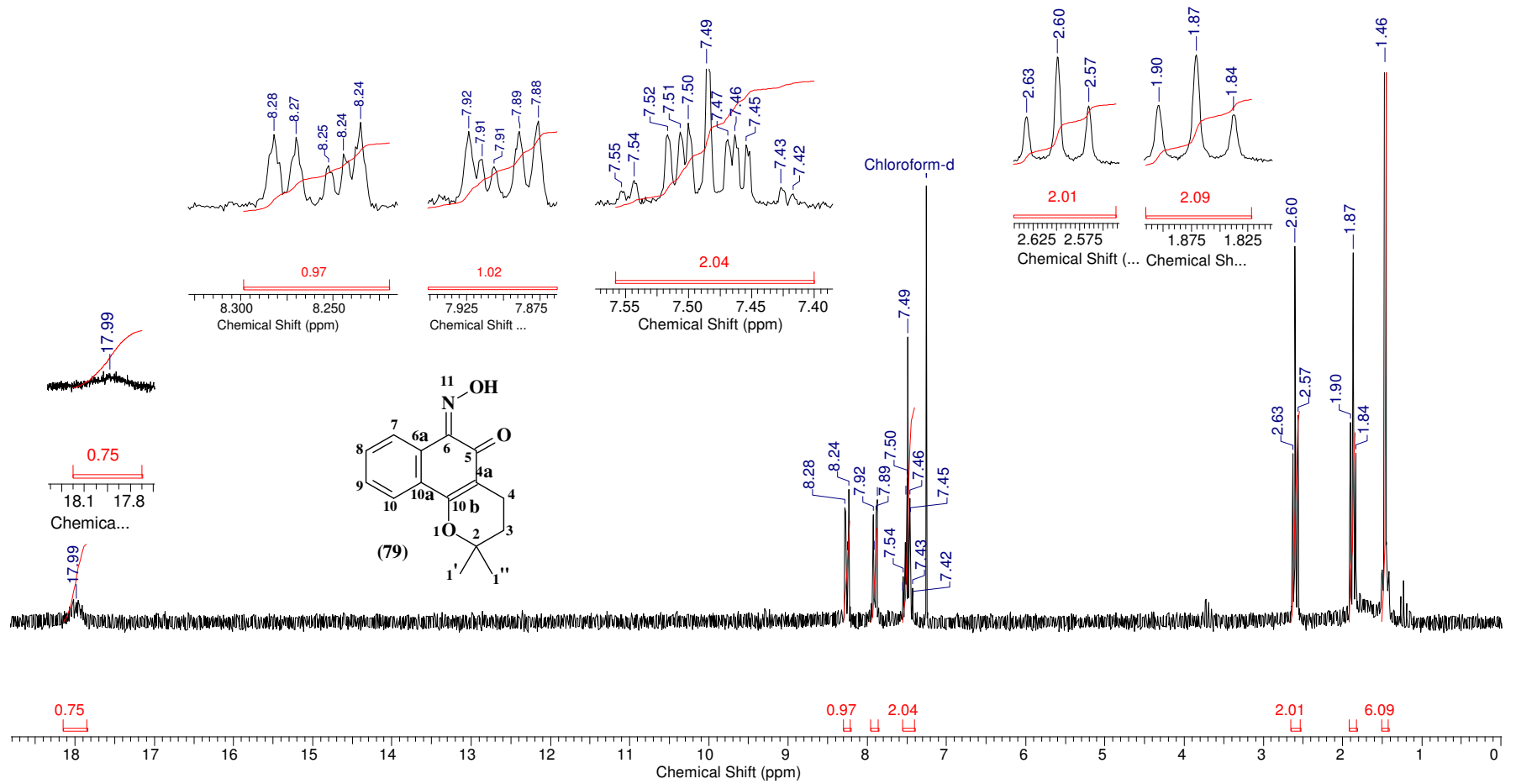
Espectro 90: RMN de ^1\text{H} do composto 79.
