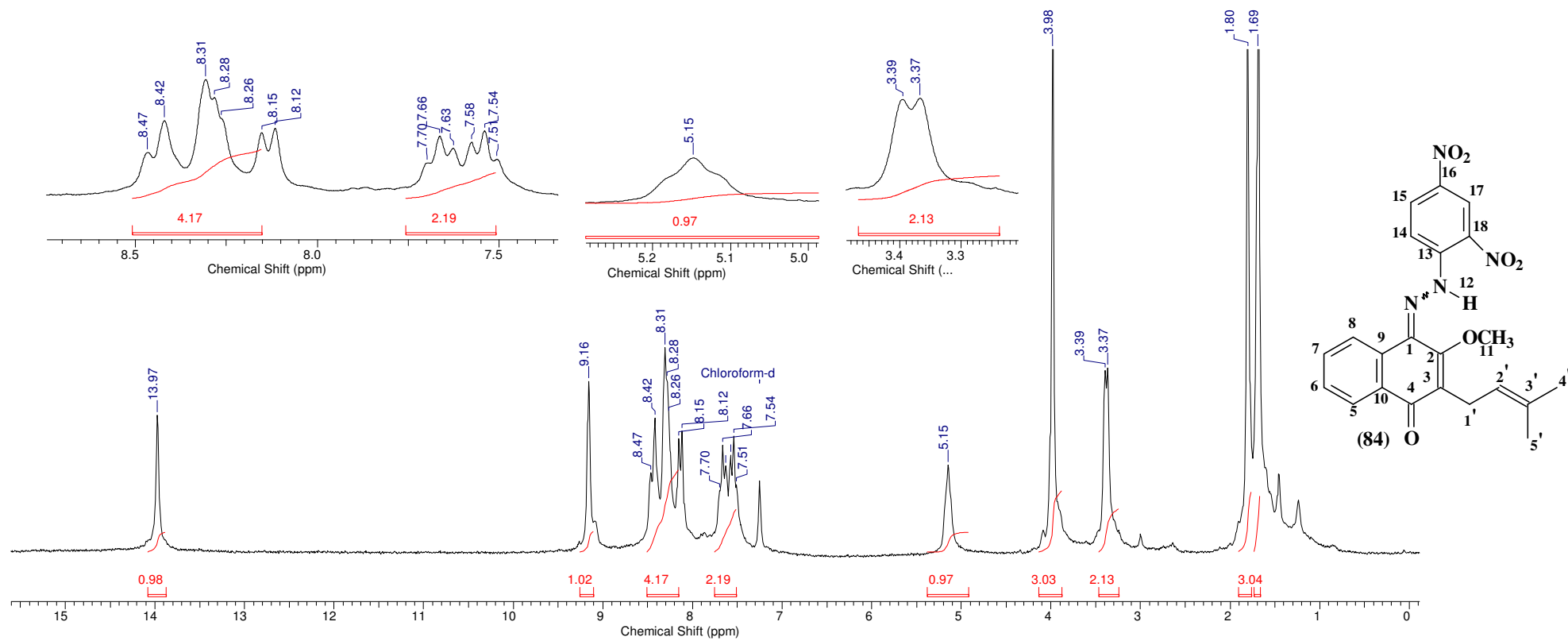
Espectro 114: RMN de 1 H do composto 84 .
