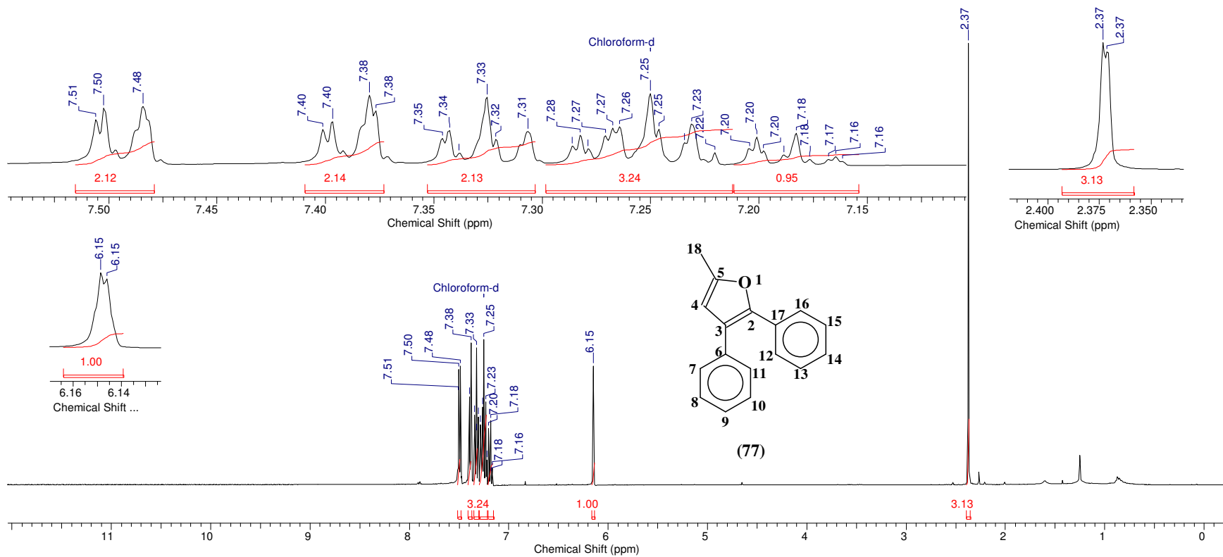
Espectro 82: RMN ^1\text{H} do composto 77 .
