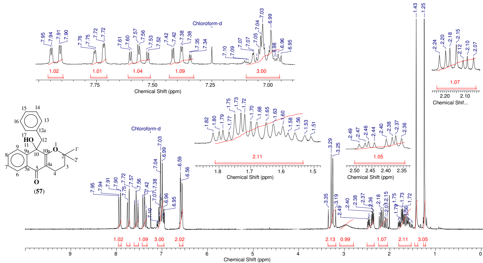
Espectro 23: RMN de 1 H do composto 57 .
