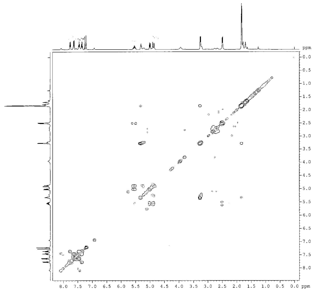
Espectro 33: RMN de H x H COSY do composto 59 .
