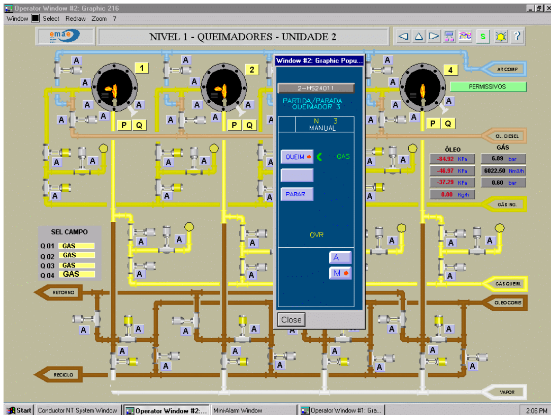
Figura 52 - Tela e interface de comando de acionamento do conjunto queimador
