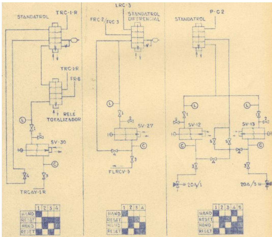
Figura 12 - Válvulas seletoras de controle das caldeiras 1 e 2
