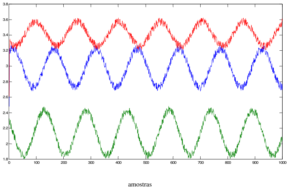
Figura 7.4 – Sinais elétricos dos sensores
