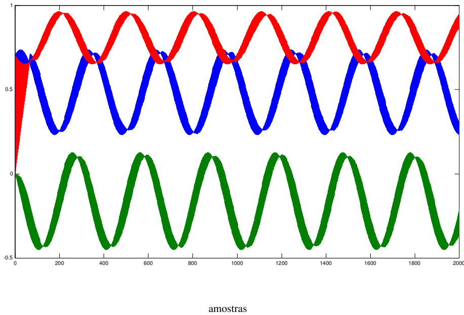
Figura 7.6 – Sinais após Filtro passa-baixa
