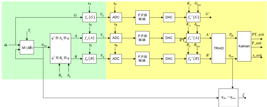
Figura 1.2 – Diagrama de bloco dos dois subsistemas
