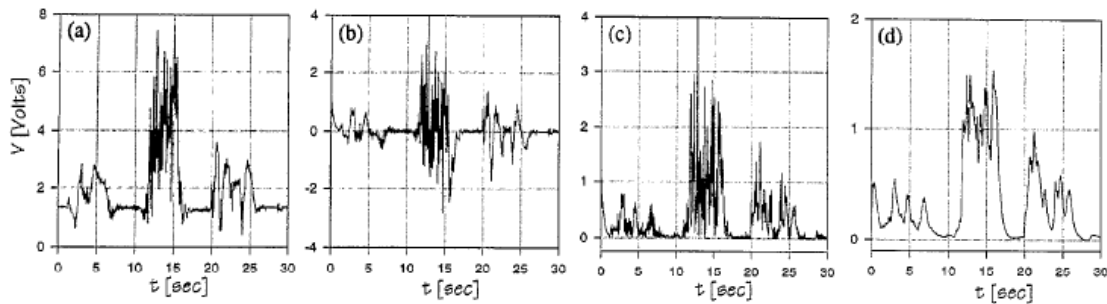
Figura 6.1 – Representação do funcionamento detector de momentos estáticos: (a) o sinal composto do acelerômetro; (b) o sinal depois do filtro passa-alta; (c) o sinal depois do retificador; (d) o sinal depois do filtro passa-baixa.
