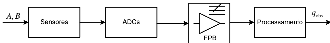
Figura 7.5 – Subsistema de determinação de atitude
