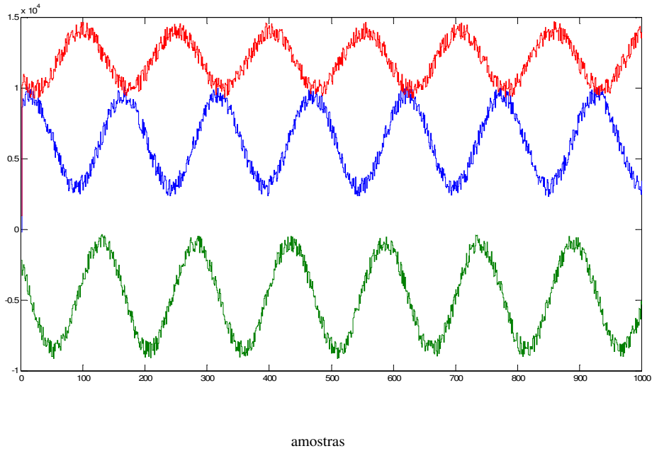
Figura 7.7 – Sinais dos sensores após conversão AD
