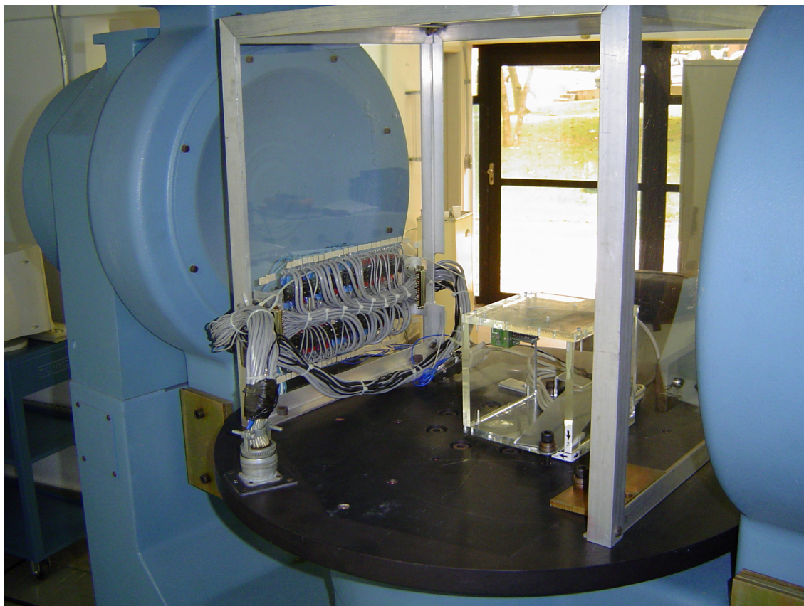
Figura 1.3 – Mesa de rotação. Protótipo do determinador de atitude no interior da mesa
