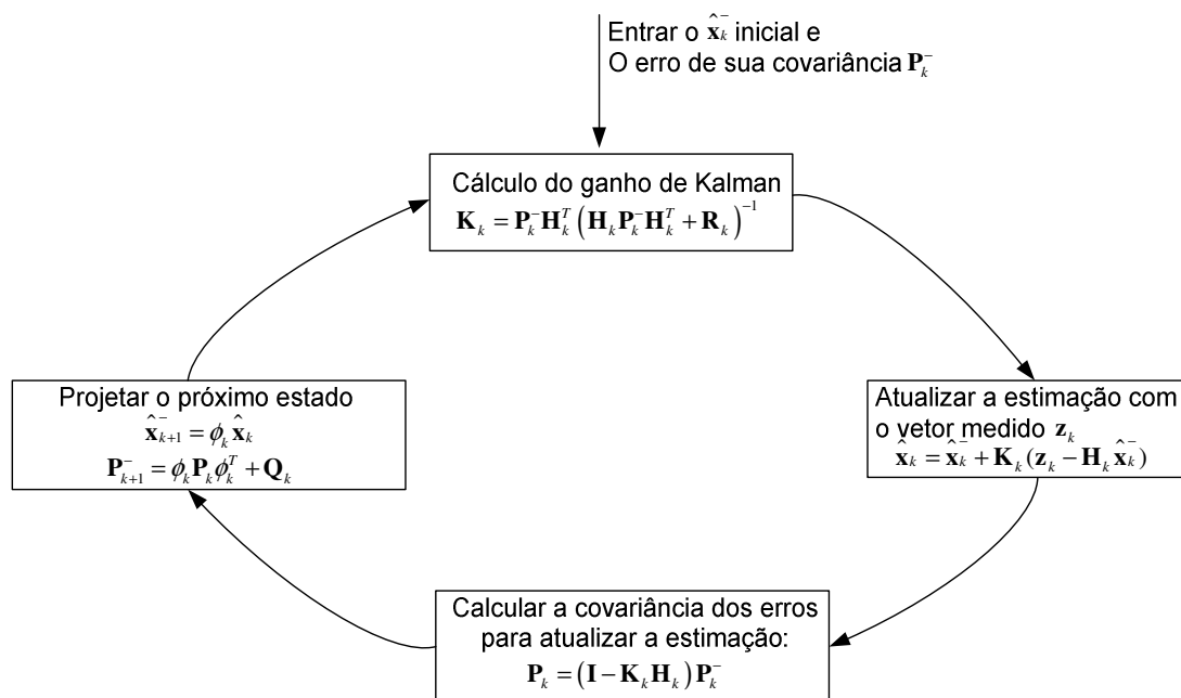
Figura 4.1 – Fluxograma do Filtro de Kalman
