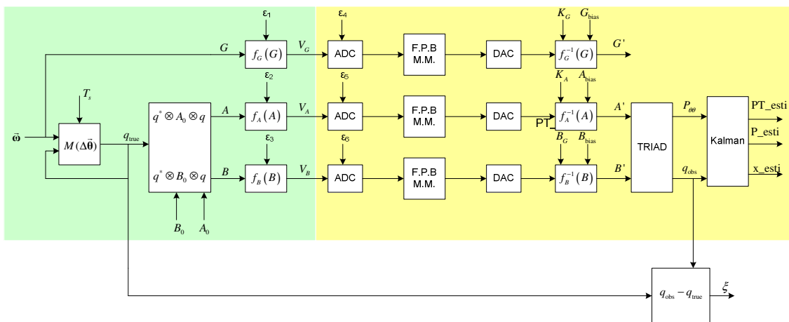
Figura 7.1 – Diagrama de blocos do simulador
