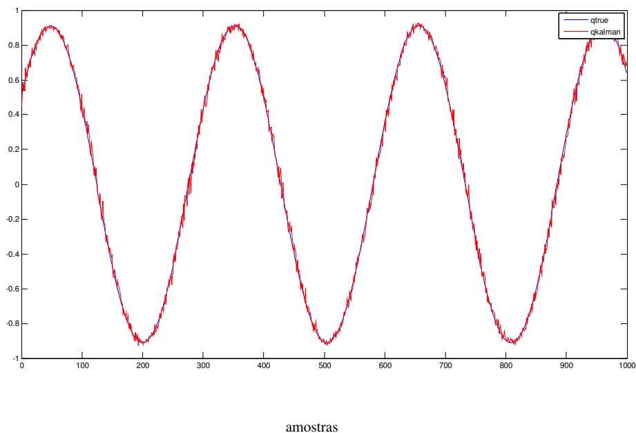
Figura 7.10 – Quatérnions simulados
