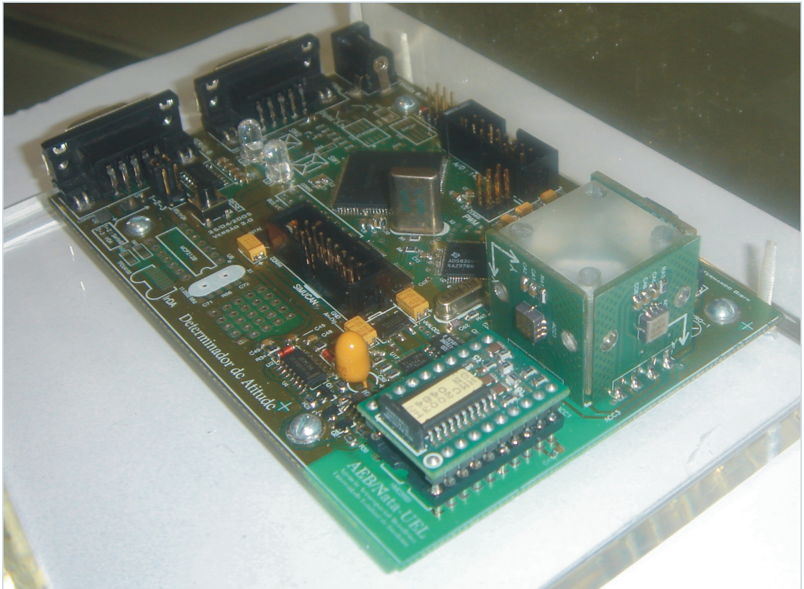
Figura 1.1 – Protótipo do determinador de atitude baseado em sensores MEMS
