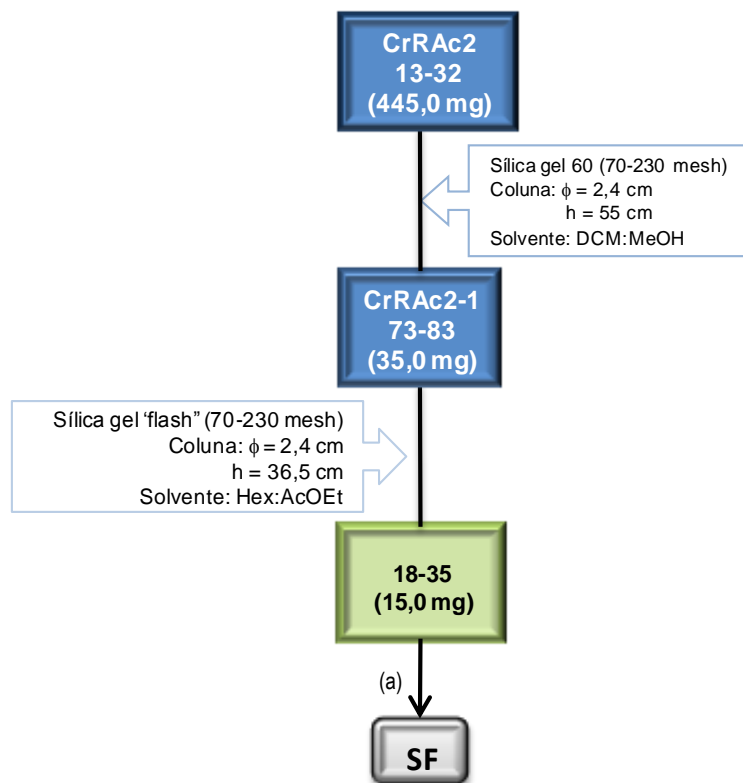
Fig. 13. Fluxograma do processo de re-fracionamento e purificação da fração acetato de etila CrRac2 e CrRac2-1 de C. regium . A cor verde identifica a fração em que houve substância cristalizada, a qual foi purificada e em seguida, recristalizada (a), formando a substância identificada como F (SF). A cor azul identifica as frações que foram recromatografadas.
