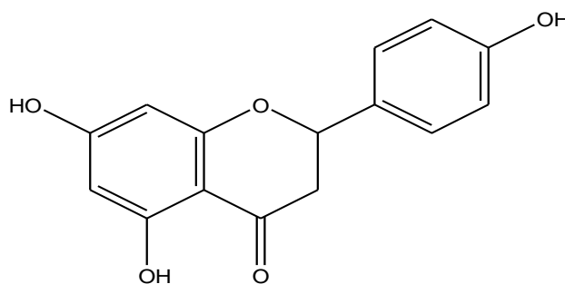
Fig. 16. Estrutura química da naringenina.
