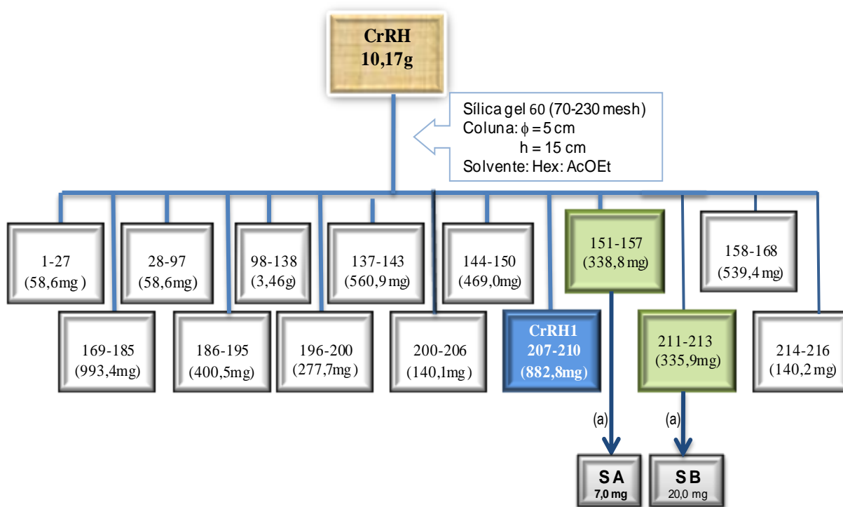
Fig. 8. Fluxograma do processo de fracionamento do extrato hexânico das raízes de C. regium . Nas frações identificadas com a cor verde houve cristalização dos compostos, que após passar por processo de purificação com MeOH (a), recristalizaram formando as substâncias A (SA) e B (SB). A fração identificada com a cor azul foi recromatografada.
