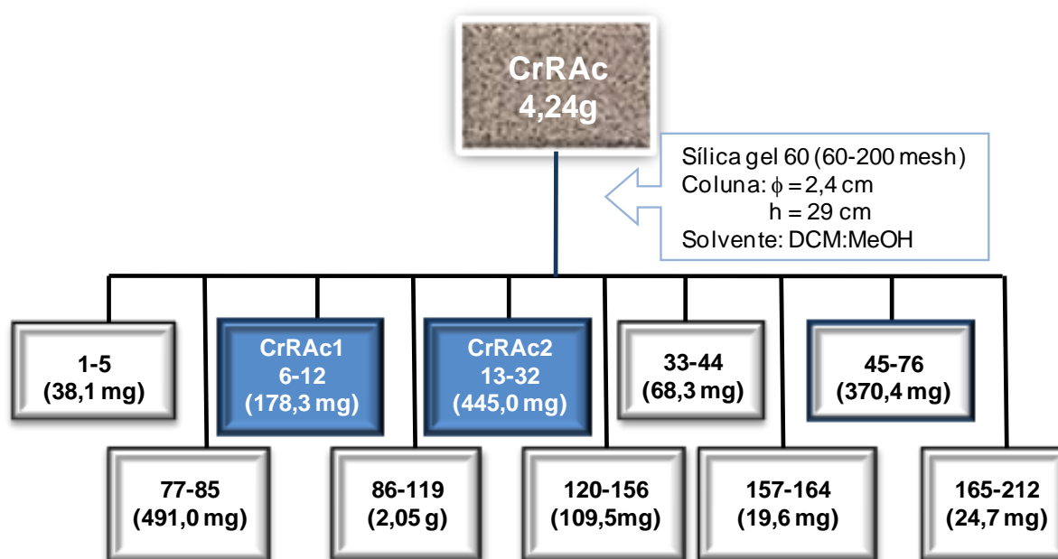
Fig. 11. Fluxograma do processo de fracionamento do extrato acetato de etila CrRAc da raiz de C. regium . As frações representadas em azul foram recromatografadas.
