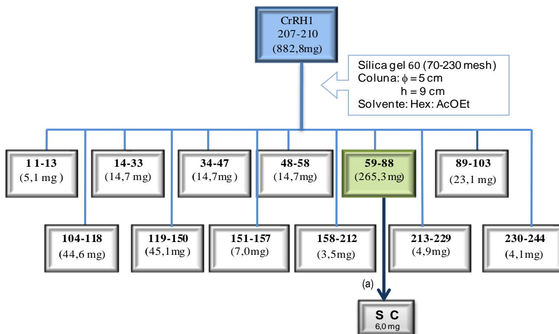
Fig. 9. Fluxograma do processo de purificação da fração hexânica CrRH1 da raiz de C. regium . A cor verde identifica as frações onde houve cristalização de compostos. (a) procedimento de purificação, com posterior recristalização resultando na formação da substância C (SC). A cor azul identifica a fração que foi recromatografada.
