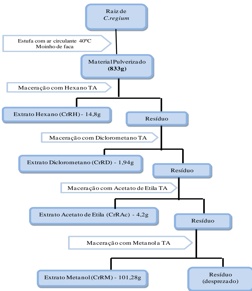
Fig. 7. Fluxograma geral de obtenção dos extratos da raiz de C. regium .
