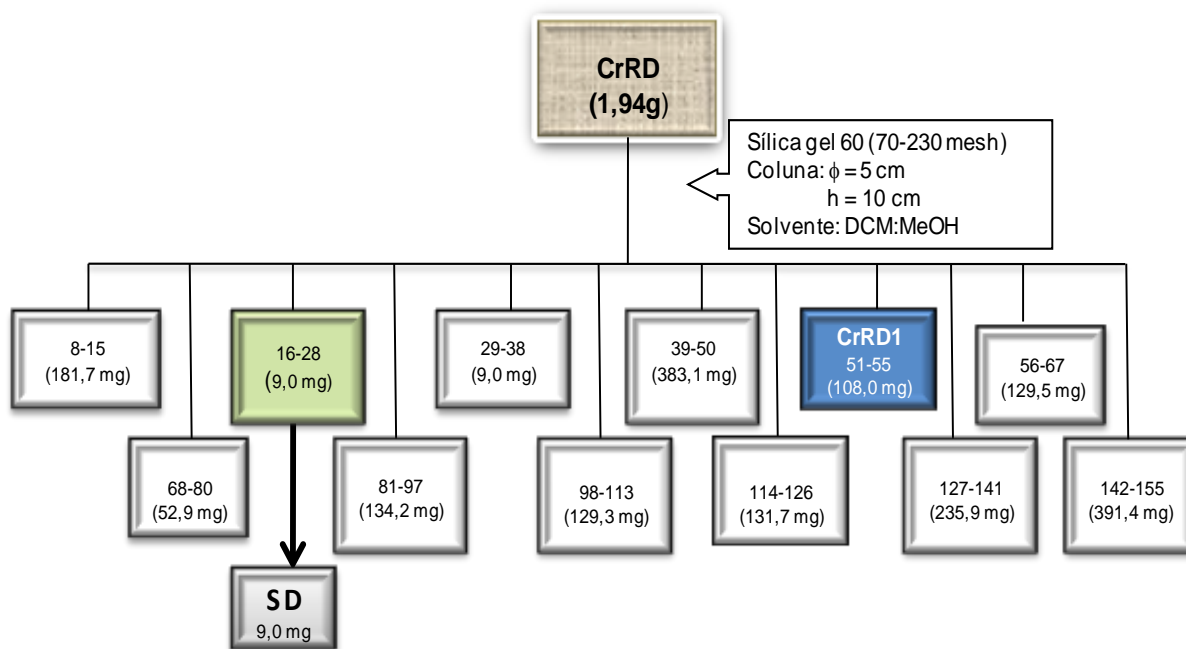
Fig. 10. Fluxograma do processo de fracionamento do extrato diclorometânico das raízes de C. regium . Nas frações representadas em verde, compostos foram cristalizados. Estes foram purificados e recrystalizados (a) formando a substância D (SD). A fração identificada com a cor azul foi submetida à nova cromatografia.
