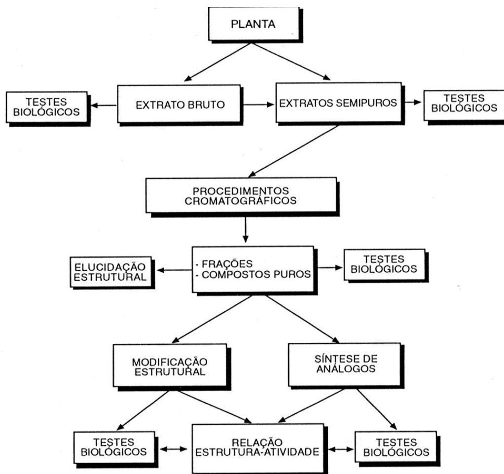
Fig.1. Procedimentos gerais para a obtenção de compostos biologicamente ativos. Fonte: Cechinel Filho e Yunes (2001)
