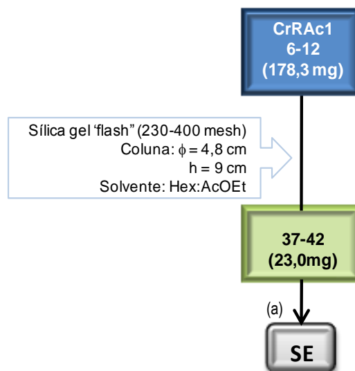
Fig. 12. Fluxograma do processo de re-fractionamento e purificação da fração acetato de etila CrRAc1 de C. regium . A cor verde identifica a fração em que houve substância cristalizada, que passou pelos processos de purificação e recristalização (a), formando a substância E (SE). A cor azul identifica a fração que foi recromatografada.
