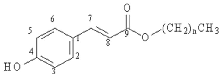
Fig. 15. Estrutura química do ácido p-hidroxicinâmico esterificado
