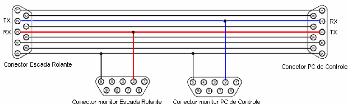
Figura 30 - Esquema de pinagem do cabo derivador
