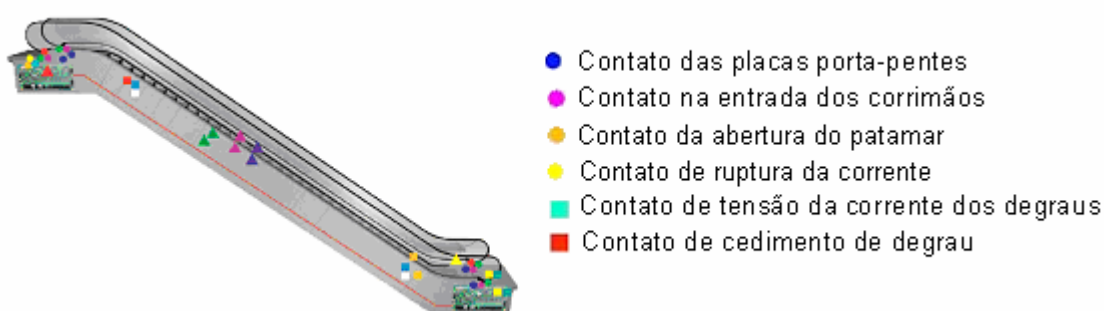
Figura 6 – Pontos de segurança
