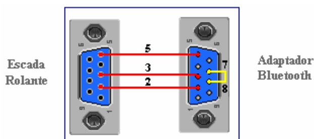
Figura 25 - Esquema de ligação do adaptador controle de fluxo
