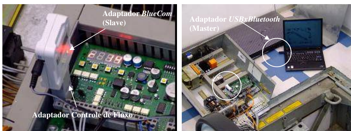
Figura 33 - Ligação dos adaptadores na placa de comando e no terminal
