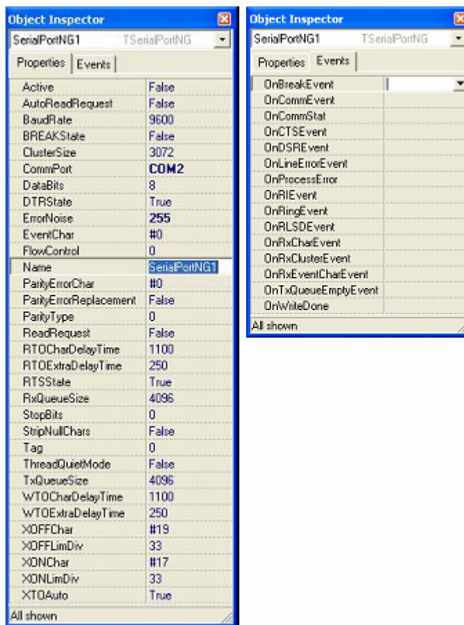
Figura 26 - Componente TSerialNG
