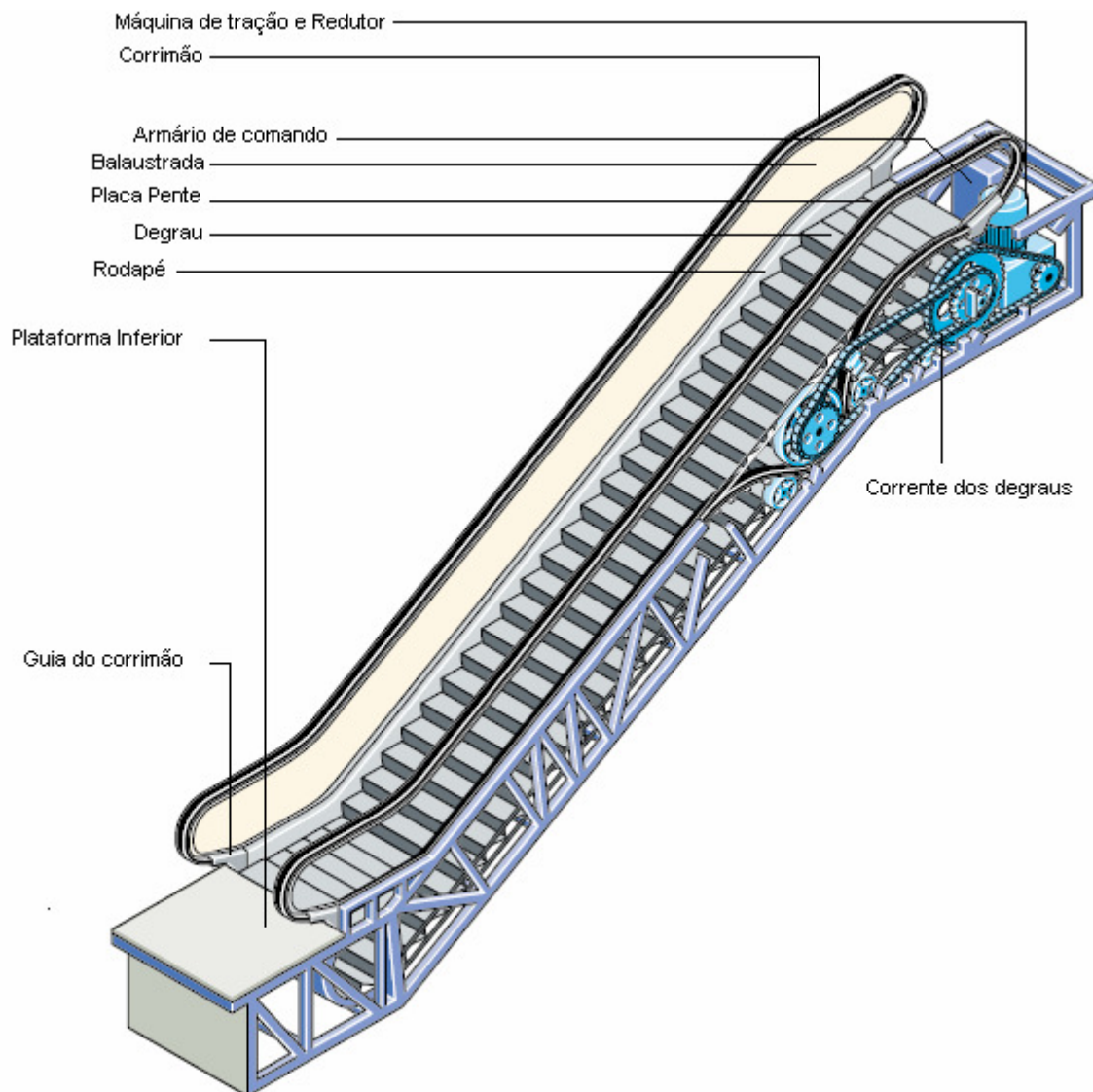
Figura 1 - Escada Rolante
