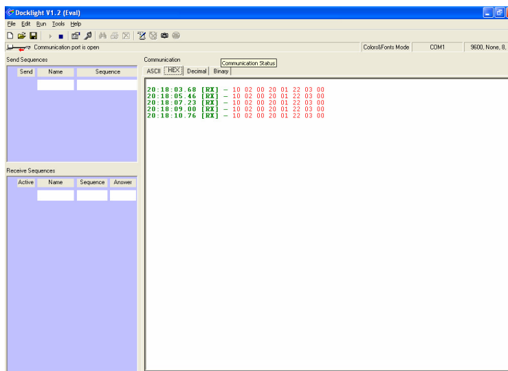
Figura 28 - Conexão entre a placa de comando da escada rolante e o software analisador de protocolos
