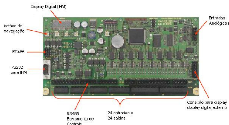
Figura 11– Comando Eletrônico da Escada Rolante
