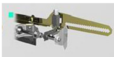
Figura 8 – Contato de tensão da corrente dos degraus
