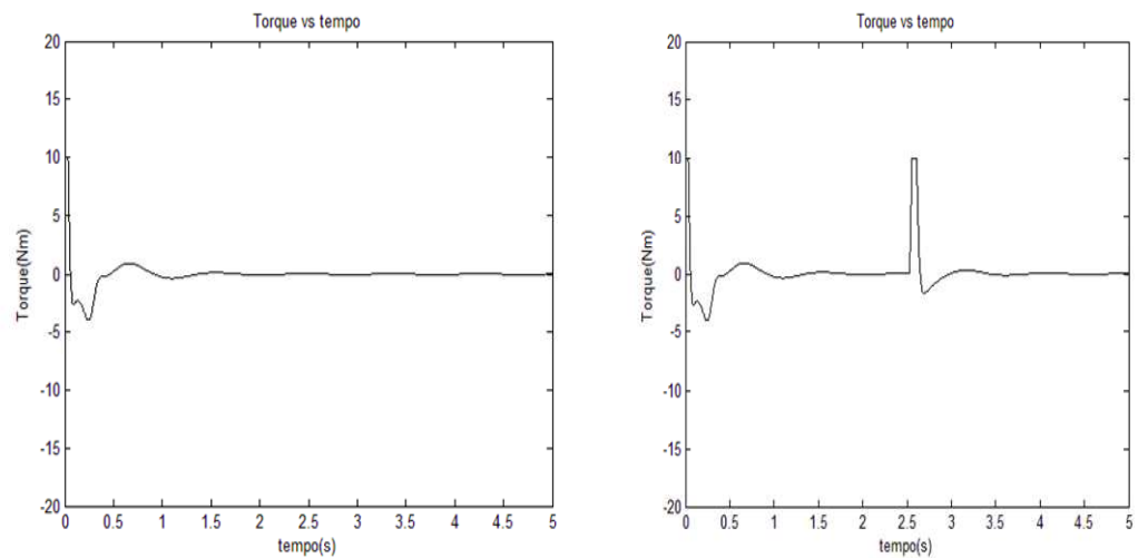
d. Variações de torque com perturbação
