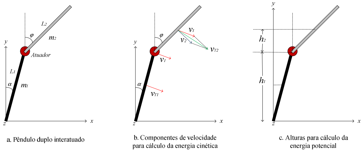
Figura 4.3- Parâmetros para o cálculo das equações de movimento do pêndulo duplo invertido interatuado.
