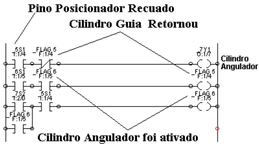
Figura 48 Programa em Ladder do cilindro angulador
