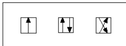
Figura 13 Direção de fluxo das Válvulas Direcionais
