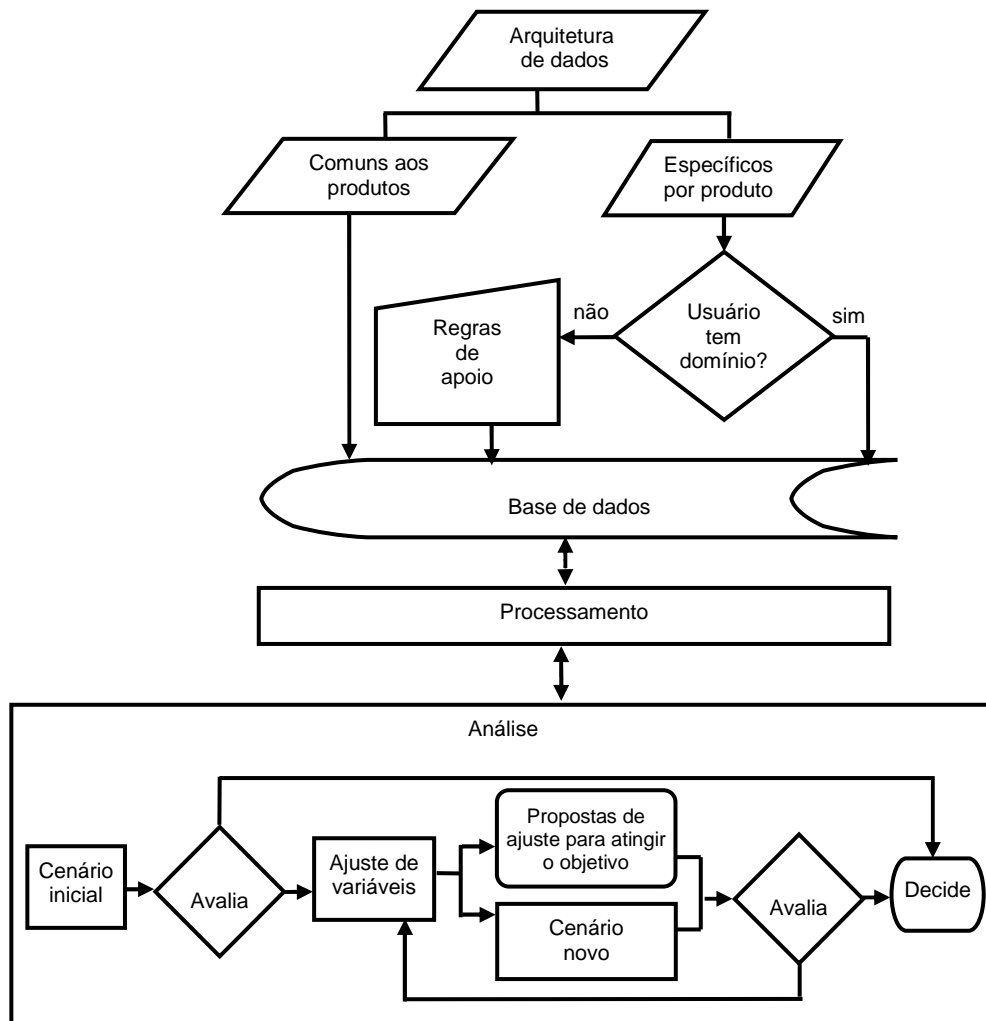
Figura 4: Modelo do processo decisório implementado no Sadedc
