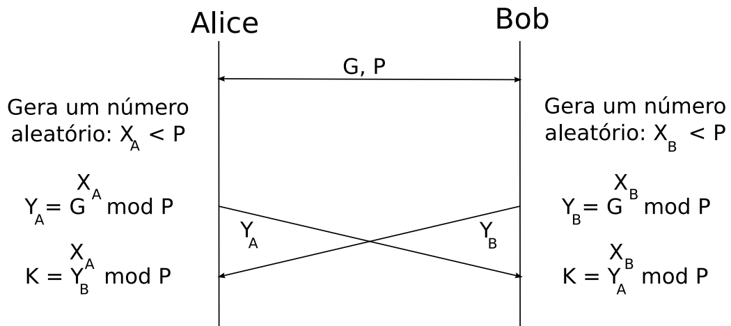
Figura 4.3: Acordo de chaves Diffie-Hellman.
