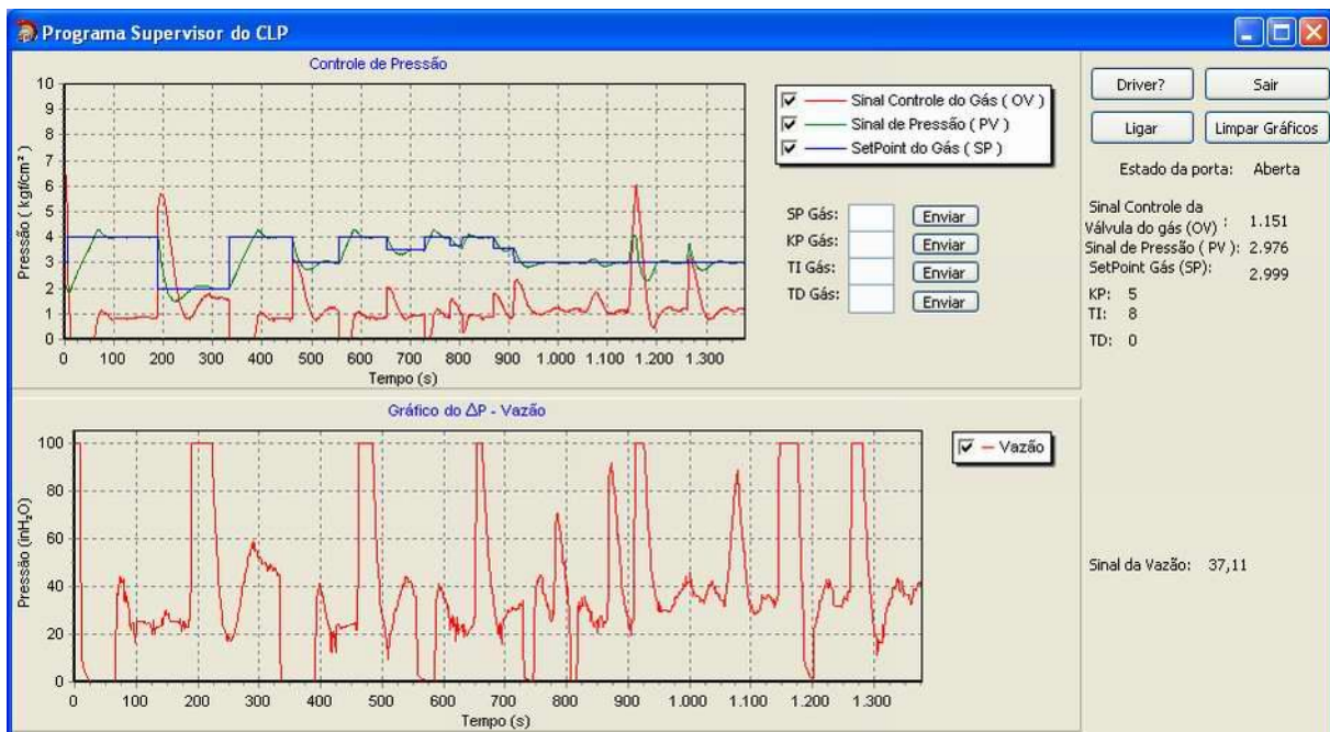
Figura 5.5-1 – Controle de pressão e medição de vazão
