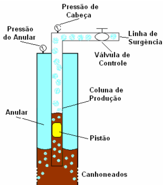
Figura 2.2.2-2 – 2ª. Etapa do ciclo: abertura da válvula de controle na superfície
