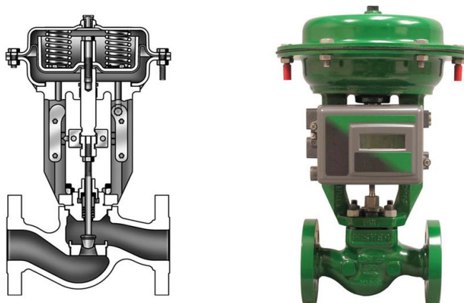
Figura 2.5.2-1 – Válvula de controle convencional
