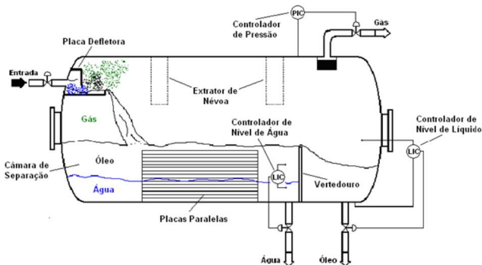
Figura 2.4.3-1 – Separador Trifásico
