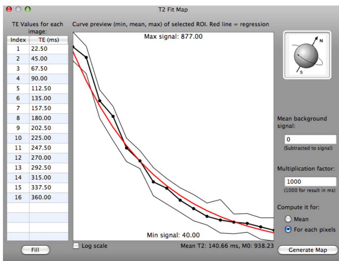
Figura 7. Curva exponencial dos valores de T2 obtidos na Relaxometria.
