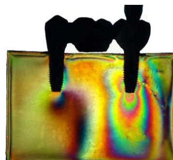
Fig. 15 - Aplicação de carga axial no molar -HI- Prótese Parafusada.
