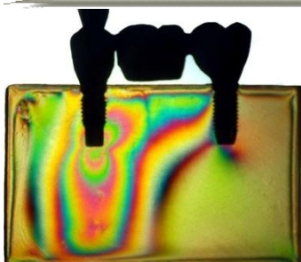
Fig. 16 – Aplicação de carga axial no pré-molar -HE- Prótese Parafusada.
