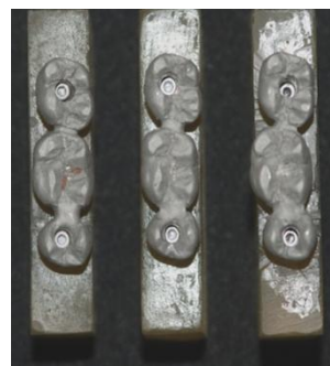
Fig. 8- Coroas metálicas múltiplas nos modelos fotoelásticos.
