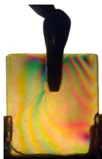
Fig. 14- Modelo unitário –HI-parafusada - carga oblíqua.
