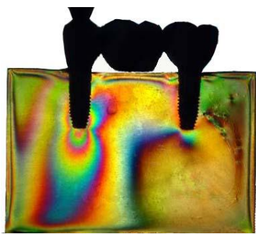
Fig. 13 – Aplicação de carga axial no pré-molar -HI- Prótese Parafusada.
