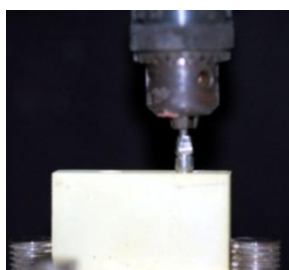
Fig. 4 – Instalação do conjunto transferente quadrado e análogo do implante com auxílio do delineador.
