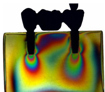
Fig. 21 – Aplicação de carga axial no molar -CM- Prótese Parafusa.
