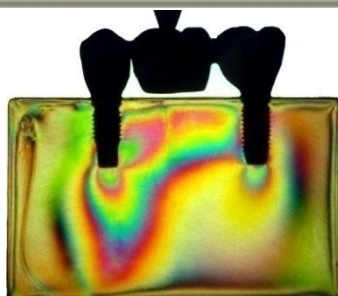
Fig. 17 - Aplicação de carga axial no pântico -HE- Prótese Parafusada.
