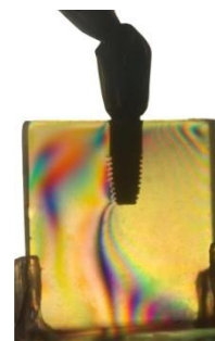
Fig. 15- Modelo unitário –CM-parafusada - carga oblíqua.
