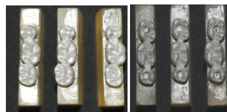
Fig. 22 - Coroas no modelo fotoelástico
