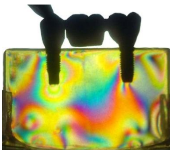
Fig. 19 – Aplicação de carga oblíqua no pré- molar -HE- Prótese Parafusada.
