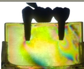
Fig. 26 - Aplicação de carga oblíqua no pântico - HI - Prótese Parafusada.
