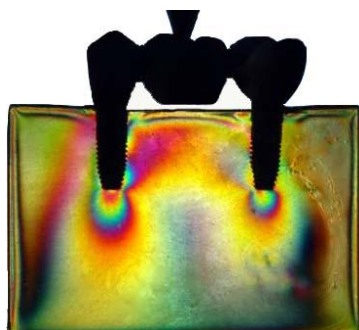
Fig. 14 - Aplicação de carga axial no pântico -HI- Prótese Parafusada.
