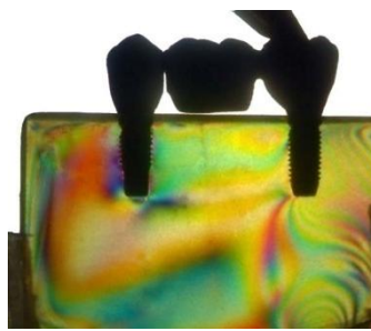
Fig. 21 – Aplicação de carga oblíqua no molar -HE- Prótese Parafusada.
