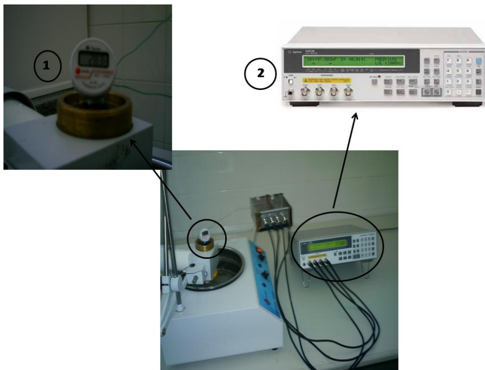
Figura 3.5: Aparato experimental para as medições de impedância das emulsões em frequências pontuais.
