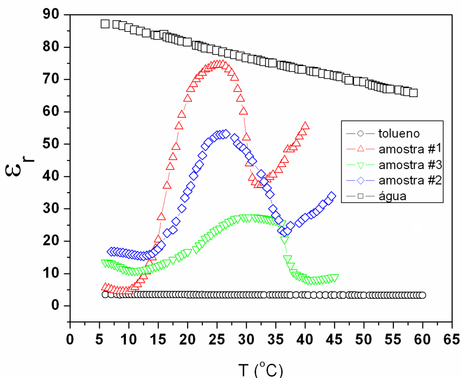
Figura 5.14: Permissividade relativa para cada amostra em função da temperatura na frequência de 100 kHz.
