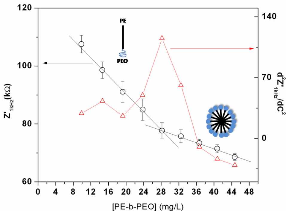
Figura 4.1: Parte real da impedância ( Z' ) em 1kHz versus concentração do copolímero em bloco 50%PEO e a segunda derivada de Z' como função da concentração (condição de Phillips).
