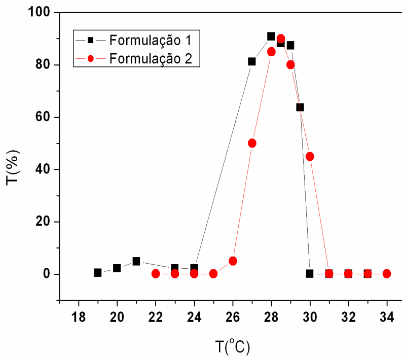
Figura 5.22: Varredura da transmitância da emulsão como função da temperatura para duas formulações a 700nm (comprimento de onda).
