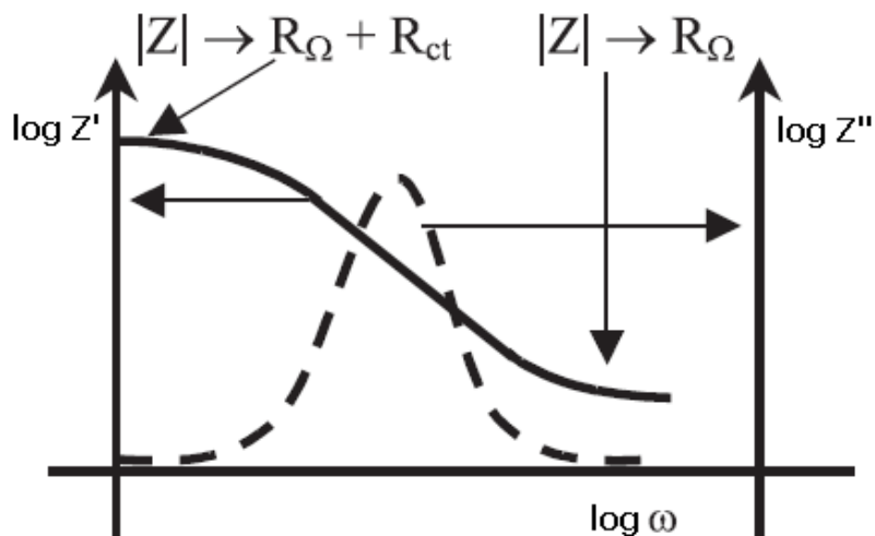
Figura 3.3: Curvas de Bode para Z' e Z'' em função da frequência.
