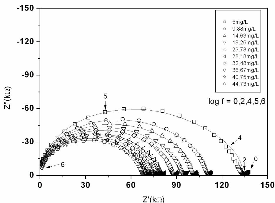
Fig. 4.3 Diagramas de Nyquist que determinam a CMC do PE-b-PEO.
