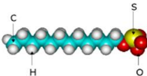
Figura 1.1: Estrutura de uma molécula anfifílica [2].
