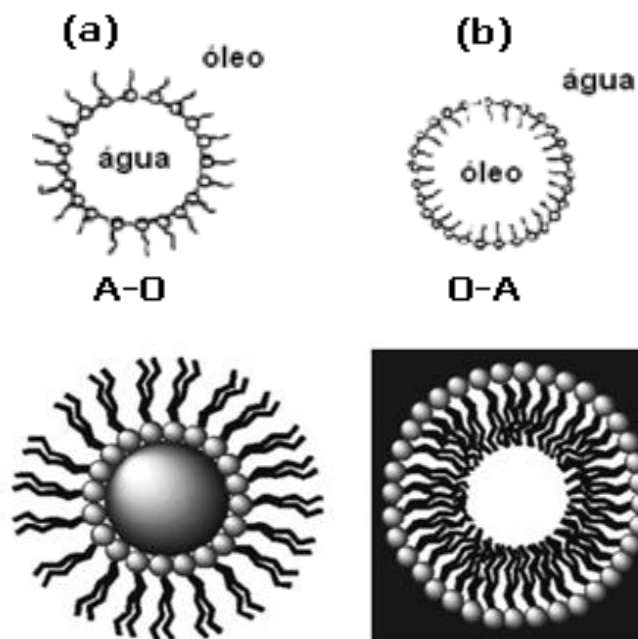
Figura 1.7: (a) Gotículas inversas (fase A-O) e (b) gotículas diretas (fase O-A) [3].
