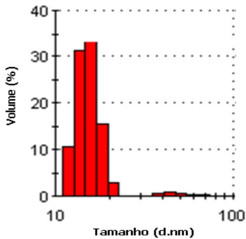
Figura 5.3: Análise de tamanho de partícula para a formulação (40-40-20).
