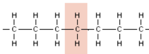
Figura 1.8: Representação esquemática de uma cadeia polimérica. Em destaque, o monômero que dá origem a essa molécula [28].
