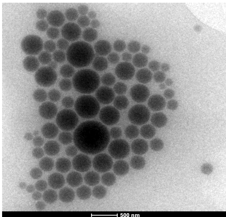
Figura 5.5: Imagens obtidas por TEM para a microemulsão à 25°C.
