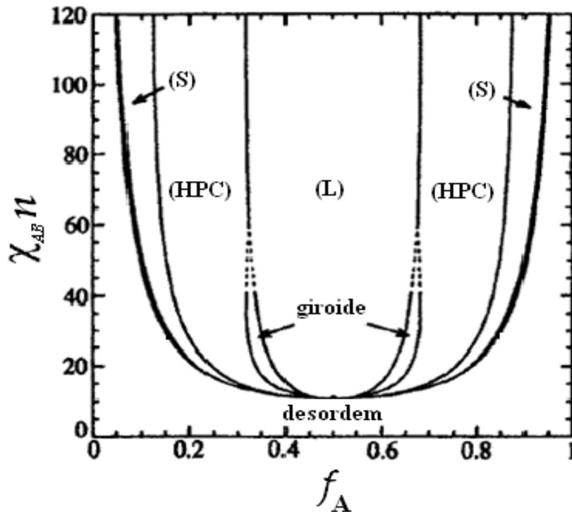
Figura 1.14: Diagrama de fases \chi_{AB}n versus f_A para copolímeros dibloco [29].
