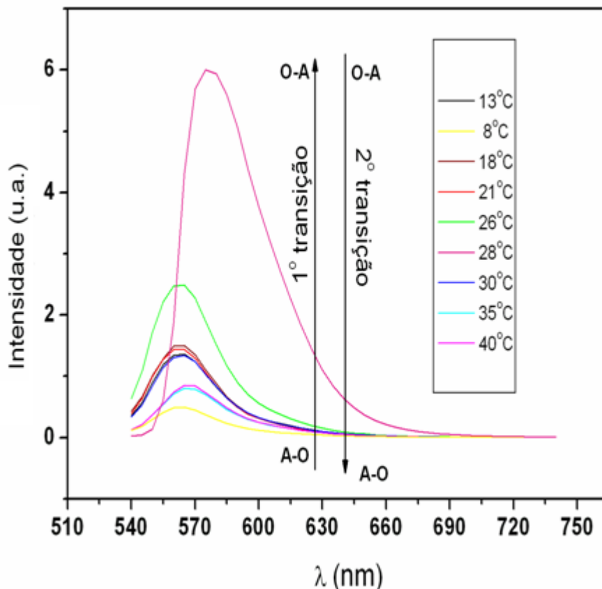
Figura 5.18: Espectro de fluorescência da Rodamina 6G ( 10^{-4}\text{M} ) na interação com a microemulsão, variando a temperatura do sistema.
