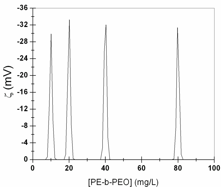
Figura 4.8: Valores de potencial Zeta para os sistemas para as concentrações de 10, 20, 40 e 80 mg/L de 50%PEO.
