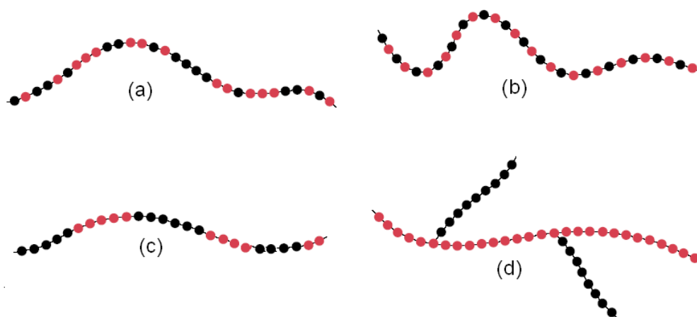
Figura 1.12: Tipos de copolímeros. (a) randômico, (b) alternante, (c) em bloco e (d) grafitizado. Círculos pretos representam os monômeros do tipo A e os vermelhos, os do tipo B [28].
