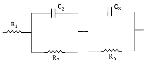
Figura 4.2: Associação em série entre um resistor R_1 e dois circuitos RC ( R_2C_2 e R_3C_3 ) paralelo.
