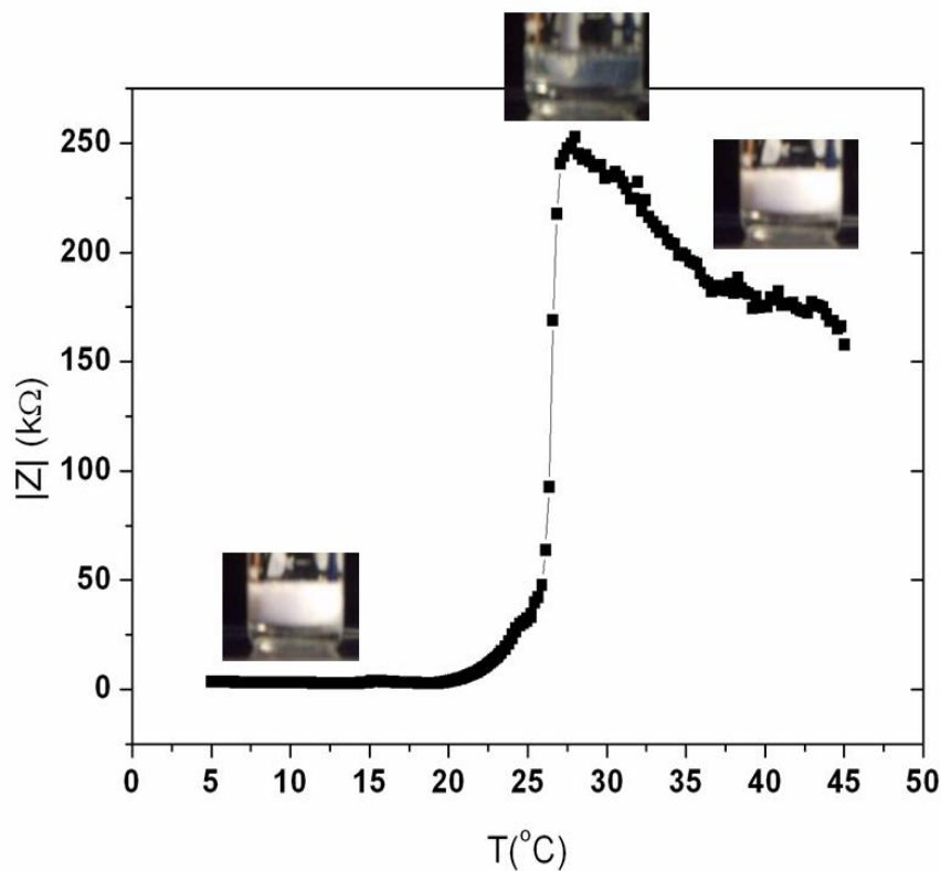
Figura 5.21 Análise elétrica da microemulsão proposta ao SACI. As inversões de fase são acompanhadas da mudança de coloração.
