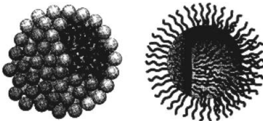
Figura 1.3: Da esquerda para a direita: micelas esféricas diretas e micelas invertidas [3].
