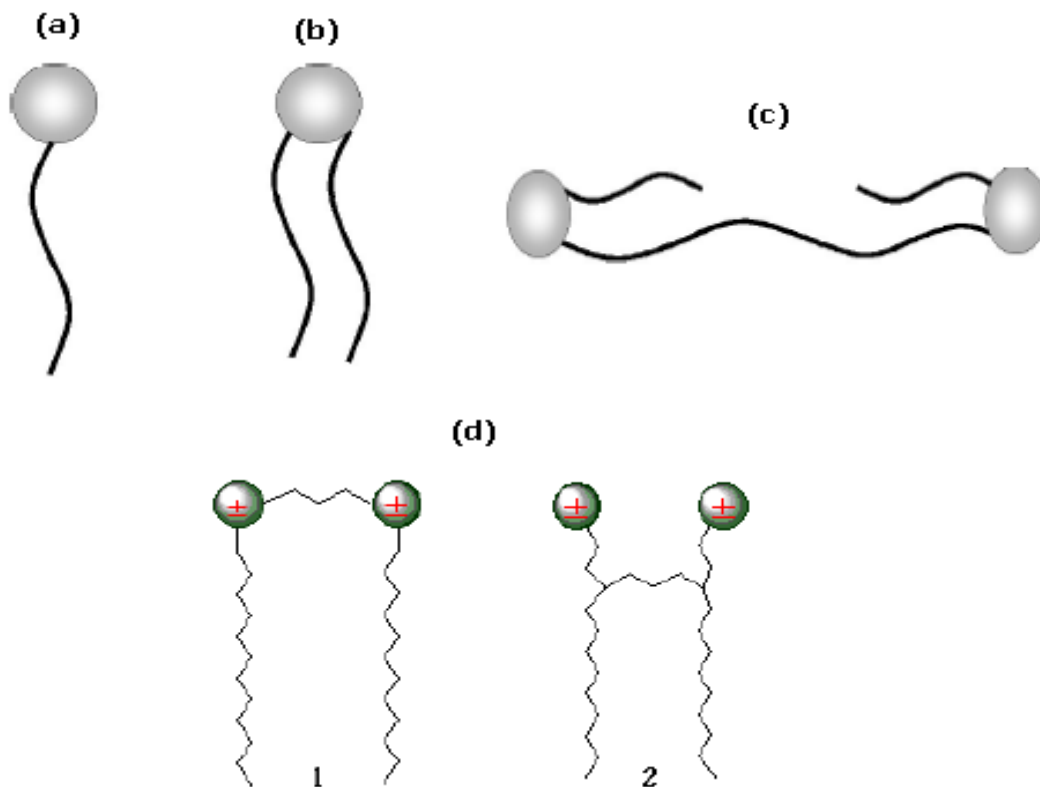
Figura 1.5: (a) Monômero de um surfactante com calda simples e (b) calda dupla. Em (c), um surfactante do tipo bolaform e em (d), dois surfactante do tipo gemini [2].
