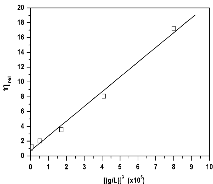
Figura 4.11: Ajuste linear da viscosidade relativa com a terceira potência da concentração para dispersões do copolímero em bloco na faixa de 8% a 24% em massa.
