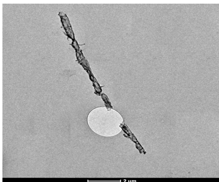
Figura 4.7: Estrutura das micelas do tipo ‘charuto’ em uma concentração de 80mg/L de 50%PEO.
