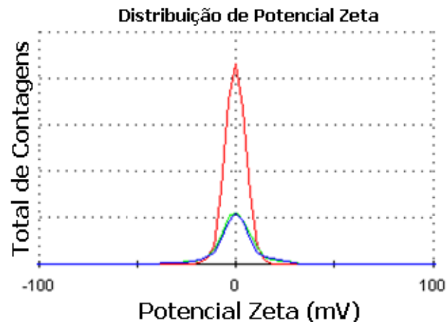
Figura 5.7: Distribuição do potencial Zeta para a amostra (40-40-20).
