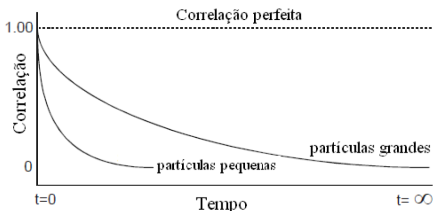
Figura 3.11: Função de correlação para partículas grandes e pequenas.
