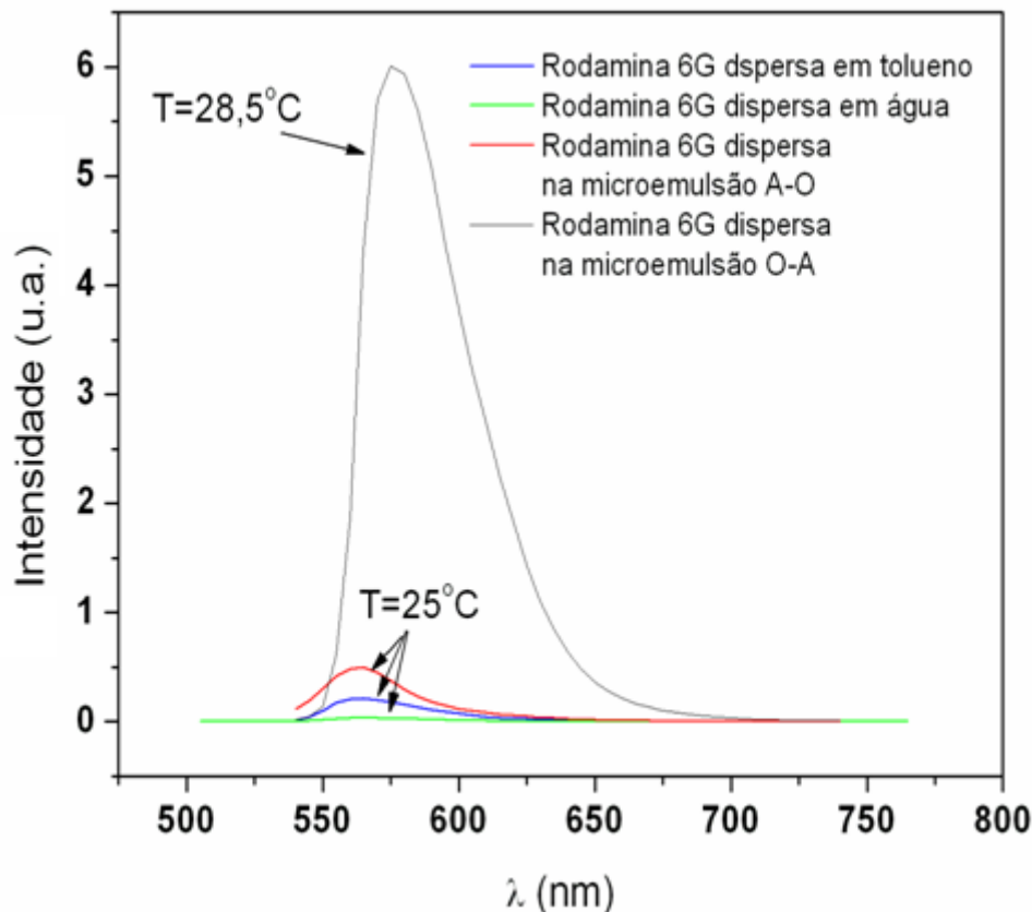
Figura 5.17: Variações no espectro de fluorescência para diferentes meios.
