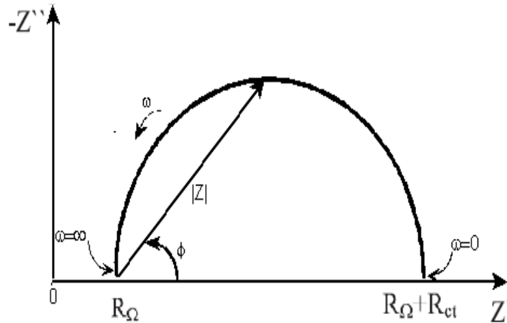
Figura 3.2: Diagrama de Nyquist.
