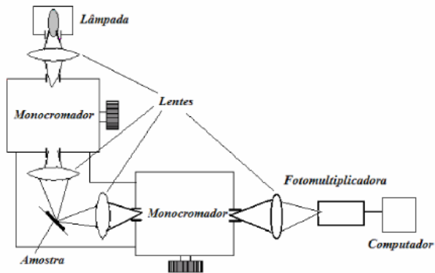
Figura 3.12: Princípio de funcionamento do espectrofluorímetro ISS PC1.
