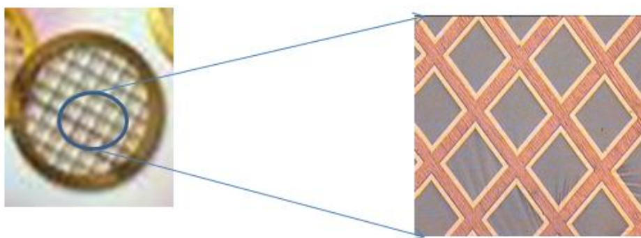
Figura 3.7: Porta-amostra para as medições de TEM. Em destaque, a grade concatenada de cobre (em vermelho) recoberta por um filme de carbono (em cinza).
