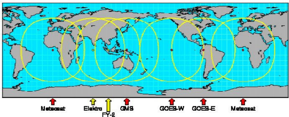
Figura 2.3 – Áreas observadas por alguns satélites geoestacionários (SOKOLIK, 2002).
