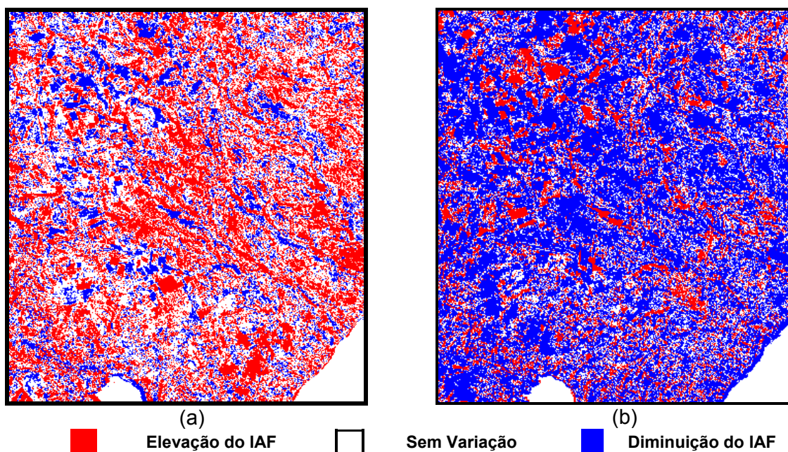
Figuras 4.26 – Imagens classificadas da subtração do IAF estimado: (a) entre o dia 11/06/1990 e o de 21/09/1998 e (b) entre o de 21/09/1998 e o dia 03/09/2003.
