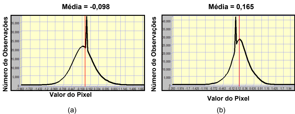
Figuras 4.25 – Histogramas de freqüência das imagens de subtração do IAF estimado entre os dias 11/06/1990 e 21/0/1998 (a) e 21/09/1998 e 03/09/2003 (b).
