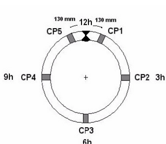
Figura 3.1 – Regiões marcadas na direção circunferencial do tubo.
