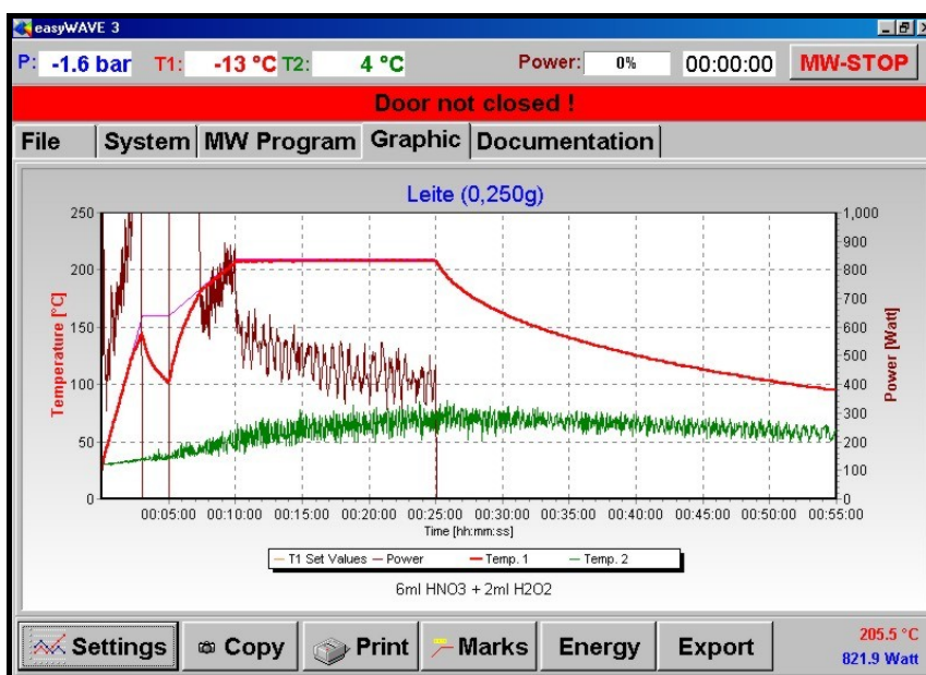
Figura 3.22 Curva de digestão característica gerada pelo aplicativo destinado à programação do tempo, temperatura e potência do forno de microondas Milestone ETHOS 1600
