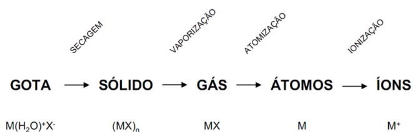
Figura 2.4 Esquema de ionização de amostras realizado pelo plasma
