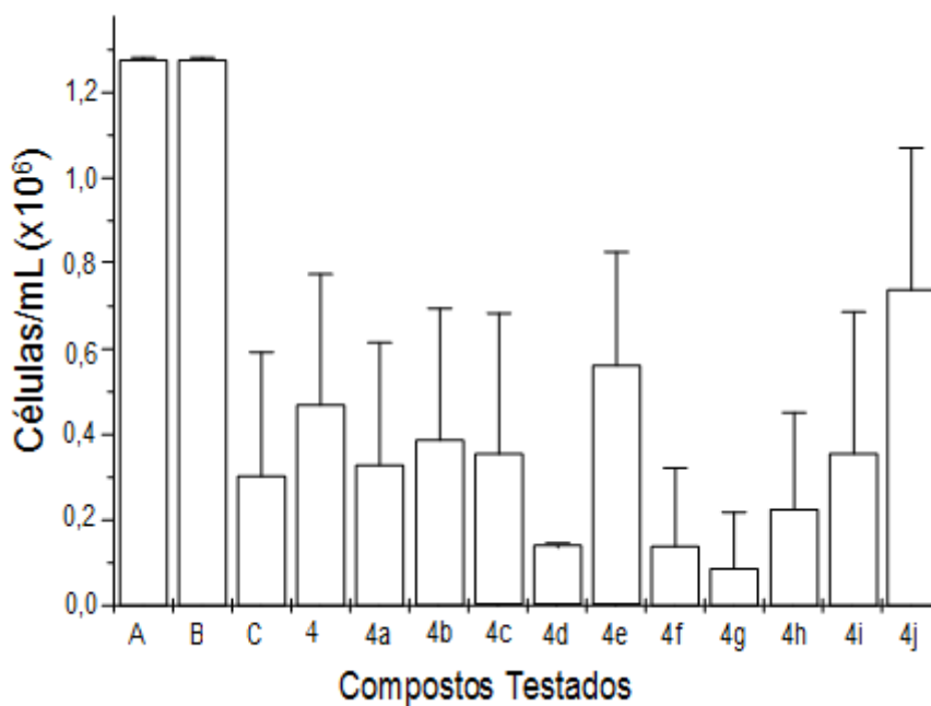
Figura 25. Efeito dos derivados tieno-piridina [50 \mu M] na proliferação de parasitas na forma promastigota da espécie Leishmania amazonensis após 24 horas de incubação. A = Controle; B = DMSO; C = Glucantime ; 4 = H; 4a = m -CH 3 ; 4b = m -OCH 3 ; 4c = m -NO 2 ; 4d = m -F ; 4e = m -Br; 4f = p -CH 3 ; 4g = p -OCH 3 ; 4h = p -NO 2 ; 4i = p -F, e 4j = p -Br.
