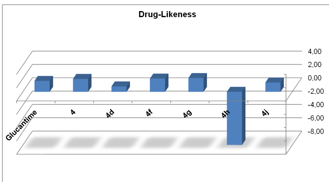
Figura 29. Drug-Likeness dos derivados mais ativos (4, 4d, 4f, 4g, 4h e 4j) comparados com o Glucantime® um fármaco comercial
