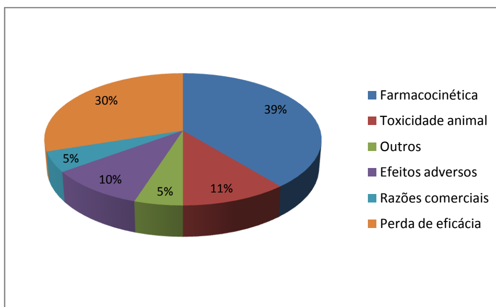
Figura 13. Principais razões do fracasso no desenvolvimento de fármacos (Adaptado de WATERBEEMD & GIFFORD, 2003)
