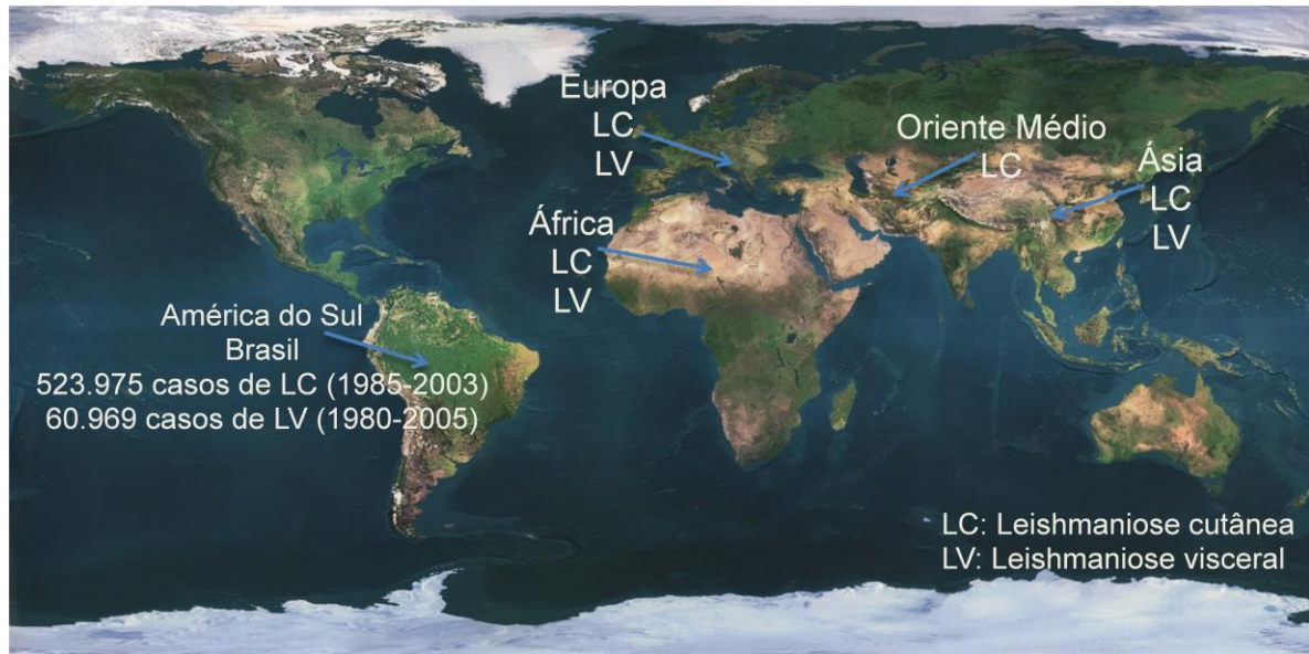
Figura 1. Distribuição mundial das duas formas de Leishmaniose (Adaptado de WHO, 2003).
