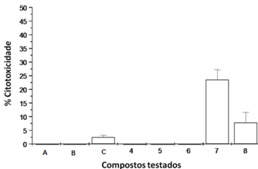
Figura 27. Efeito citotóxico dos derivados Tieno-piridinas (50 \mu\text{M} ) sobre células mononucleadas após 24 horas de incubação. A = Controle; B = DMSO ; C = Glucantime ; 4 = p -CH 3 , 5 = p -OCH 3 , 6 = p -NO 2 , 7 = m -Br e 8 = p -Br.
