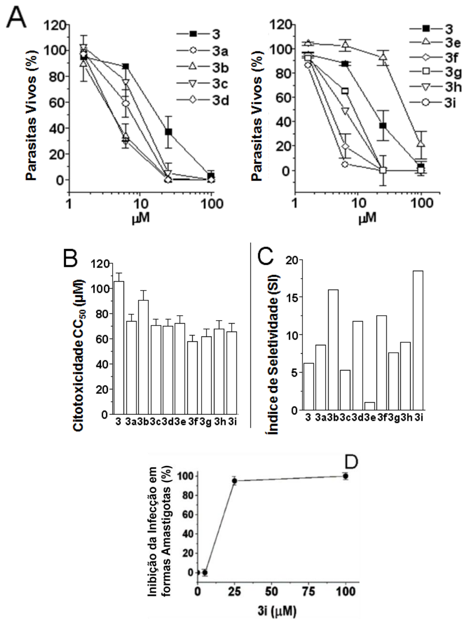
Figura 18. Avaliação Biológica dos derivados 4-metóxi-chalcona (3) e 4-metóxi-chalcona sulfonamida (3a-i). Efeito inibitório na proliferação in vitro de parasitas da espécie Leishmania braziliensis (A), perfil citotóxico em macrófagos de ratos (B), índice de seletividade (SI) calculado (C) e inibição da infecção por formas amastigotas de Leishmania braziliensis em macrófagos utilizando o composto mais ativo (3i) (D).
