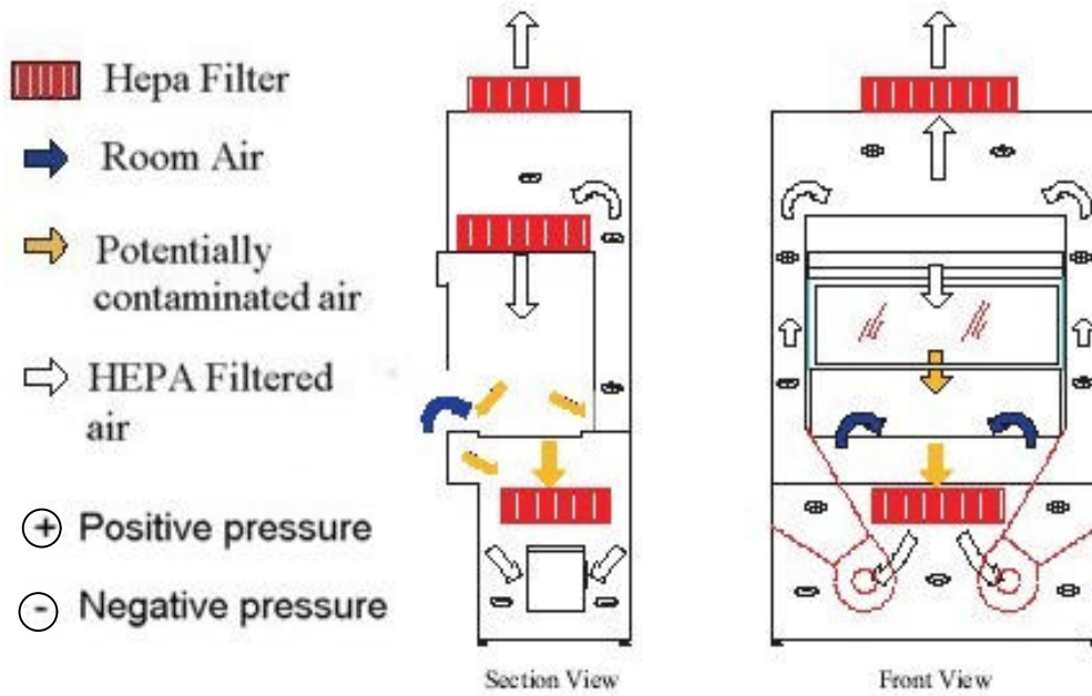
Figura 4.5 - Cabine de Biossegurança Classe II –B1
