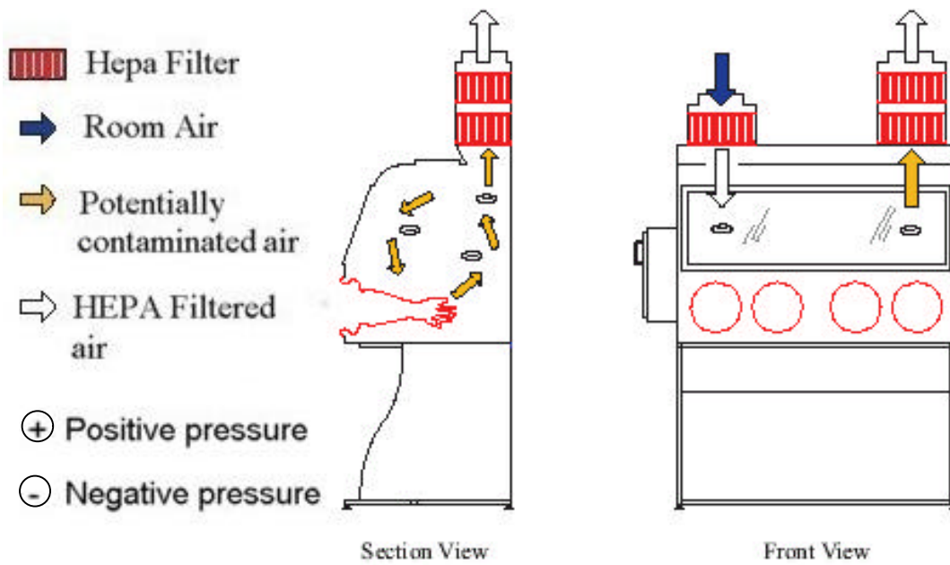
Figura 4.8 - Cabine de Biossegurança Classe III
