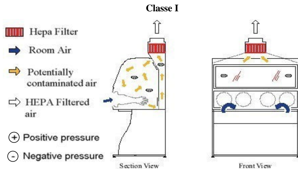
Figura 4.2 - Desenho esquemático do funcionamento da Cabine de Biossegurança Classe I
