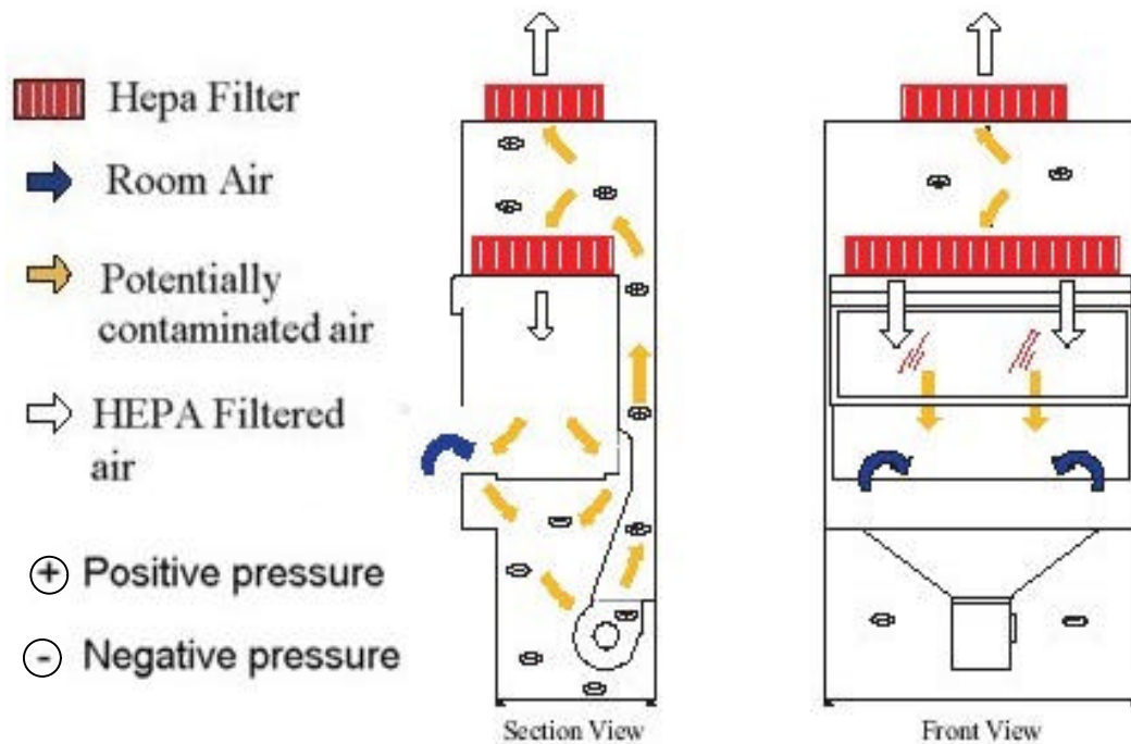
Figura 4.4 - Cabine de Biossegurança Classe II –A1
