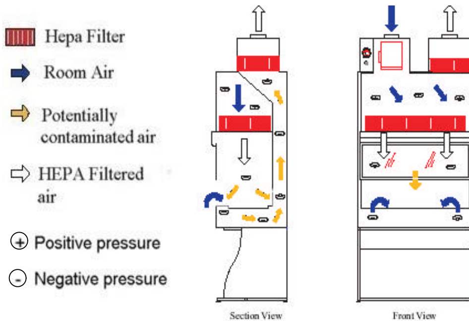
Figura 4.6 - Cabine de Biossegurança Classe II –B2
