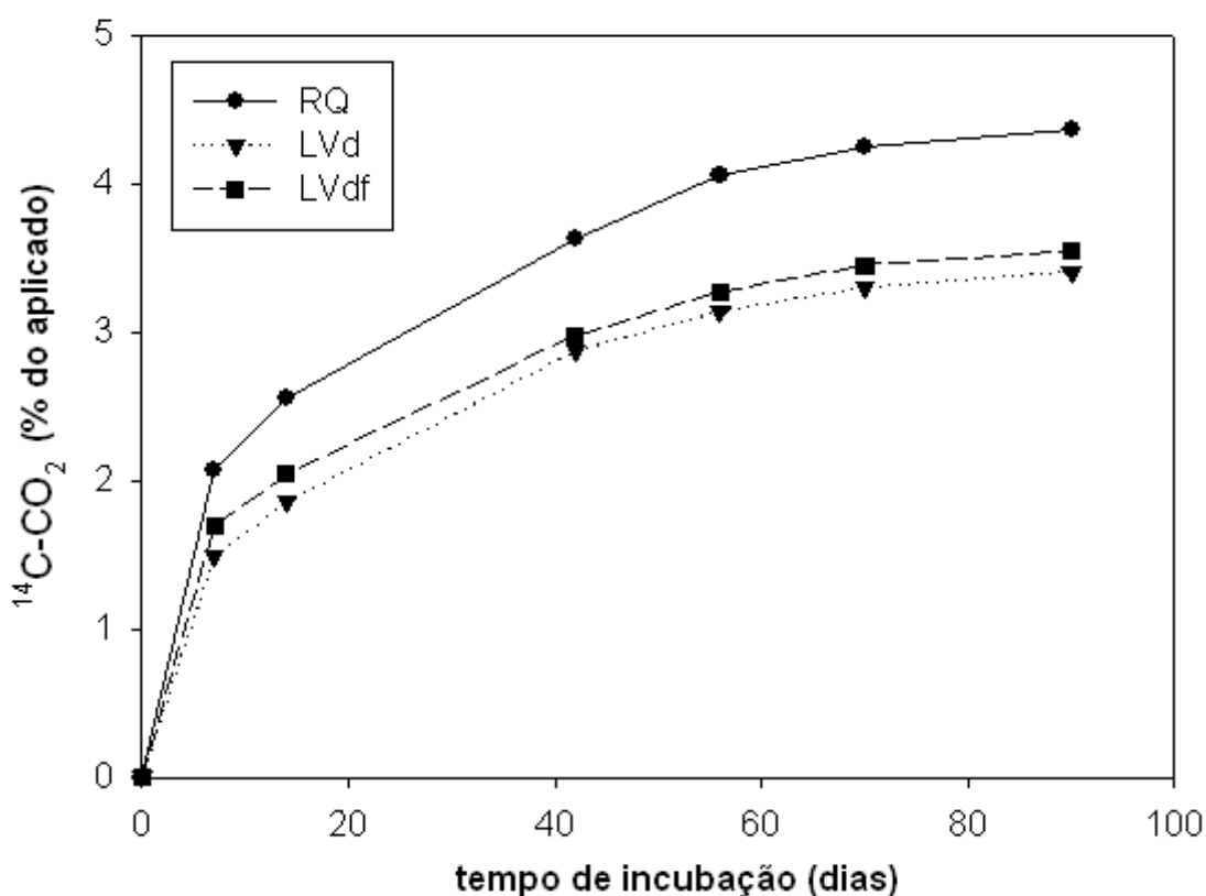
Figura 1. Porcentagem de \text{CO}_2 evoluído da aplicação de PEG-4000 em três solos do estado de São Paulo, Brasil.
