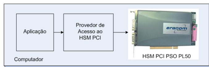
Figura 4.2: Interface de comunicação entre a aplicação e o HSM PSO PL50
