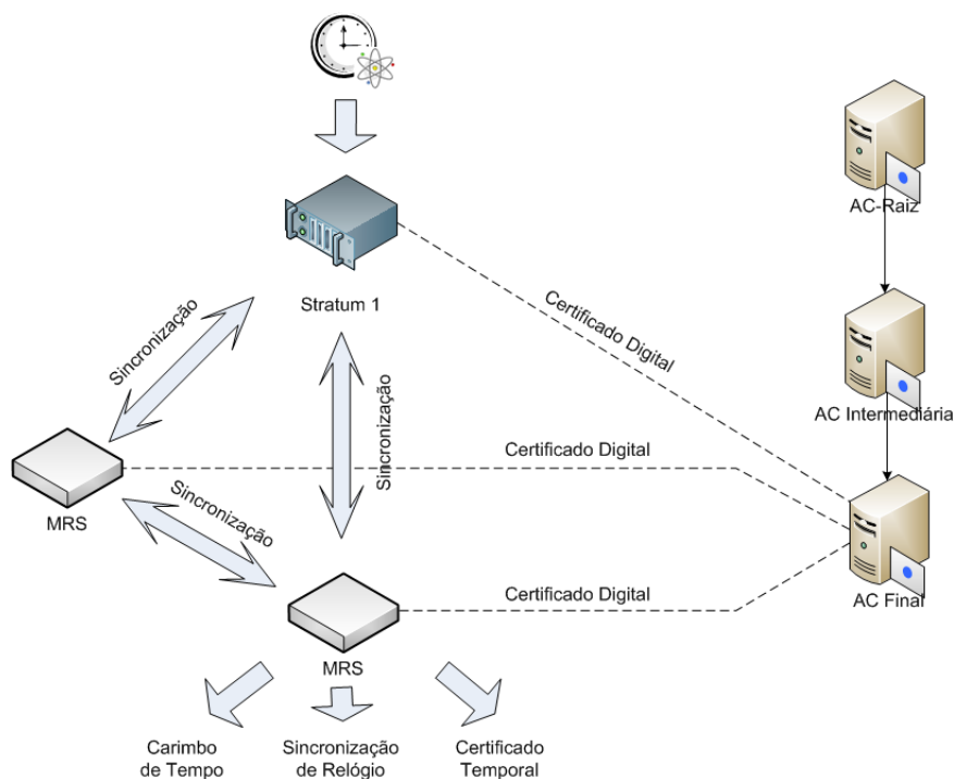
Figura 5.1: Modelo do MRS numa ICP
