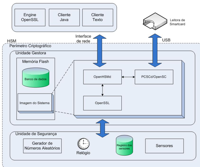
Figura A.13: Estrutura interna do ASI-HSM
