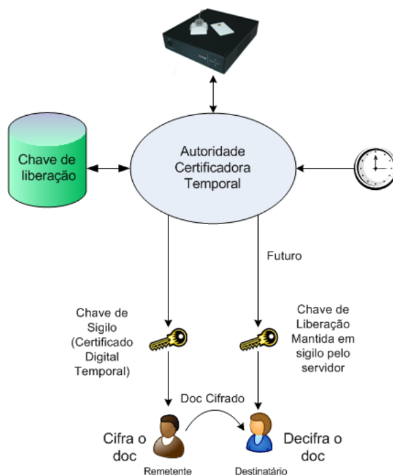
Figura 2.5: Funcionamento básico de um AC-Temporal
