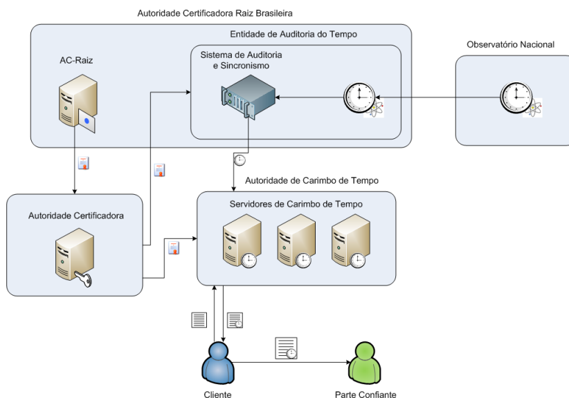
Figura 2.3: Estrutura da Rede de Carimbo de Tempo da ICP-Brasil
