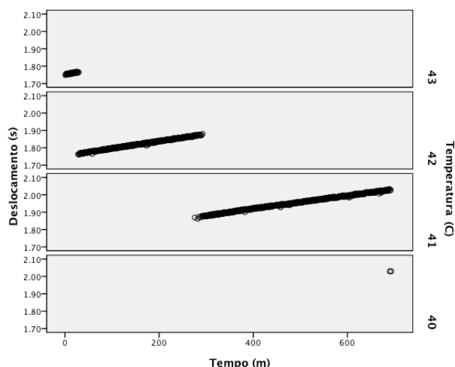
Figura A.35: Deslocamento entre o relógio do HSM e da FCT na temperatura do HSM
