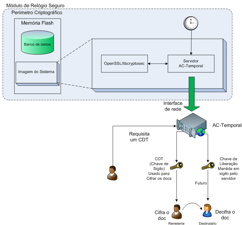
Figura 4.5: Esquema de funcionamento da Autoridade Certificadora Temporal
