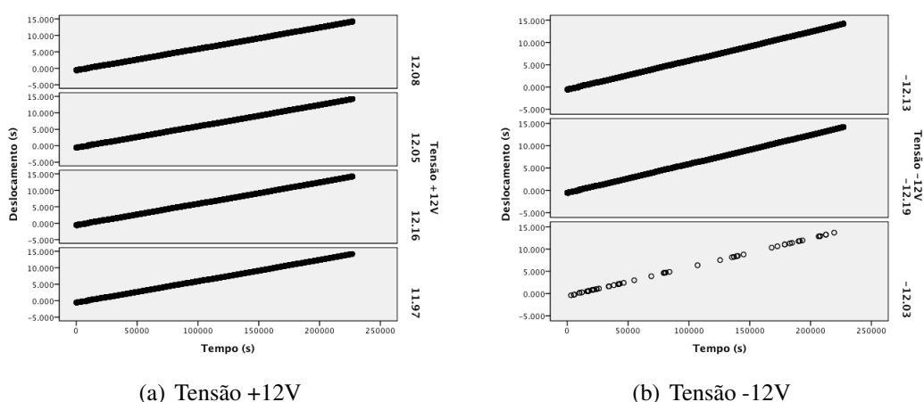
Figura A.4: Deslocamento entre o relógio do HSM e da FCT nas tensões de +12V e -12V
