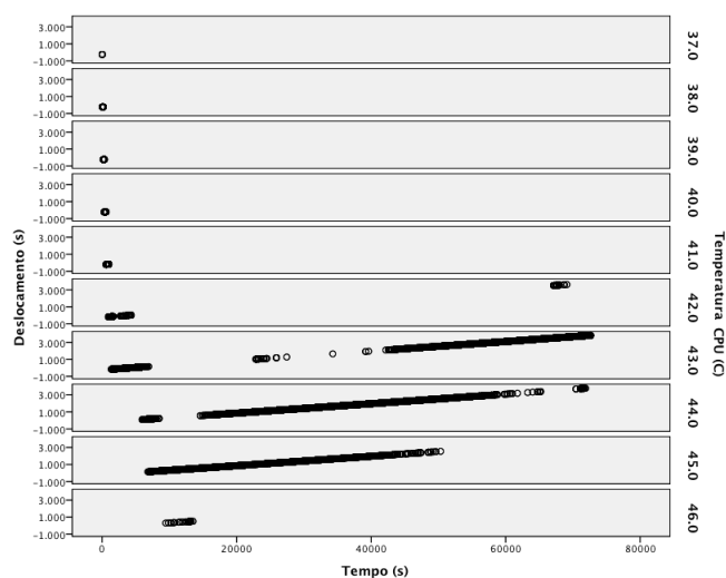
Figura A.11: Deslocamento entre o relógio do HSM e da FCT na temperatura da CPU
