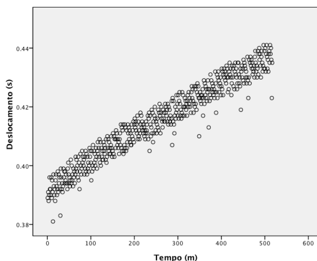
Figura A.36: Deslocamento entre o relógio do HSM e da FCT
