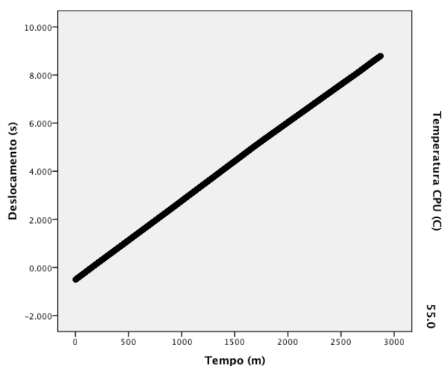
Figura A.31: Deslocamento entre o relógio do HSM e da FCT na temperatura da CPU
