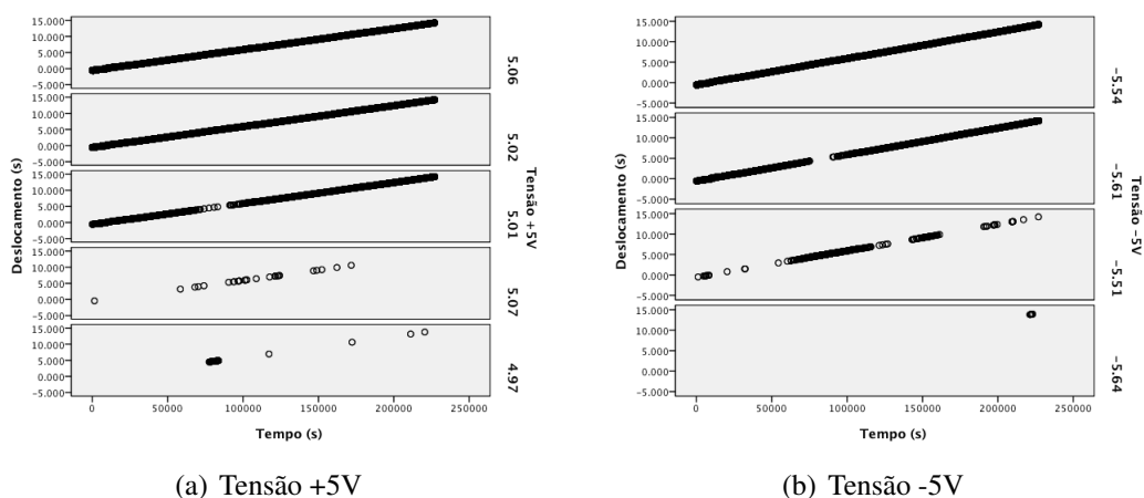
Figura A.3: Deslocamento entre o relógio do HSM e da FCT nas tensões de +5V e -5V
