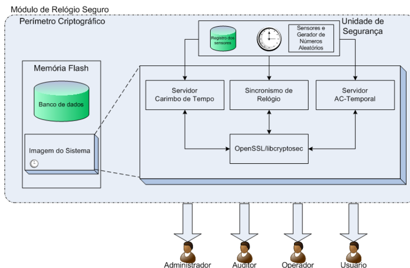
Figura 4.7: Estrutura interna do Módulo de Relógio Seguro
