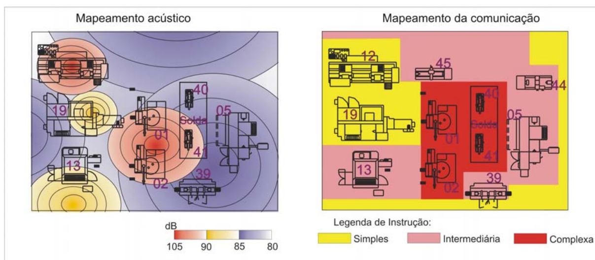
Figura 33 – Comparação do mapeamento acústico com o mapeamento de comunicação
