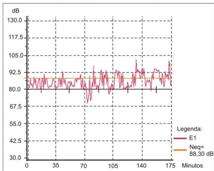
Figura 27 – Variação dos NPS para o operador no posto de trabalho E1 durante 4 horas
