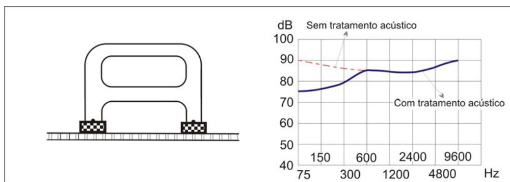
Figura 5 – Instalação de amortecedor contra vibração
