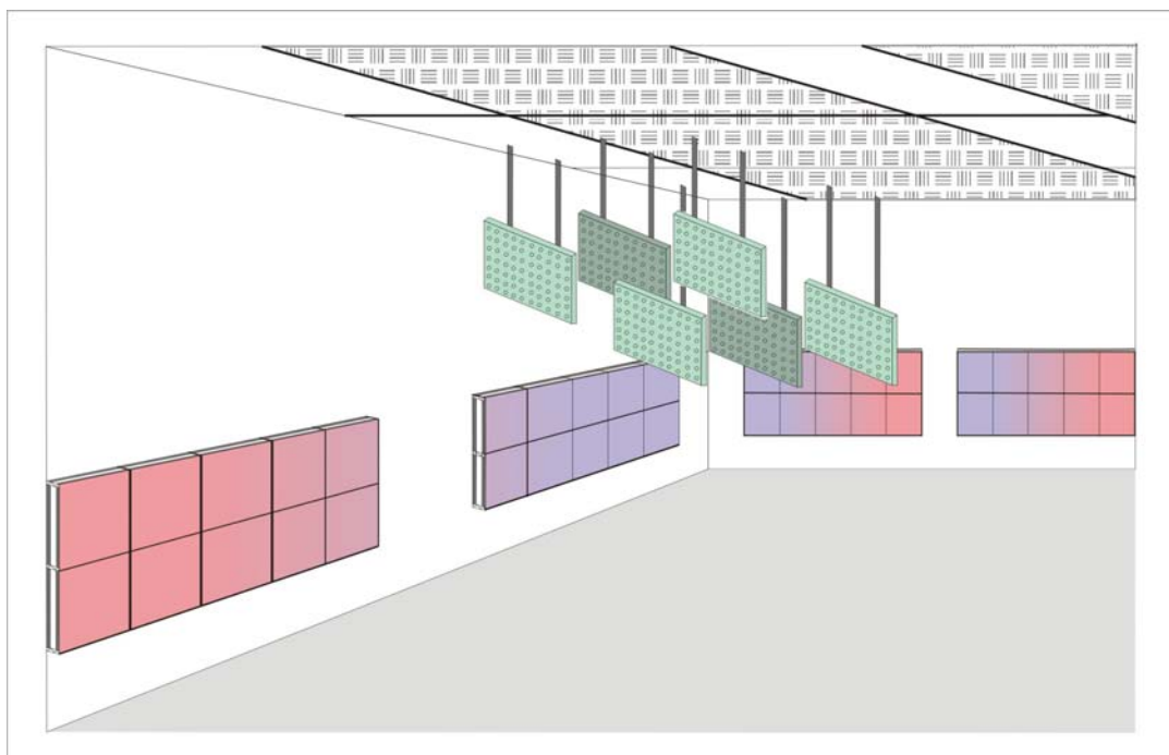
Figura 26 – Esquema dos painéis absorventes e ressonadores
