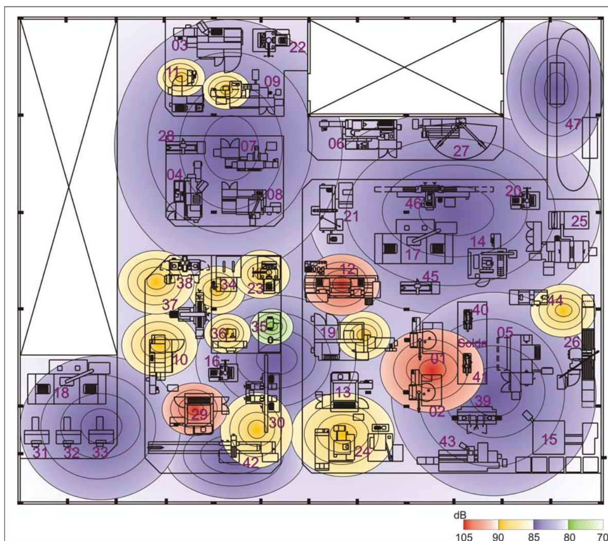
Figura 24 – Mapeamento do NPS da linha de produção
