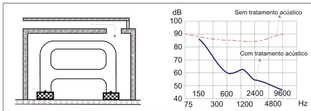
Figura 7 – Instalação de blindagem rígida
