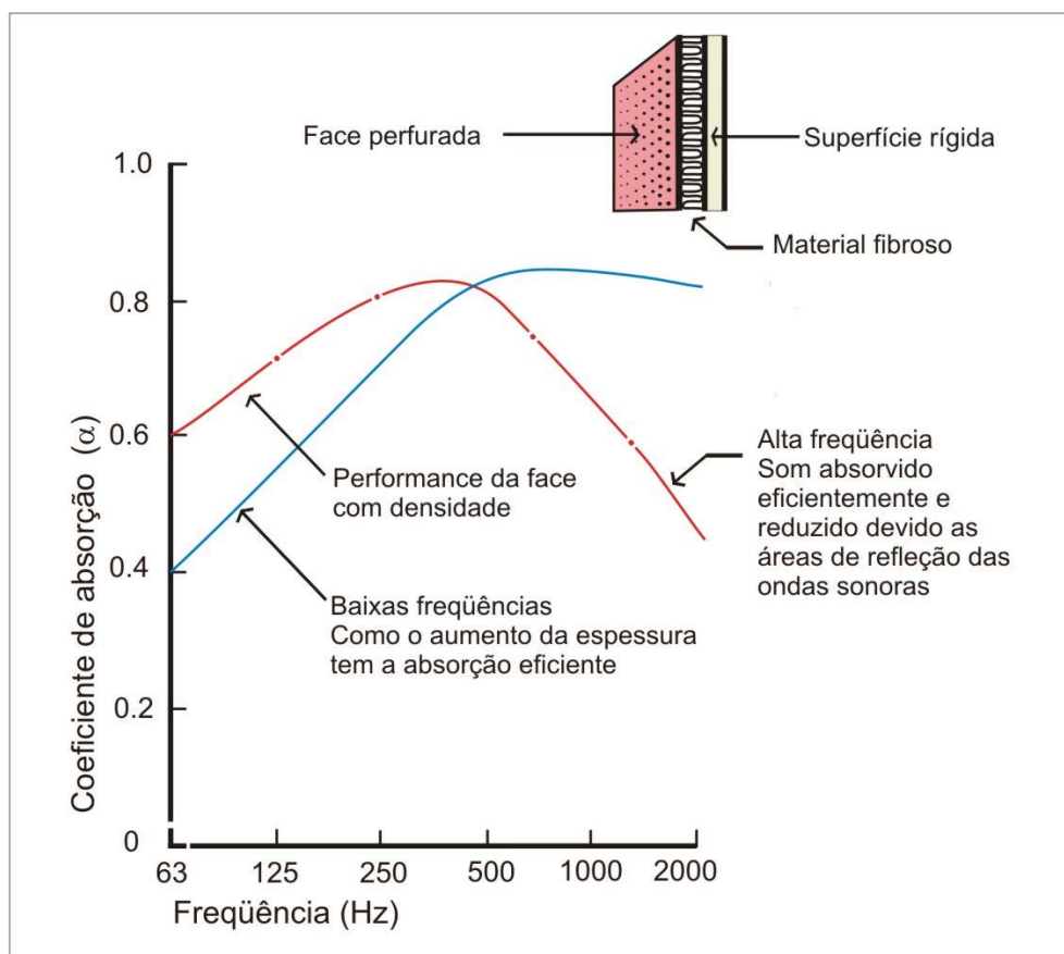
Figura 15 – Comportamento do som no ressonador com material absorvente
