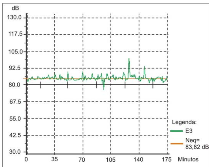
Figura 29 – Variação dos NPS para o operador no posto de trabalho E3 durante 4 horas
