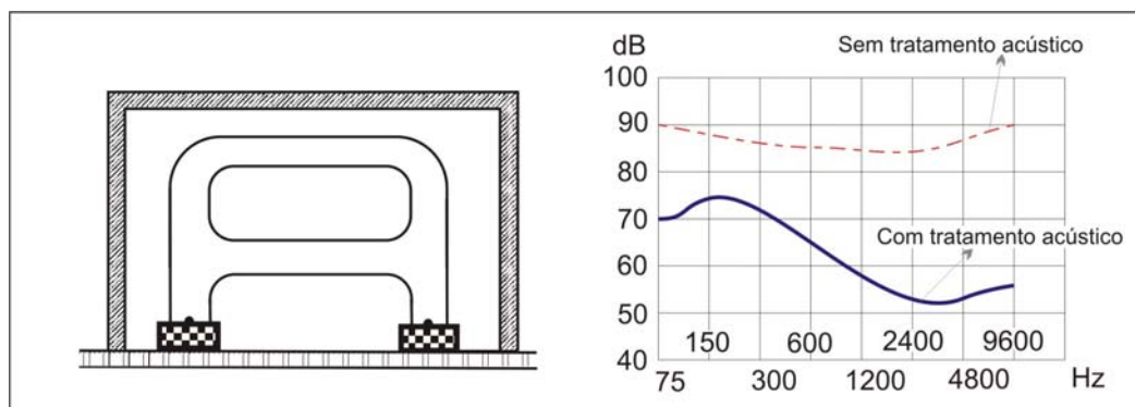
Figura 6 – Instalação de blindagem rígida e amortecedor na máquina
