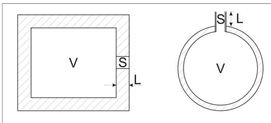
Figura 14 – Ressonadores de Helmholtz simples
