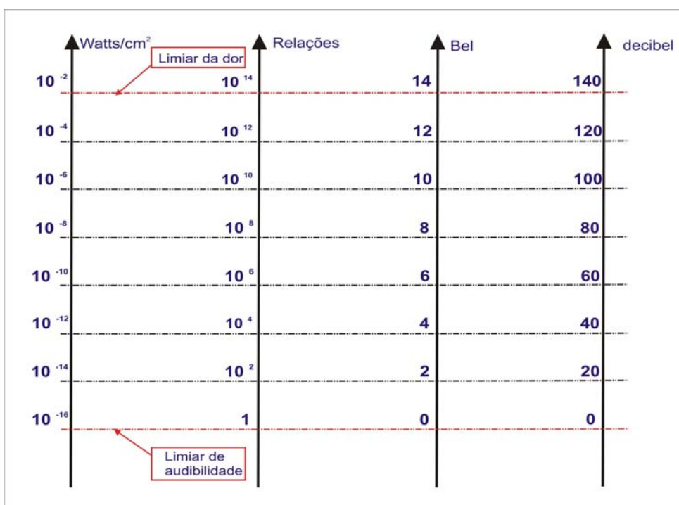
Figura 4 – Esquema da formação da escala em decibéis
