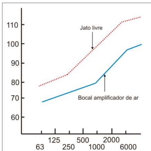
Figura 9 – Gráfico de atenuação do ruído com o uso do bocal amplificador de ar
