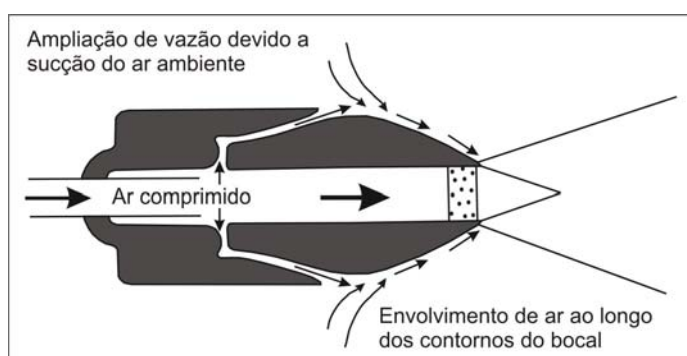
Figura 8 – Bocal amplificador de ar
