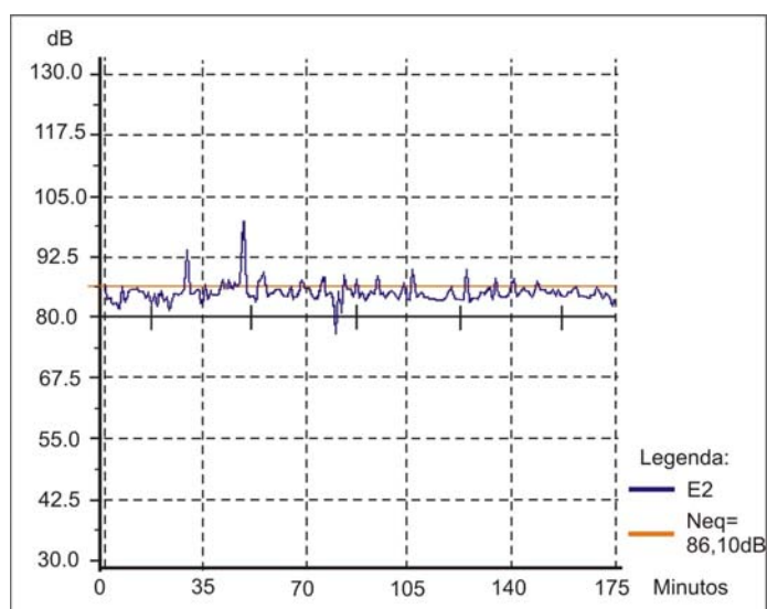
Figura 28 – Variação dos NPS para o operador no posto de trabalho E2 durante 4 horas
