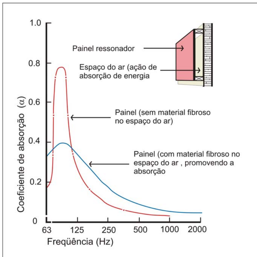
Figura 16 – Comportamento do som no ressonador com espaçamento do ar
