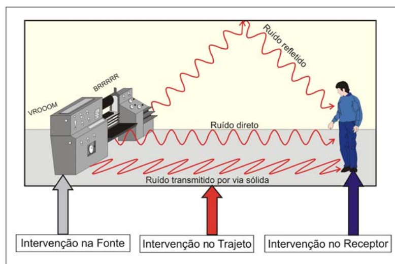
Figura 10 – Esquemática do ruído refletido, direto e transmitido por via sólida.
