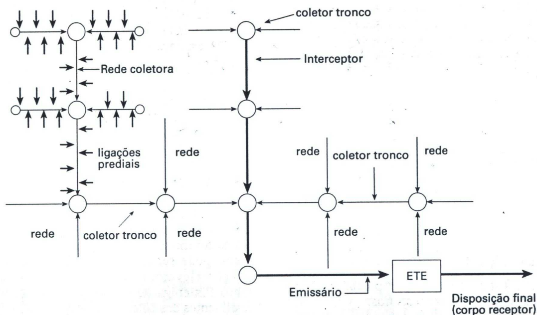
Figura 2.2 – Esquema de sistema de coleta, transporte, tratamento e disposição final de esgoto sanitário.
