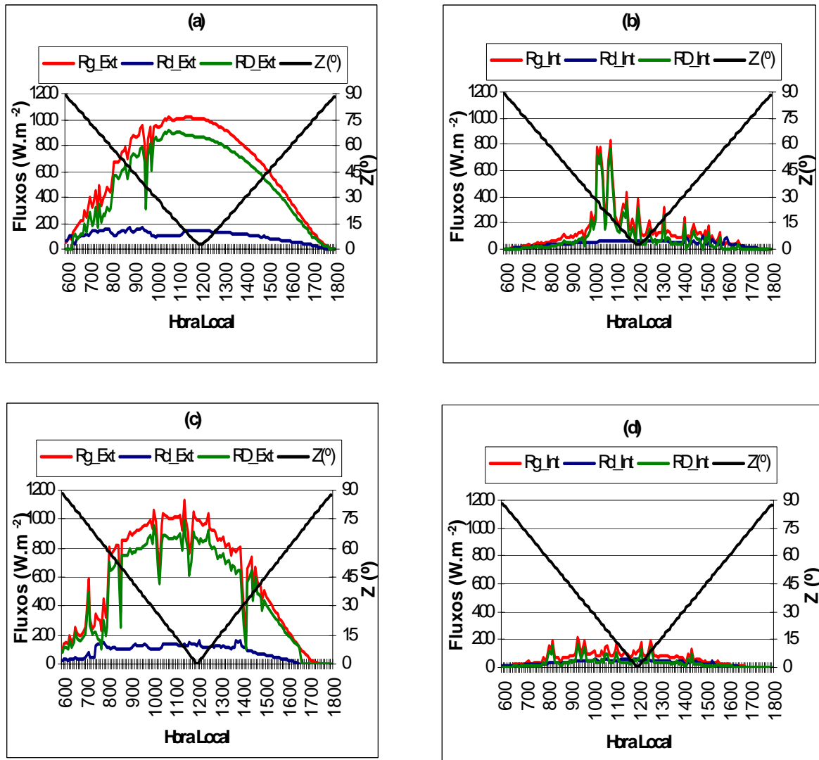
Figura 25 - Comportamento da Radiação Global Externa ( Rg\_Ext ) e suas componentes Rd\_Ext e RD\_Ext ( W.m^{-2} ) em função do Ângulo Zenital ( Z ) ( ^{\circ} ), (a) e (b) dia 06/03, (c) e (d) dia 14/10, sobre a área de estudo.
