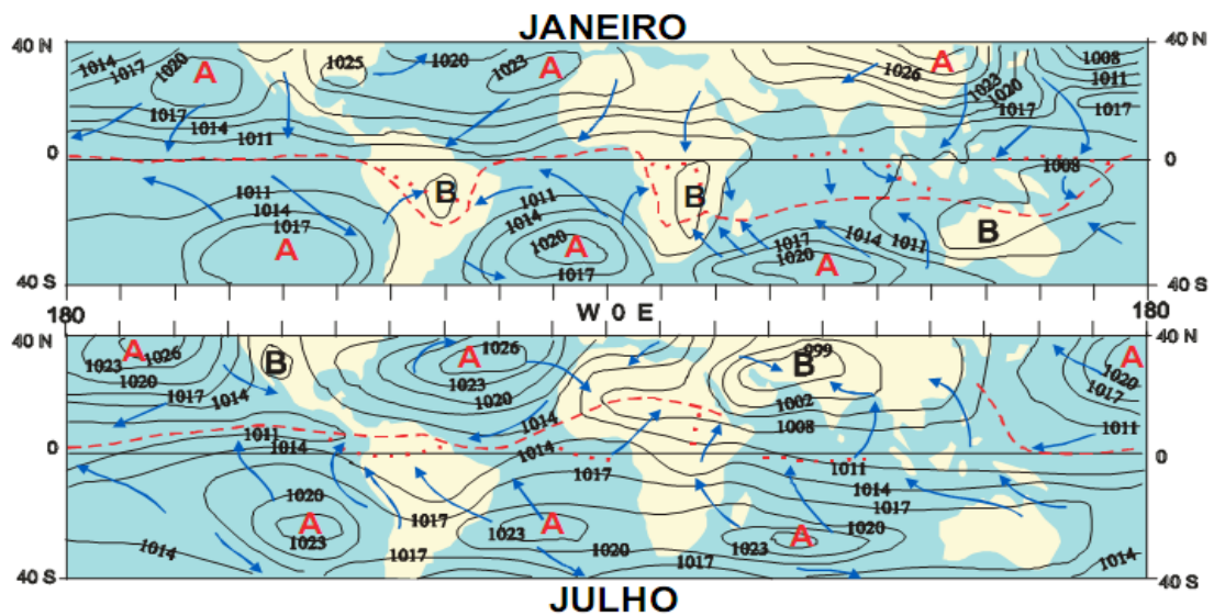
Figura 6: Distribuição média temporal da pressão (hPa) ao nível médio do mar. São indicados os centros de alta (A) e baixa (B) pressão bem como os ventos dominantes à superfície (setas).
